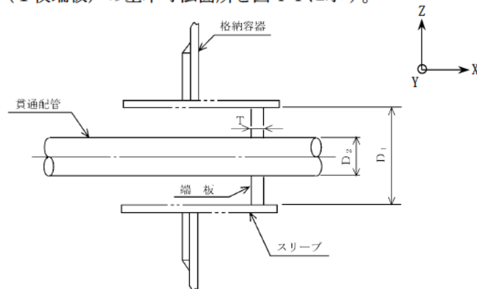
図 4-1 固定式継手（1枚端版）の基本寸法箇所
