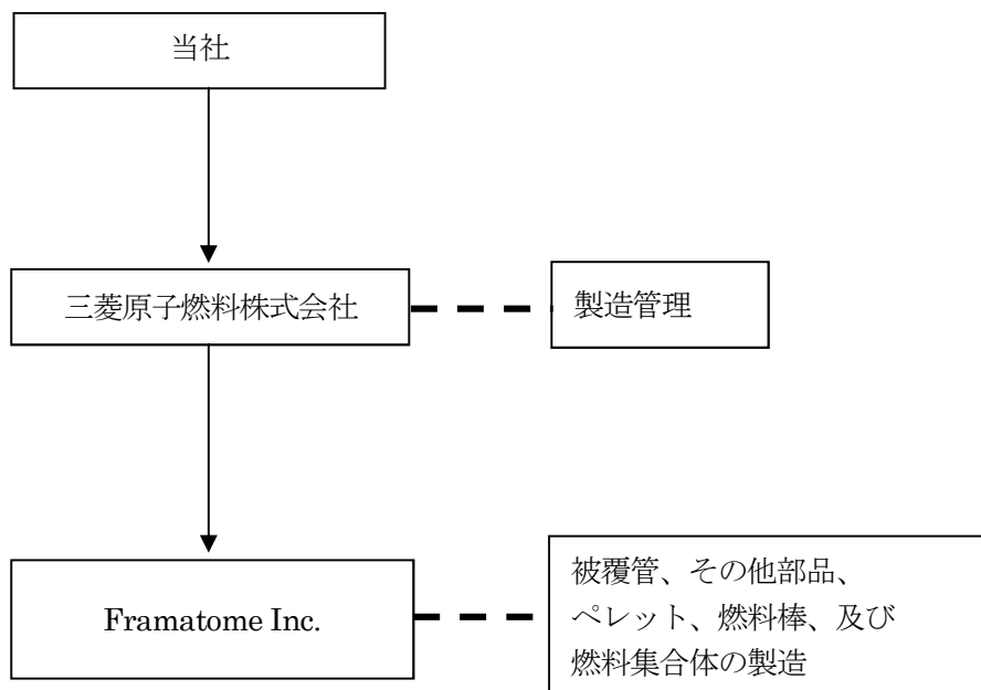
図－２ 輸入ウラン燃料体の製造体制
