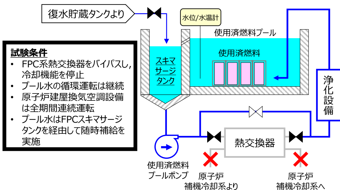
敦賀1号炉 FPC系冷却機能停止試験時の系統構成概要
