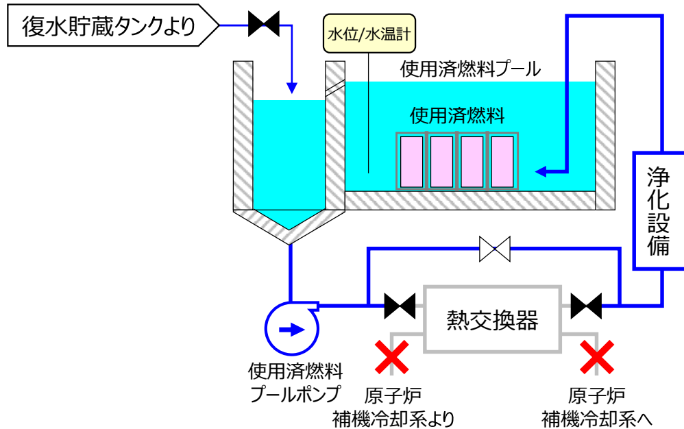
敦賀1号炉 SFP冷却機能停止試験時の系統構成概要
