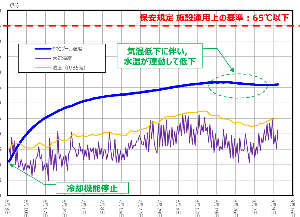
敦賀1号炉 SFP冷却機能停止試験結果
