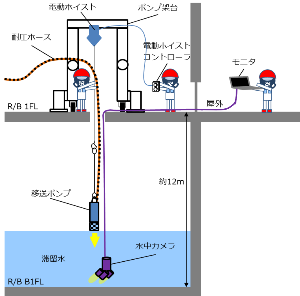
地上階でのポンプ設置作業概要図
