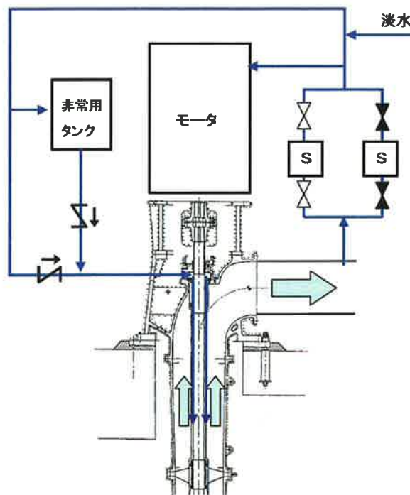
図2 海水ポンプ軸受潤滑水系統概略図
