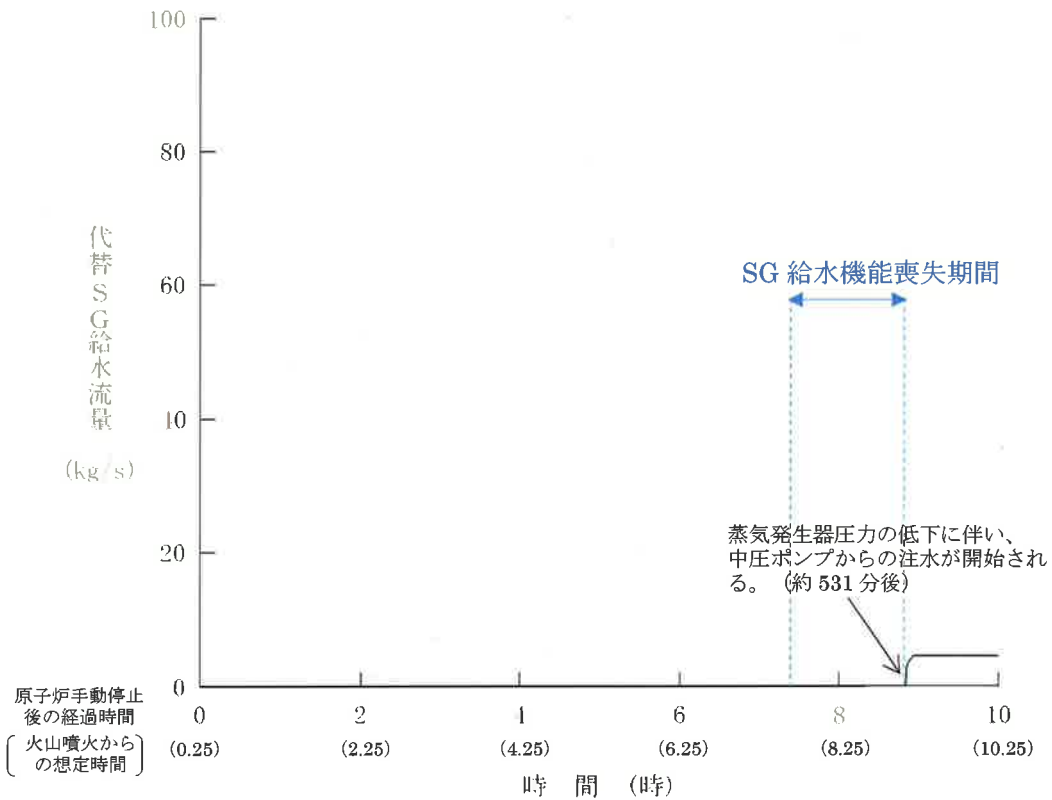
第5図 蒸気発生器2次側への注水流量
