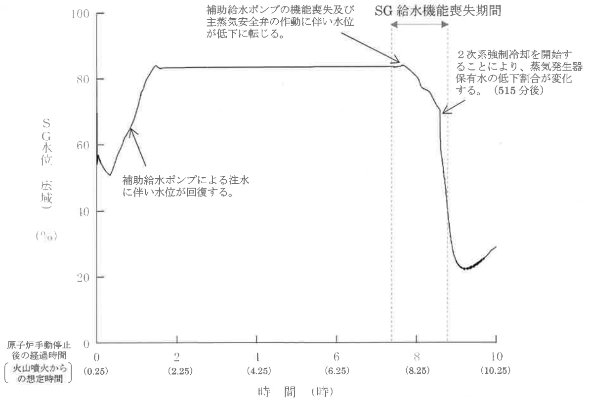
第3図 蒸気発生器水位 (広域)
