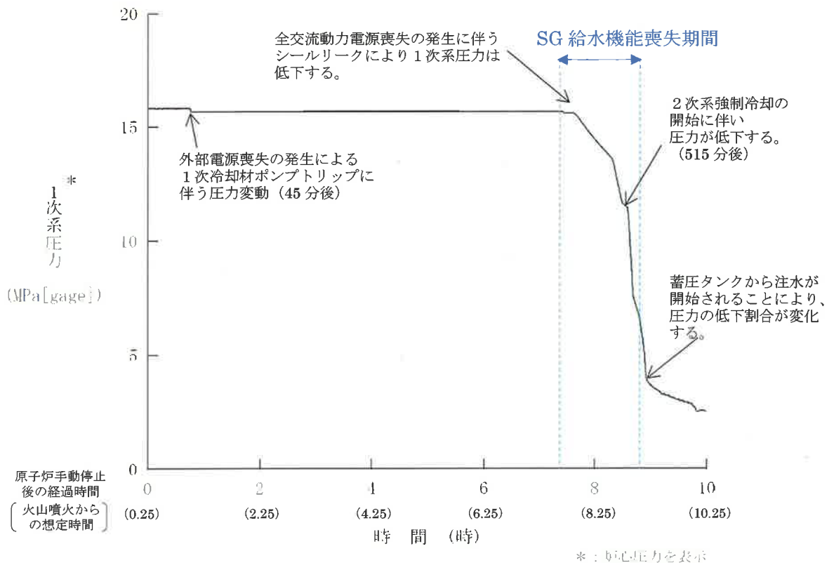
第7図 1次系圧力
