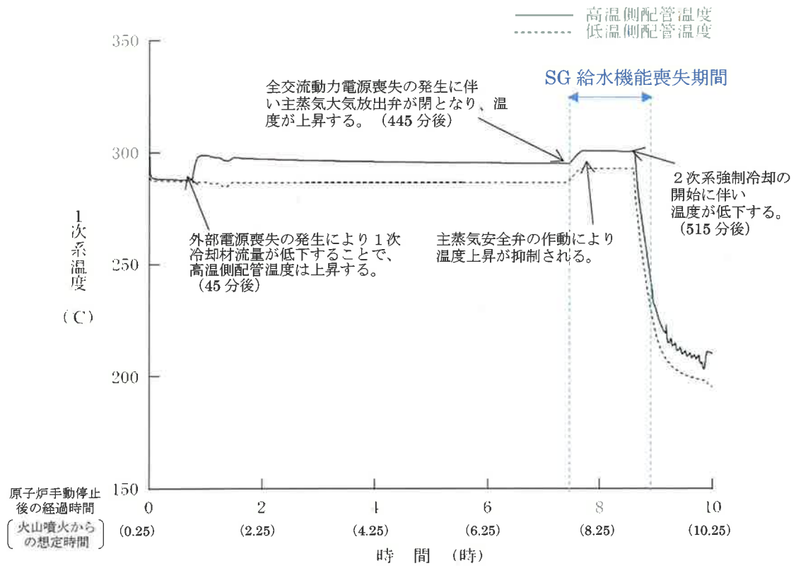
第6図 1次系温度 (高温側、低温側)
