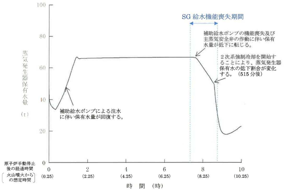
第4図 蒸気発生器保有水量 (液相)
