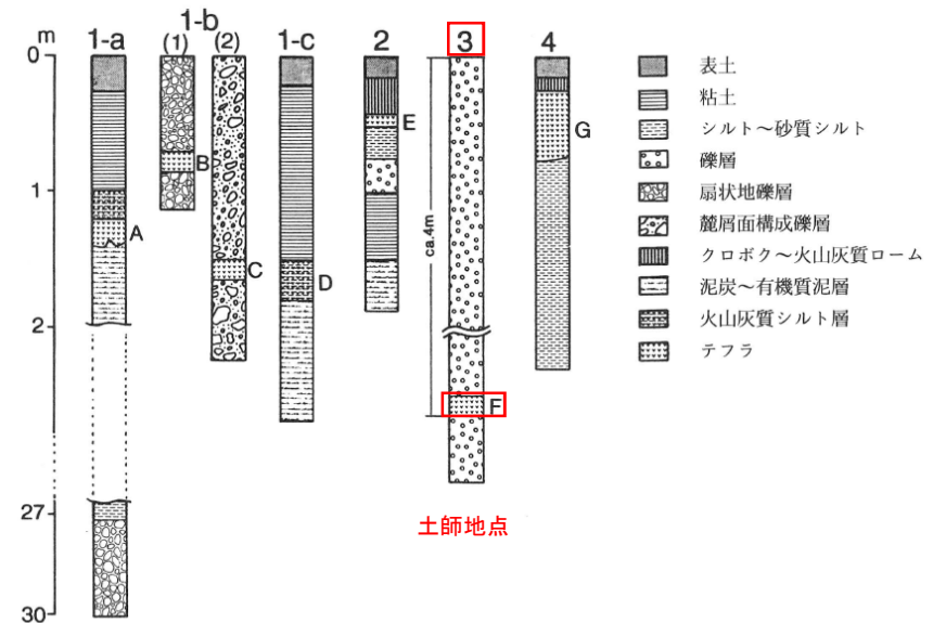
第3図 柱状図
