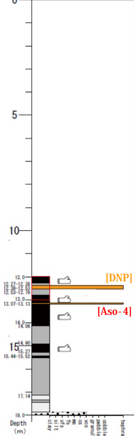
孔名: S-3B(EL=335.298m)
