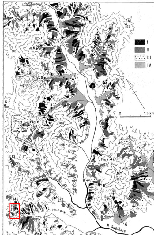
第3図 杉原川流域の山麓斜面の分布および露頭位置 I: I面 II: II面 III: III面 IV: IV面 MY: 妙見山 S: 千ヶ峰 SA: 樺ヶ峰 1~15: 露頭位置および図番号, A~A', B~B', C~C': 第11図の観断面形状位置
