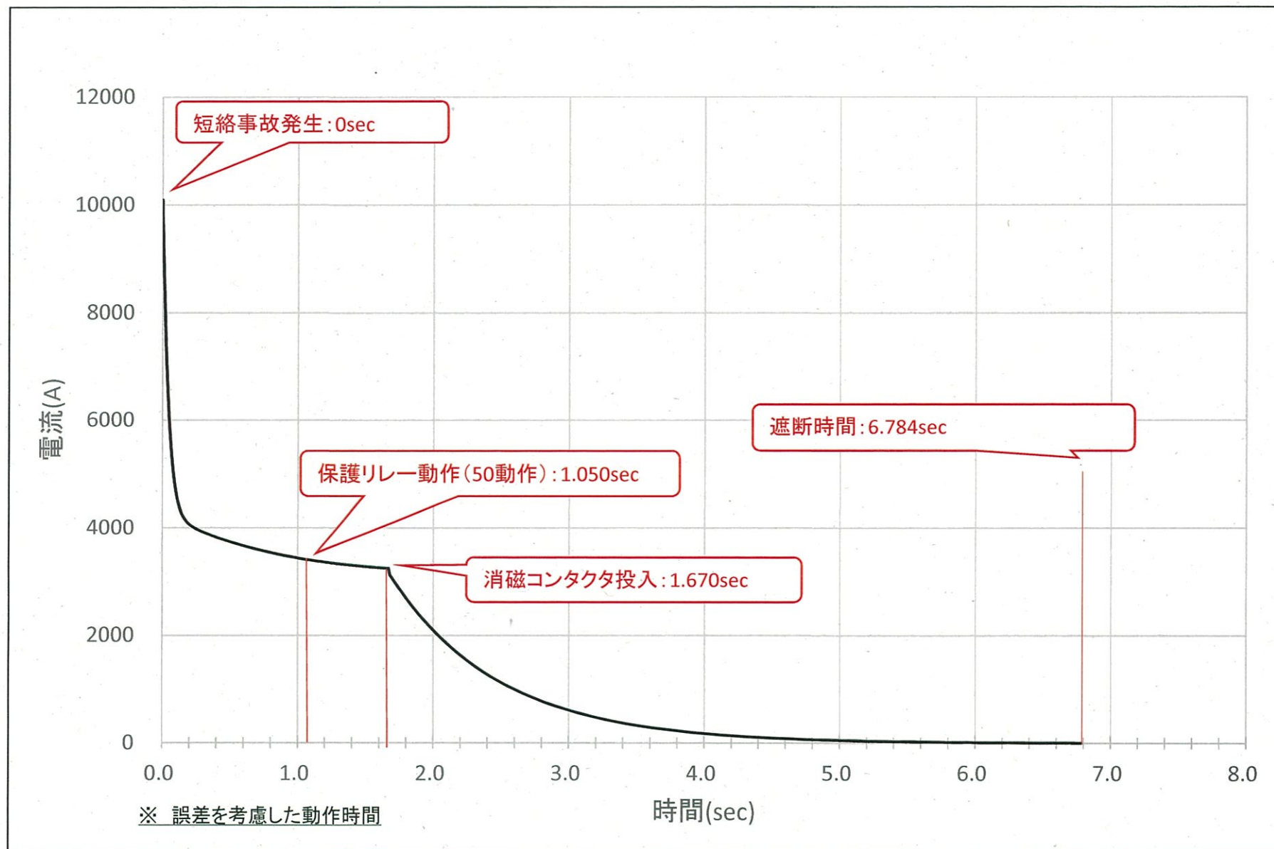
非常用ディーゼル発電機受電遮断器にHEAFが発生した場合の アーク電流の減衰(伊方3号機(A系))
