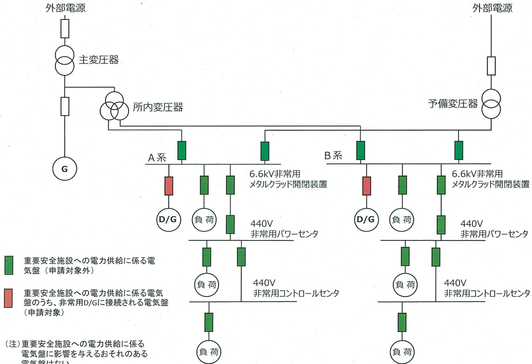
図1 伊方3号機 所内電気系統 (概要図)
