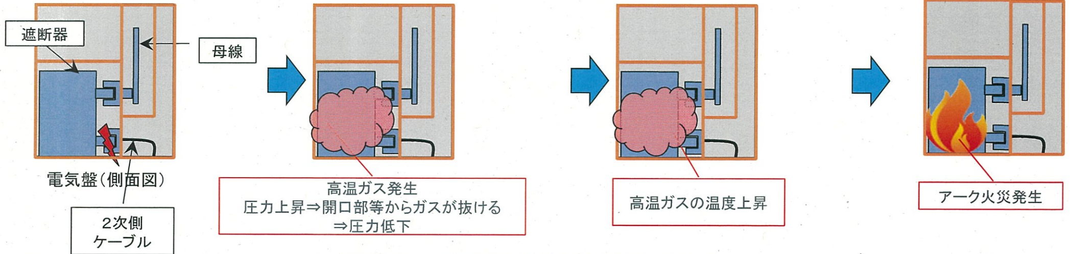
(1)アーク放電発生
