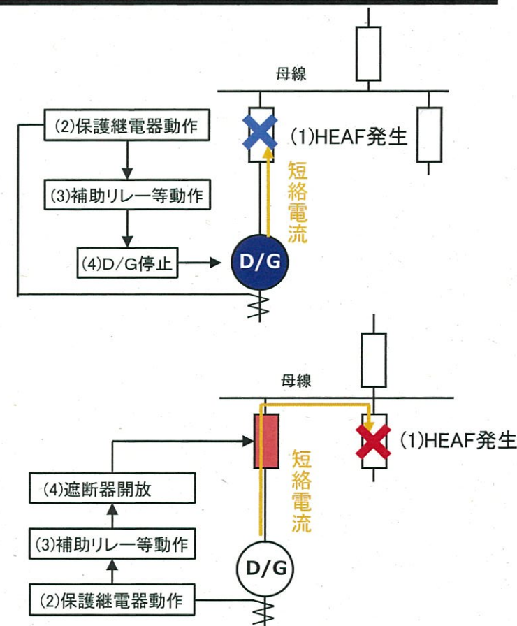
図2 電流供給停止までの流れ
