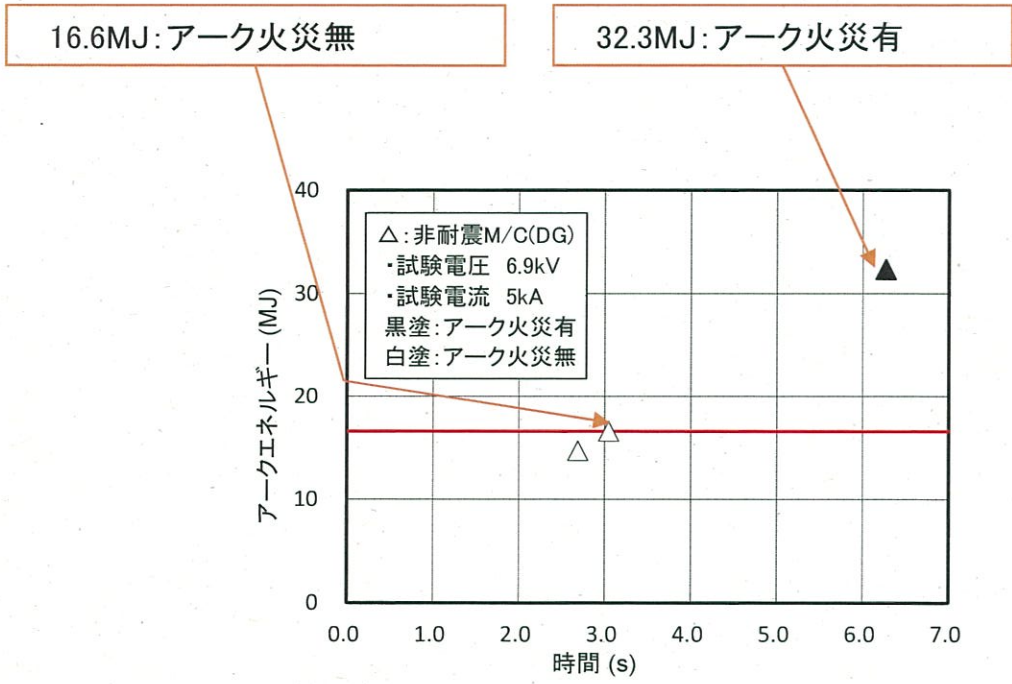
試験結果(アーク火災発生状況)
