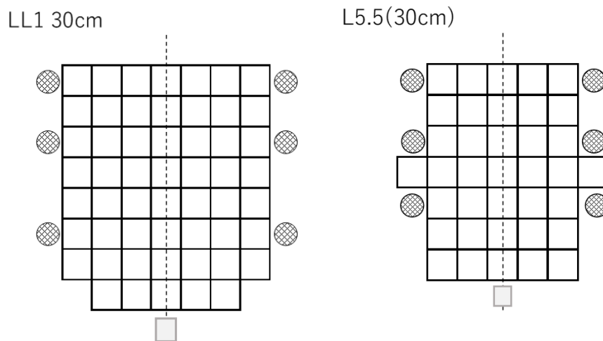
図 A-12 固体減速炉心の配置図（左：LL1（高さ約30cm）、右：L5.5（高さ約30cm））
