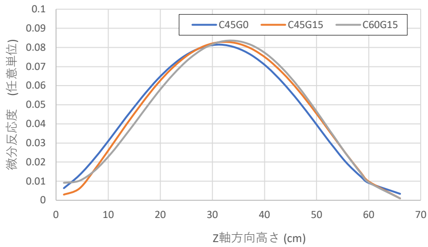
図 A-11 2分割炉心の制御棒微分反応度曲線（曲線の積分値が1となるように規格化） （C45G0(4列)炉心、C45G15(4列)炉心、C60G15(4列)炉心）
