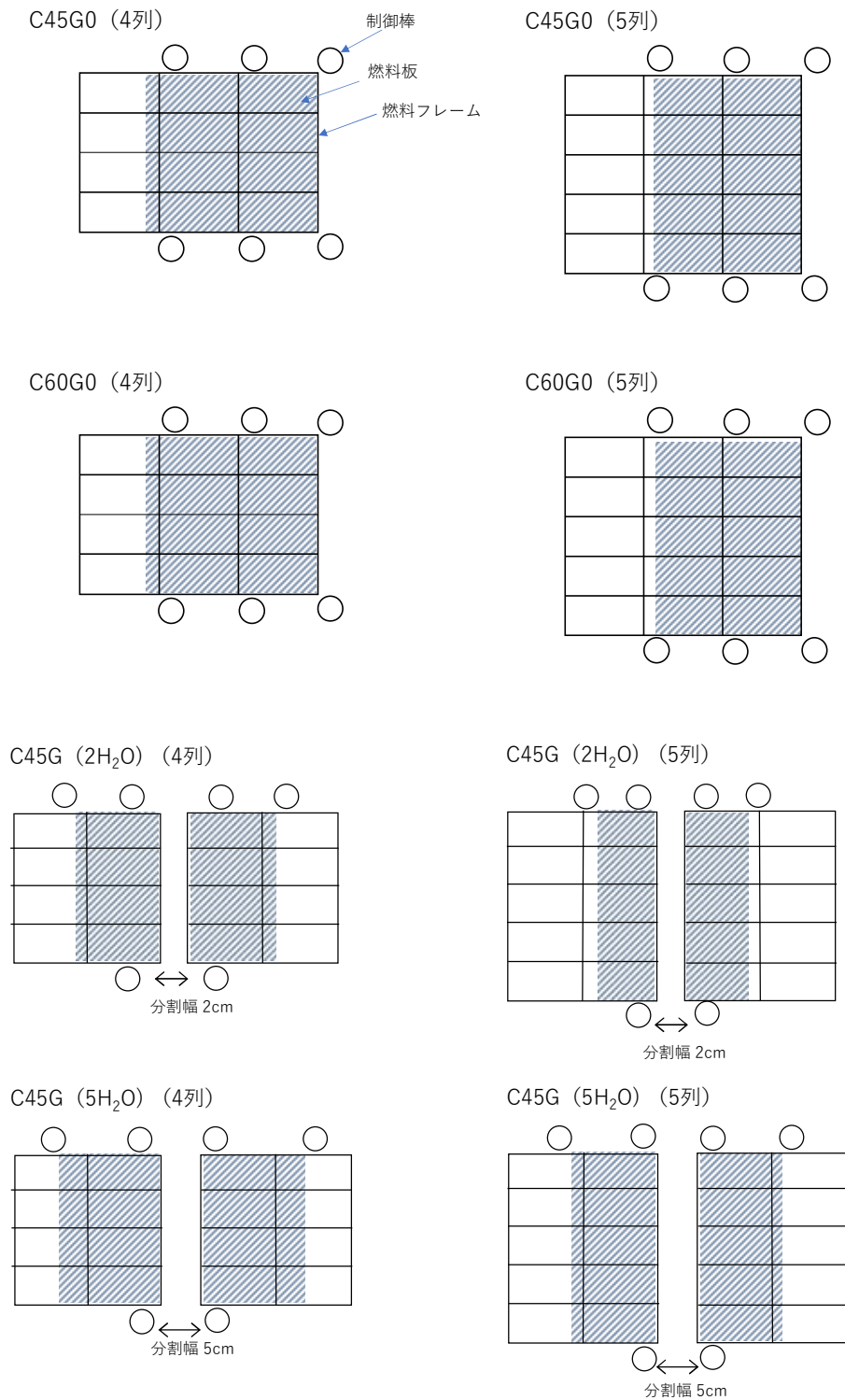
図 14 軽水減速炉心の炉心配置図 (2)
