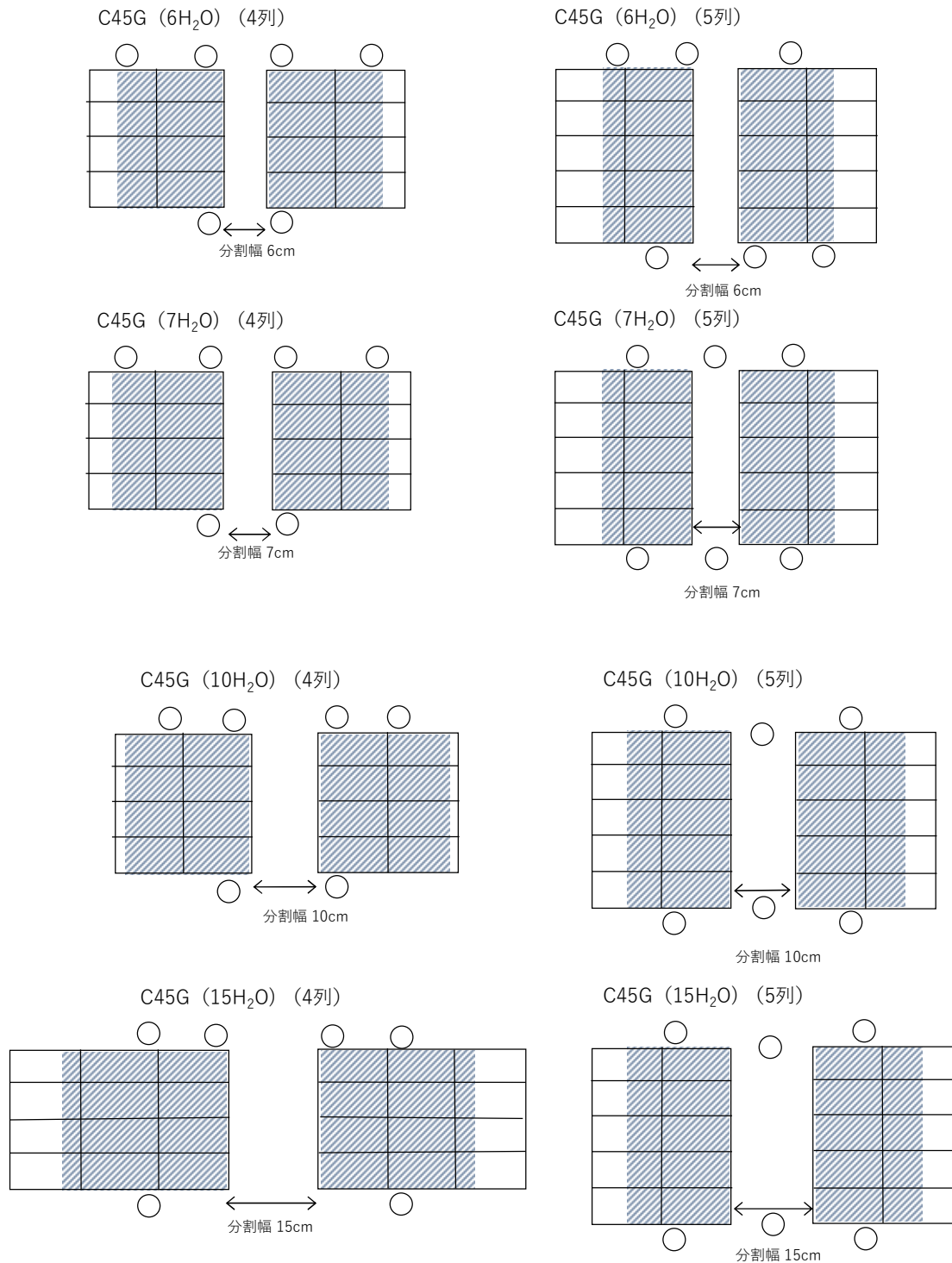
図 14-2 軽水減速炉心の炉心配置図 (3)
