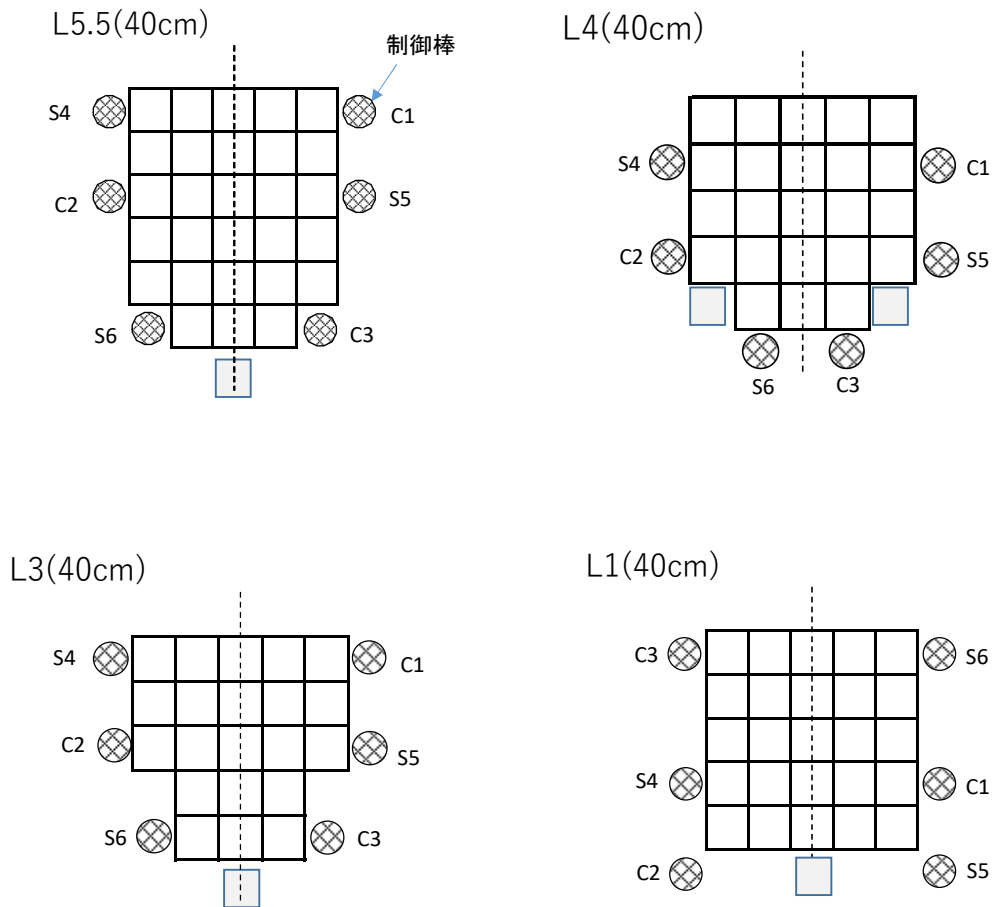
図 A-2 MCNP による解析炉心
