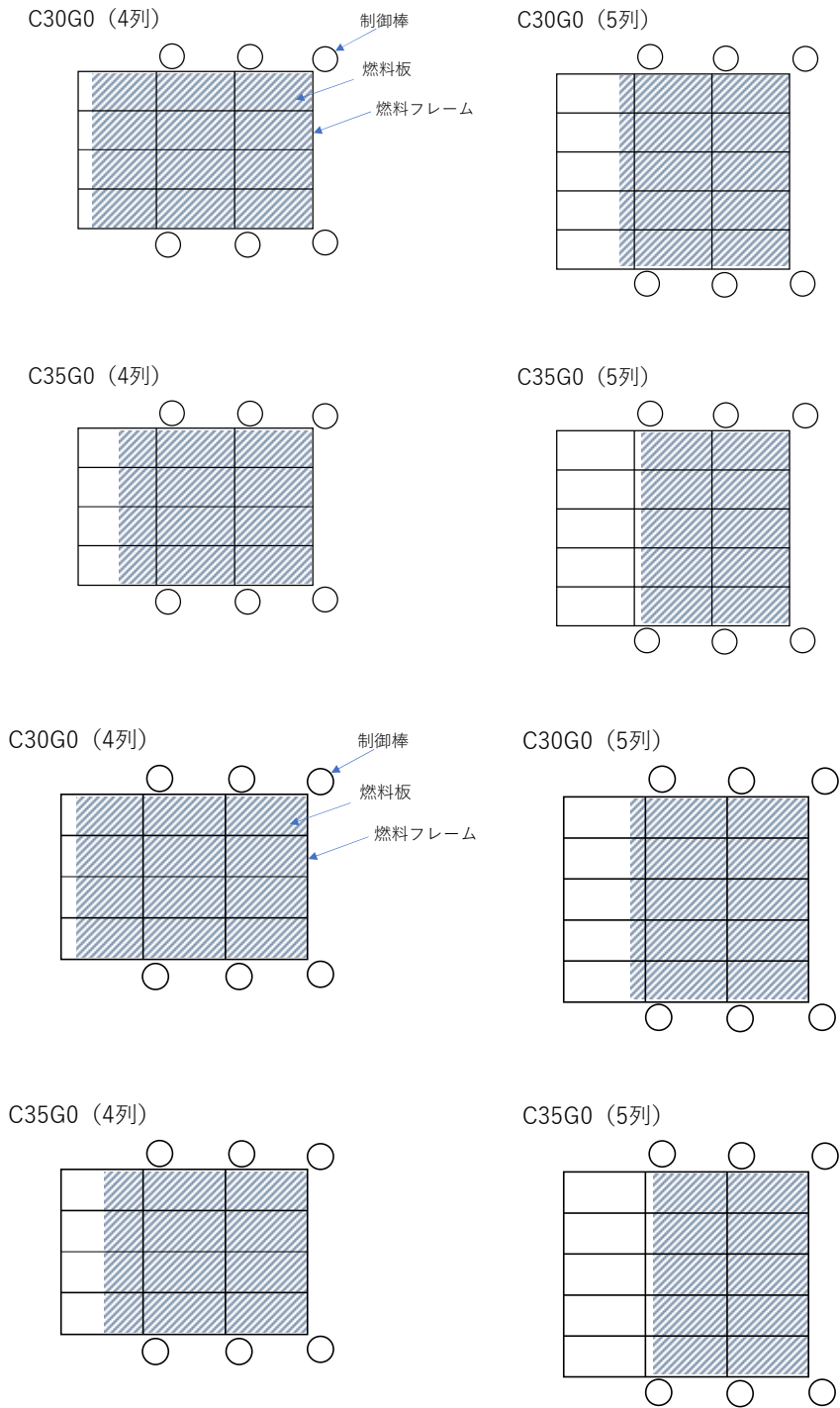
図 13 軽水減速炉心の炉心配置図 (1)
