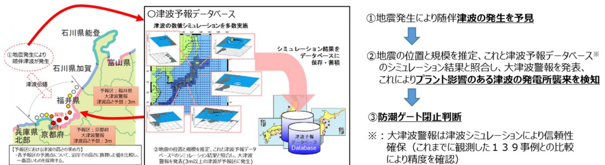
図31 既許可の基準津波1における対応
