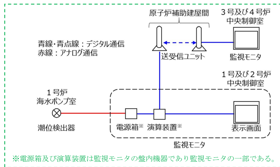
図23 1号炉海水ポンプ室に設置する潮位計(防護用)のシステム構成図
