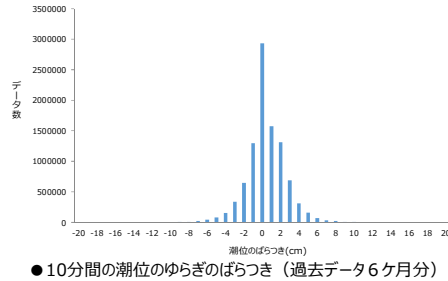
図30 潮位計（監視用）の平常時における10分間の潮位のゆらぎ
