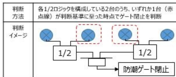
図24-2 1 out of 2 twiceの判断方法とイメージ
