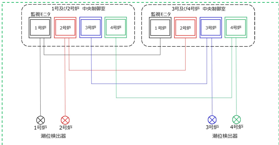
図 3 8 潮位計（防護用）のシステム構成イメージ
