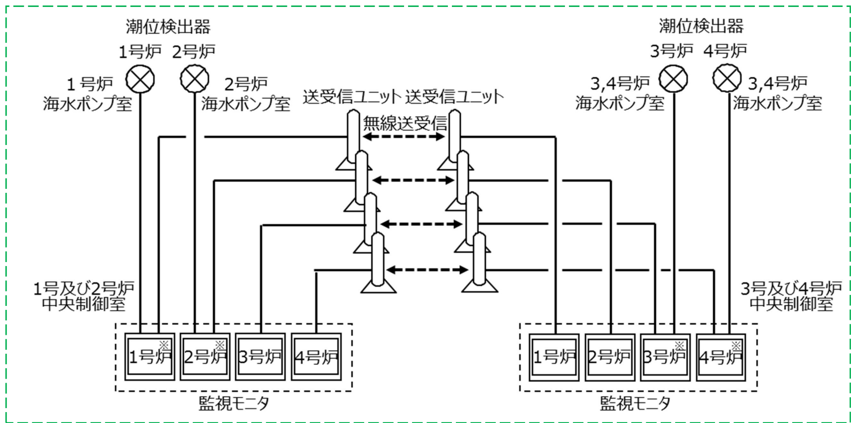
図4 潮位計（防護用）のシステム構成
