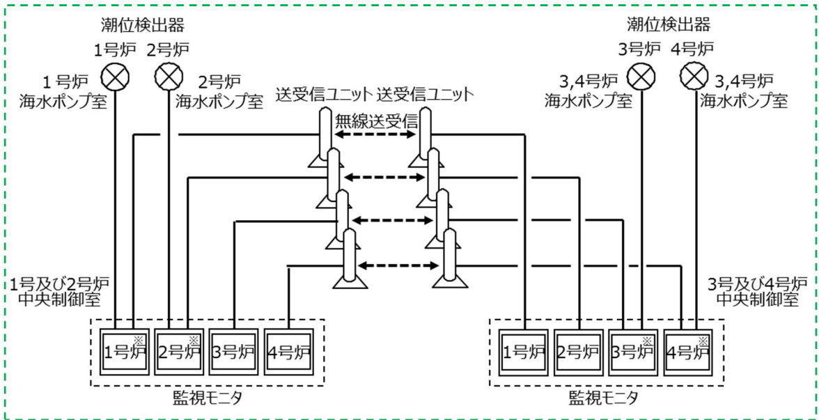
図 3 4 潮位計（防護用）のシステム構成
