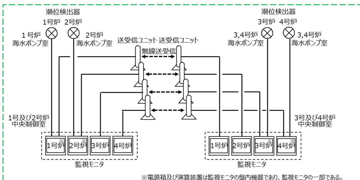
図27 潮位計（防護用）のシステム構成図
