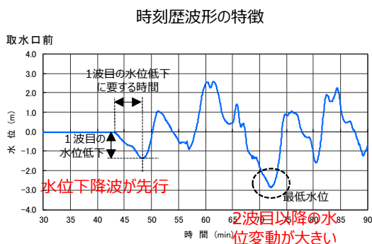
図1 隠岐トラフ海底地すべりを波源とする津波の波形の特徴
