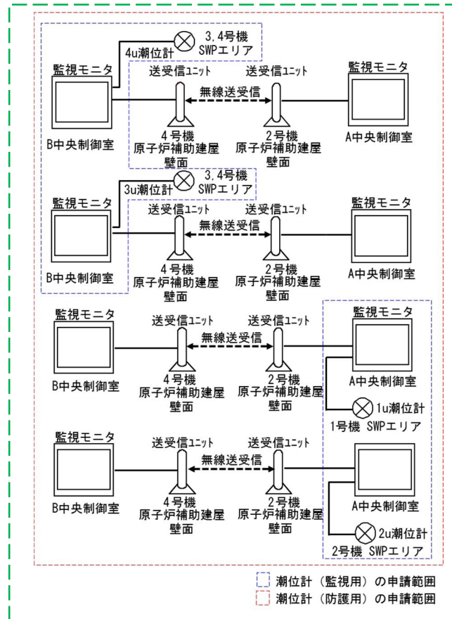
図3 1 既許可の潮位計（監視用）の設備構成
