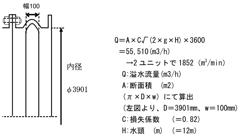
図-2-4-27 循環水ポンプ出口配管断面
