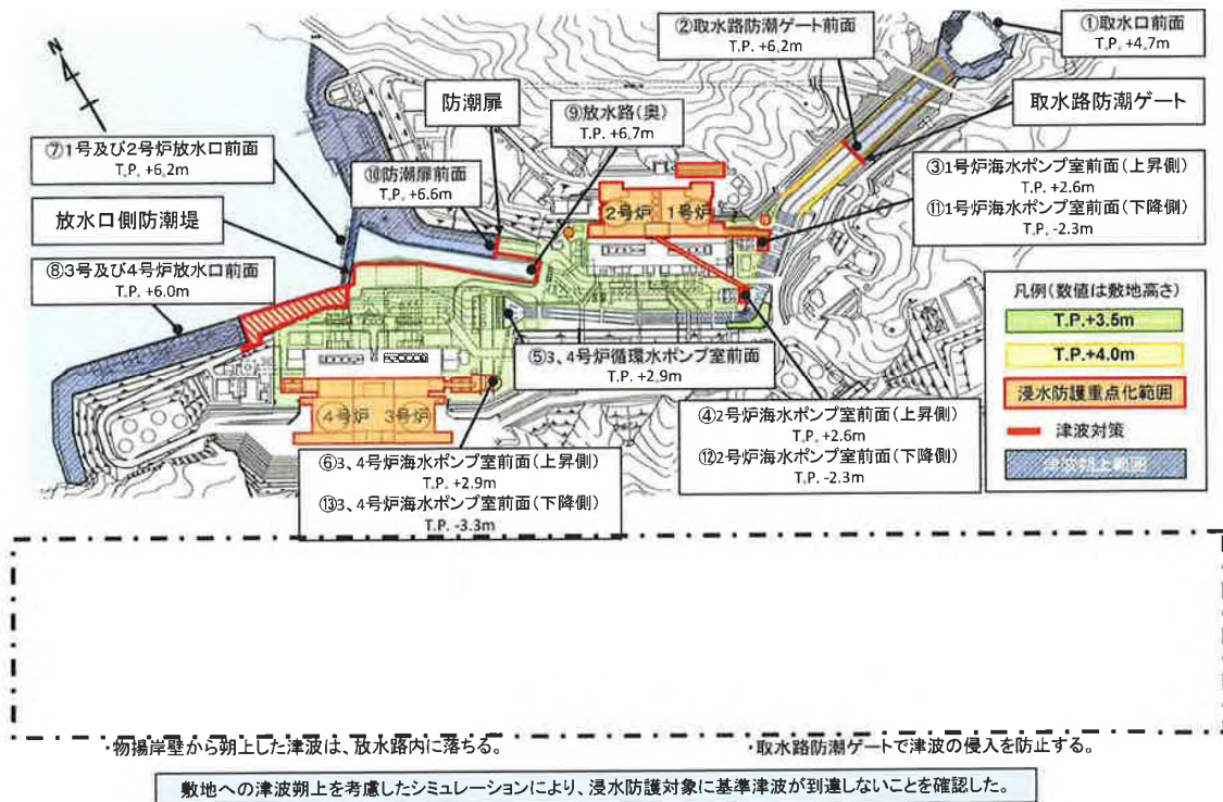
図-1-6-1 高浜発電所における入力津波評価地点
