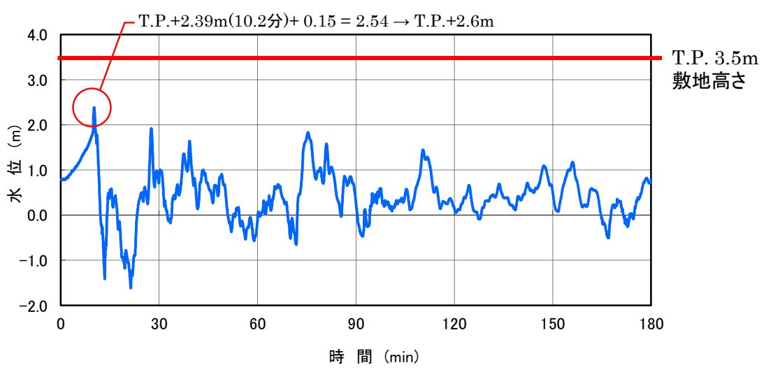
図-2-2-21 2号炉海水ポンプ室 津波波形
