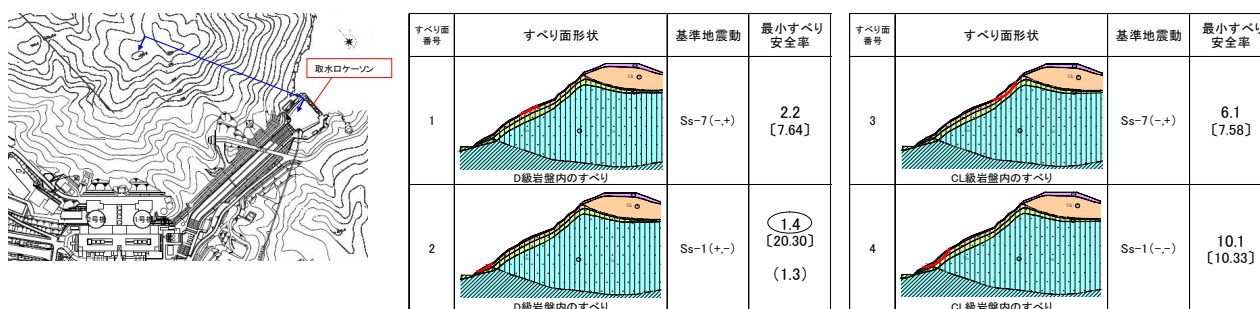
図-1-3-4 取水ロケソン周辺斜面の安定性評価結果
