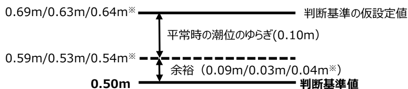
図-1-4-9 取水路防潮ゲートの閉止判断基準の概念図
