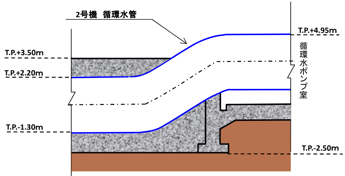
図-2-2-20 2号機循環水管埋設部 断面図④
