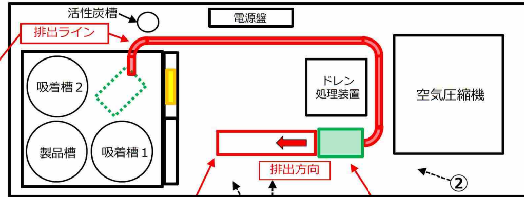
コンテナ内の機器配置 (平面図)
