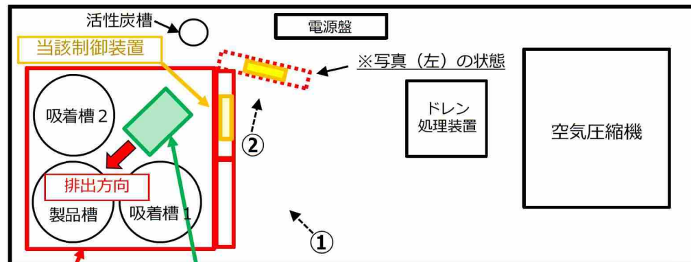
コンテナ内の機器配置 (平面図)
