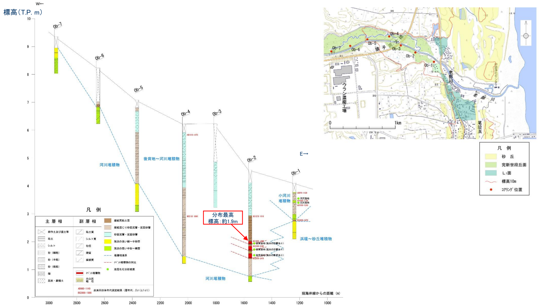
尾駸老部川地点における調査結果(地質断面図)
