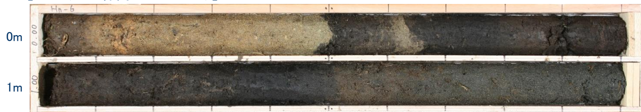
【Hn-6(孔口標高:T.P.+3.80m)】
