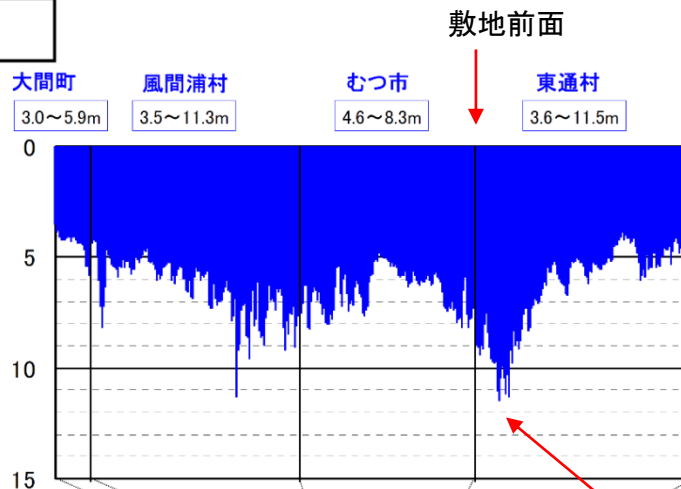
海岸線上での津波の水位図(青森県下北半島北西部)
