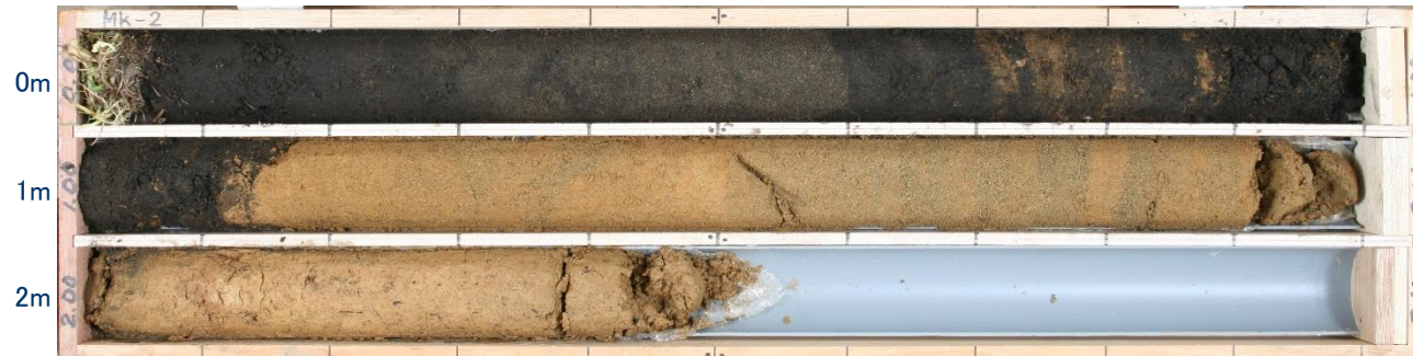
【Mk-2(孔口標高:T.P.+9.04m)】
