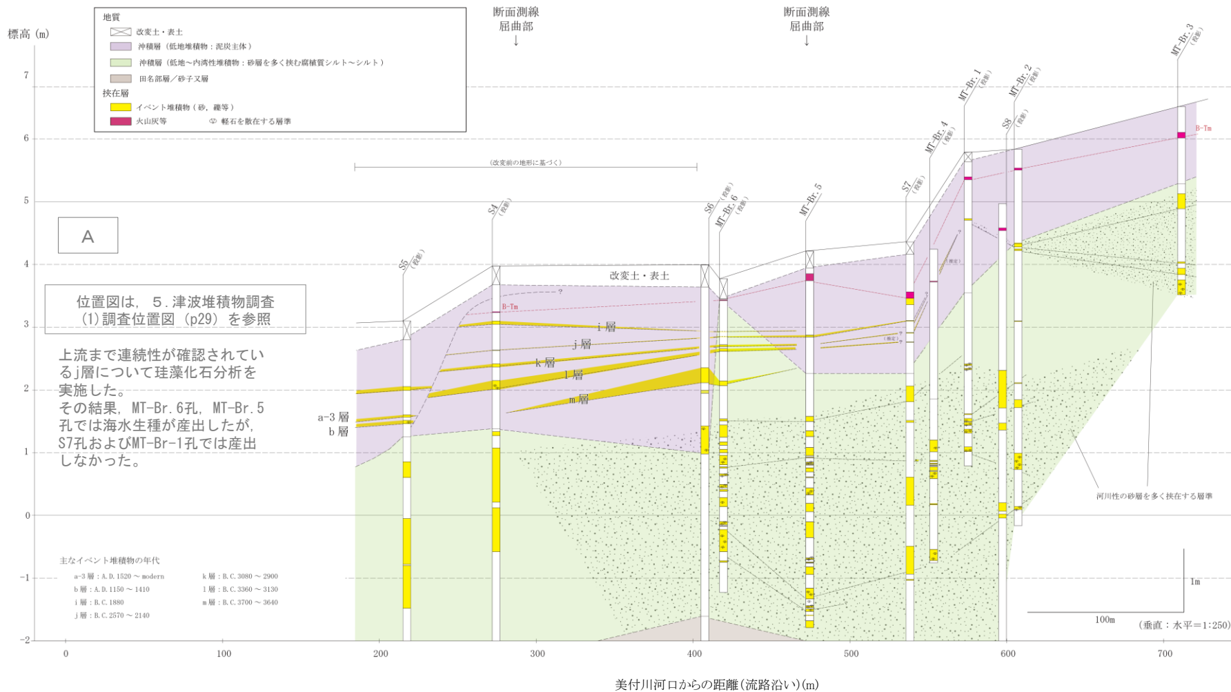
関根地点における調査結果(地質断面図)
