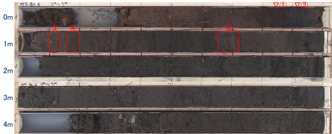
【MT-Br.6(孔口標高:T.P.+3.77m)】
