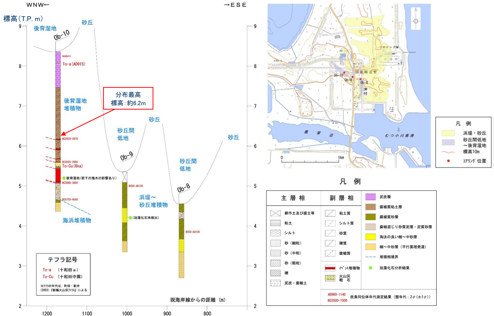
尾駈発茶沢地点における調査結果(地質断面図)
