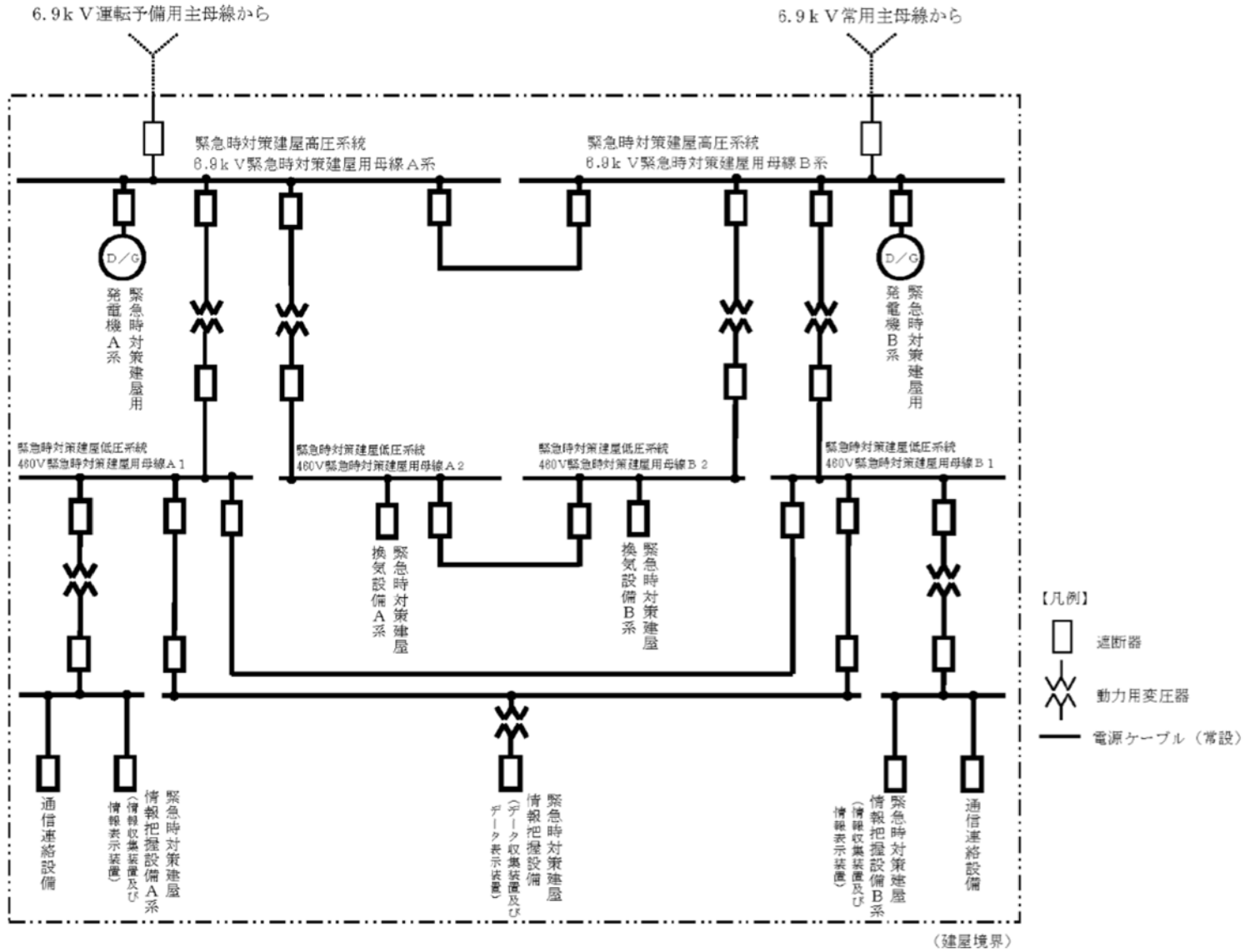
第 34. 8 図 緊急時対策建屋電源設備の系統概要図
