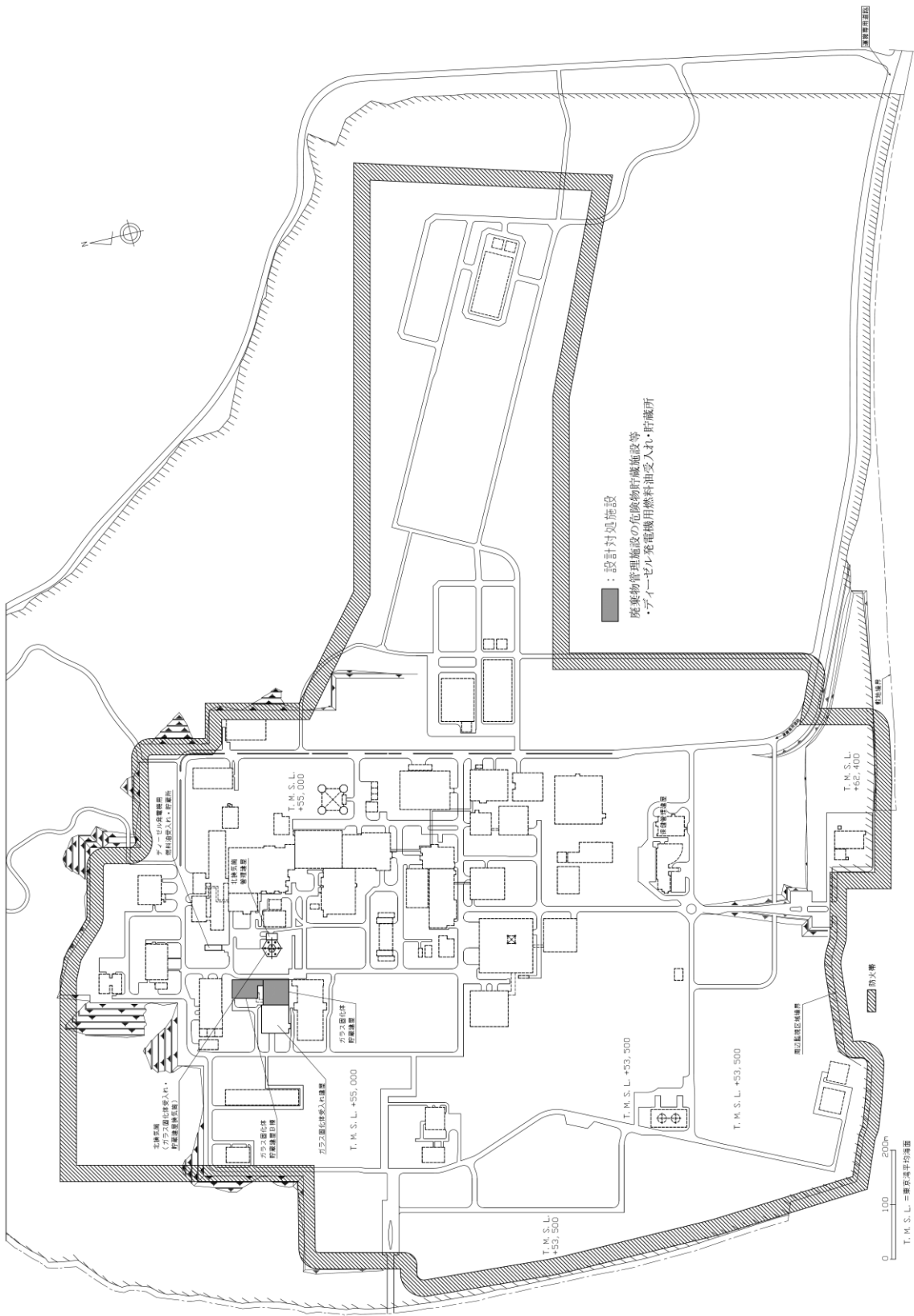
第8.5図 (外部火災) 防火帯, 設計対処施設等の配置図
