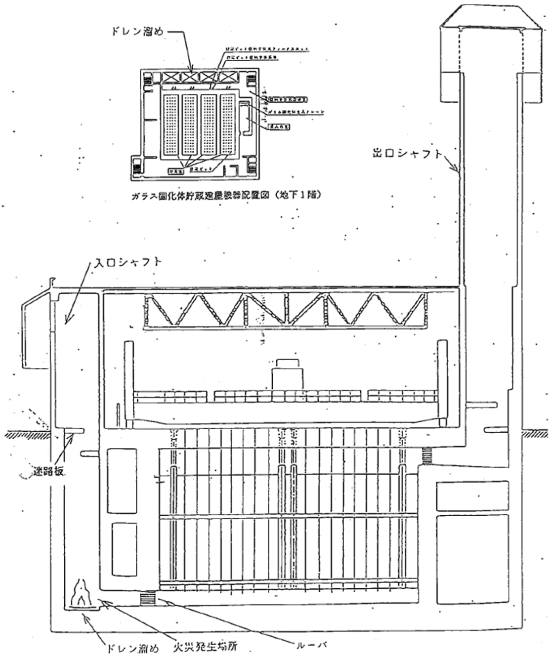
第1図 入口シャフト下部構造概念図
