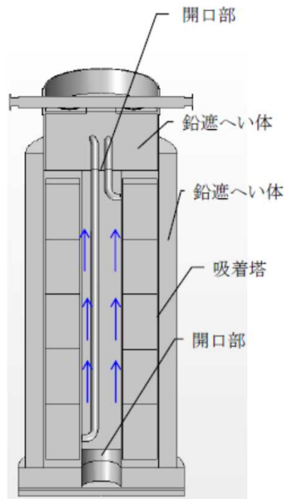
解析モデル
