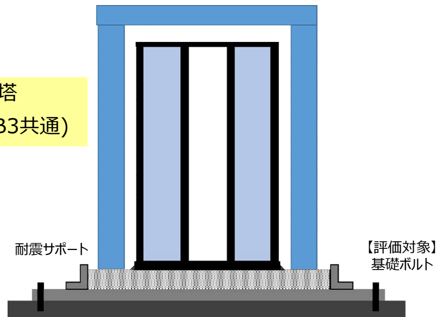
SARRY II 吸着塔 B 型
