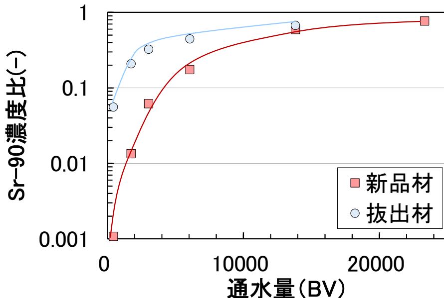
抜出材の試験結果
