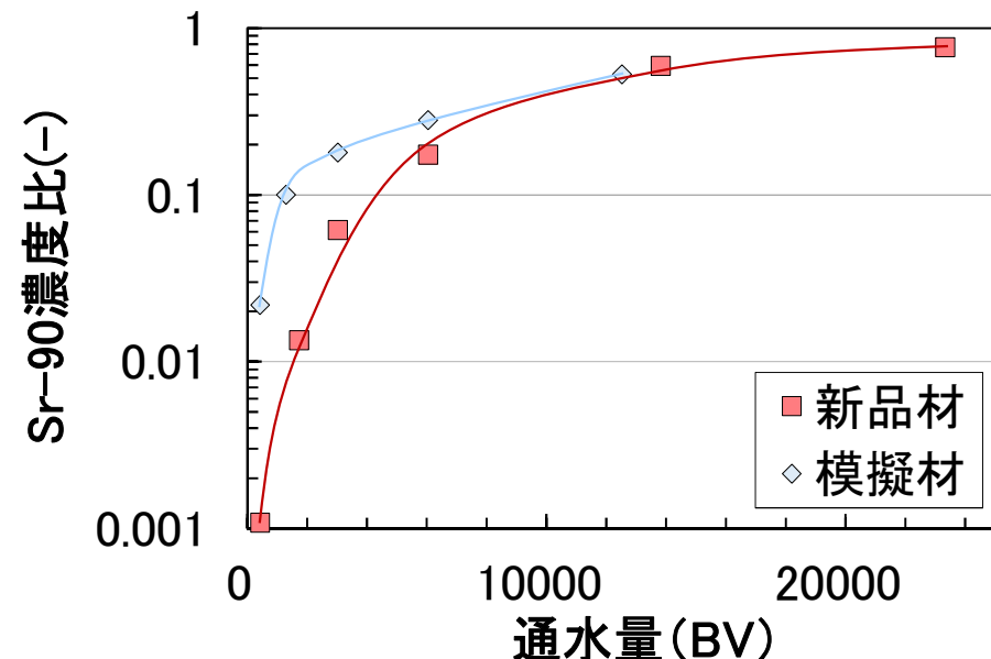
模擬材の試験結果
