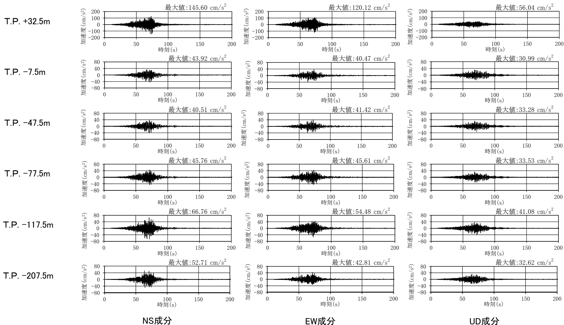
加速度時刻歴波形
