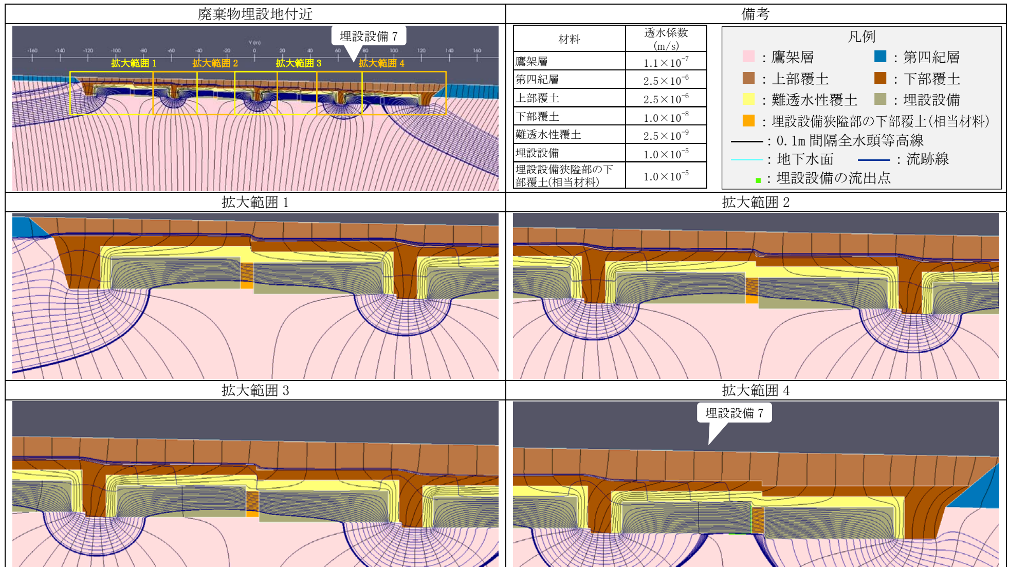
第1図 2次元地下水浸透流解析結果(確からしい設定 1,000年後) (8/9) <埋設設備7の流出点を通る流跡線>
