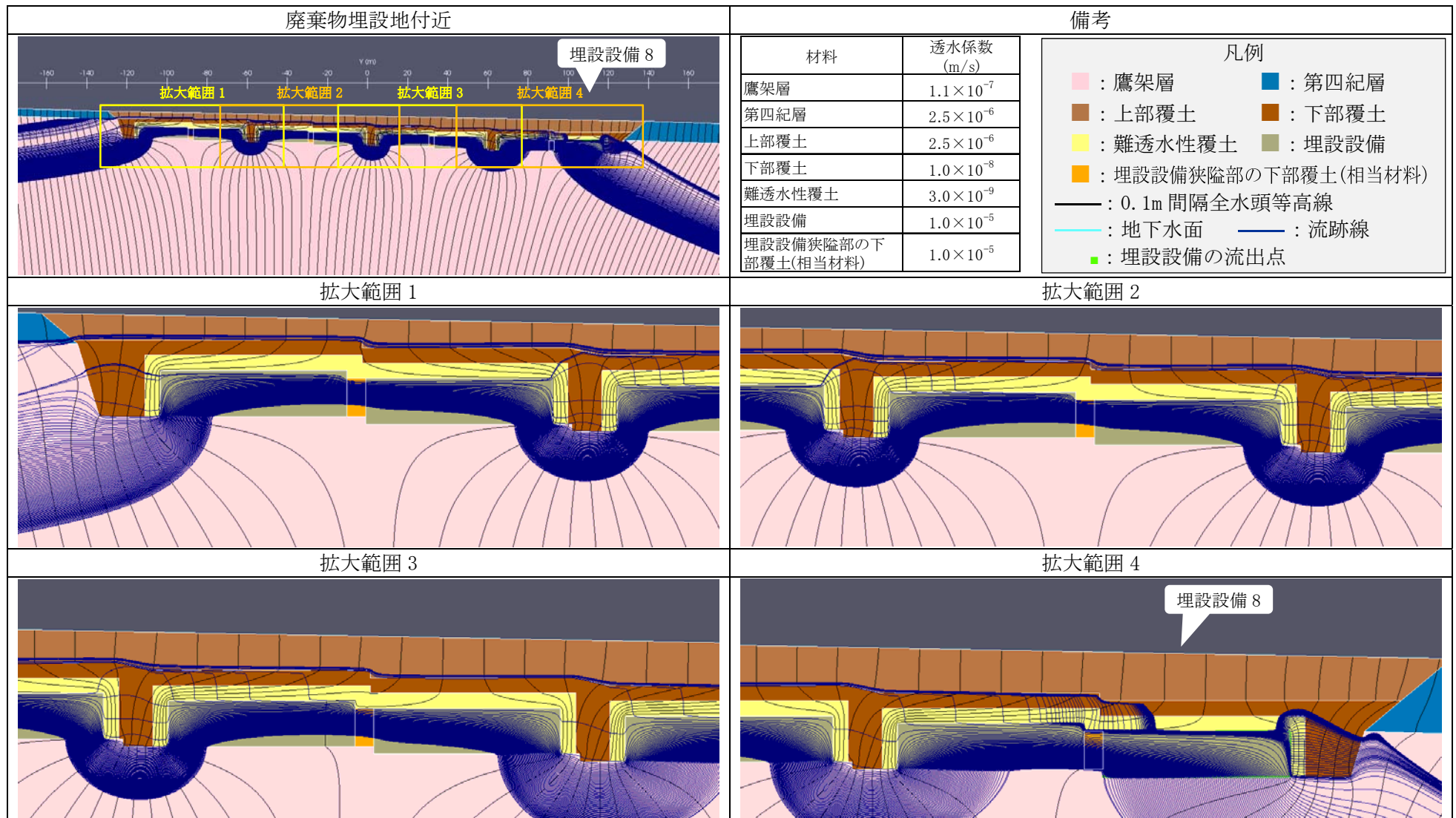
第2図 2次元地下水浸透流解析結果(厳しい設定 1,000年後) (9/9) <埋設設備8の流出点を通る流跡線>
