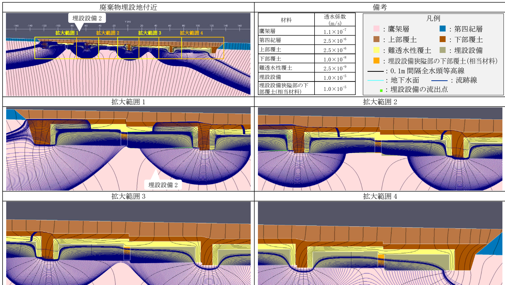
第1図 2次元地下水浸透流解析結果(確からしい設定 1,000年後) (3/9) <埋設設備2の流出点を通る流跡線>
