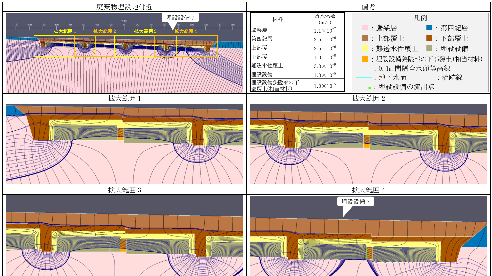
第2図 2次元地下水浸透流解析結果(厳しい設定 1,000年後) (8/9) <埋設設備7の流出点を通る流跡線>
