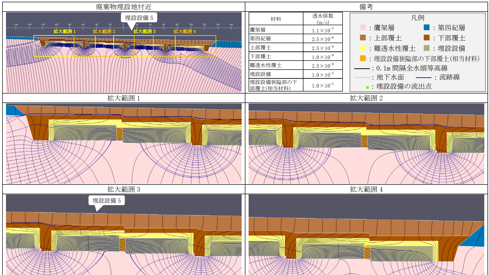
第1図 2次元地下水浸透流解析結果(確からしい設定 1,000年後) (6/9) <埋設設備5の流出点を通る流跡線>
