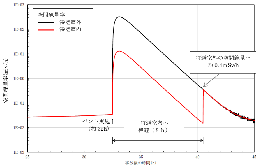
図 23-1 待避室内外の空間線量率
