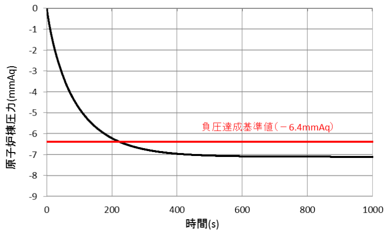
図2 原子炉棟圧力の時間変化
