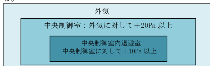
図 59 - 6 - 1 中央制御室及び中央制御室待避室 正圧化圧力
