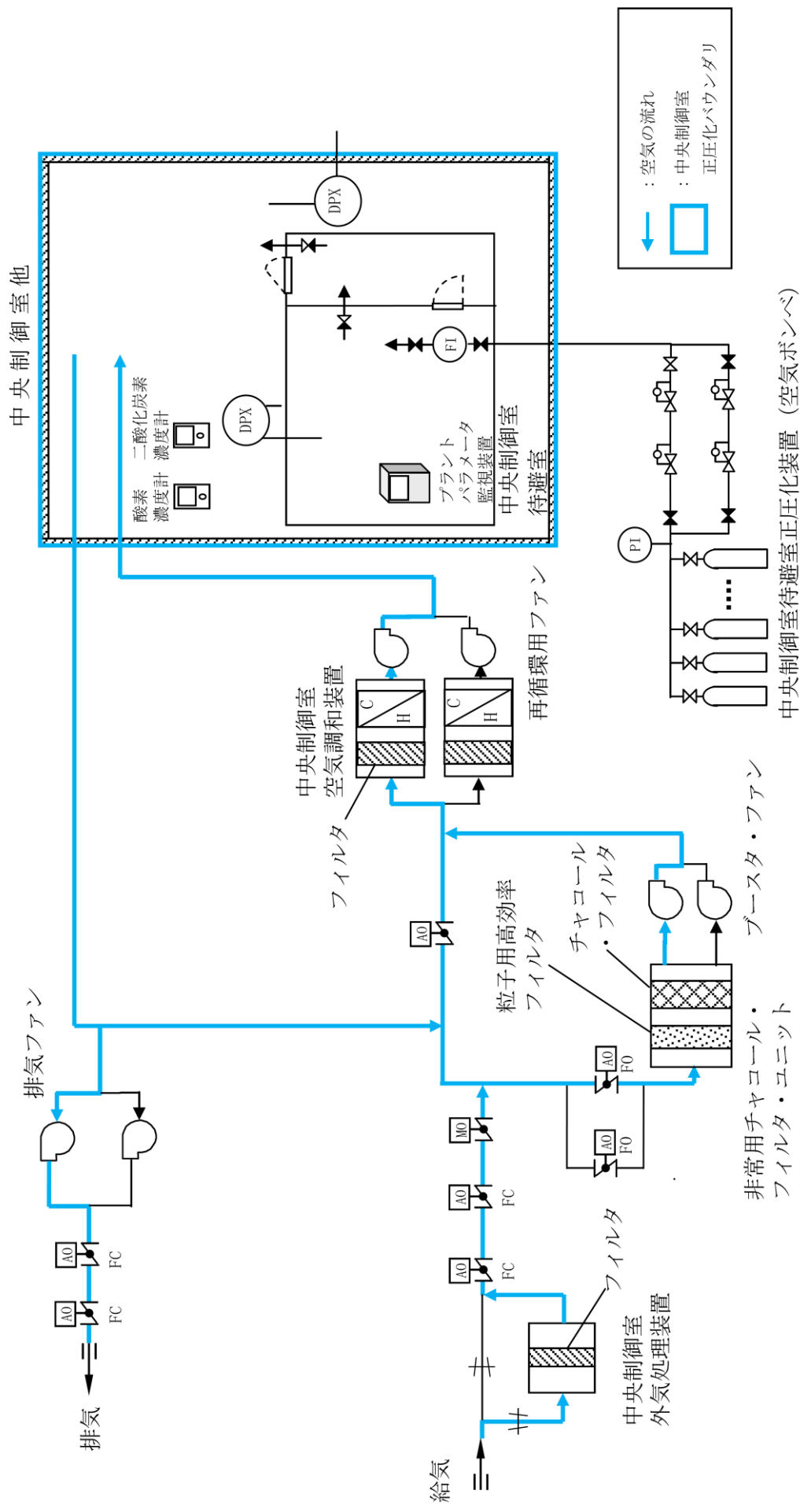
図 59-4-3 中央制御室換気系及び中央制御室待避室正圧化装置（空気ボンベ） 概略系統図 （非常時運転モード（外気連続少量取入モード））
