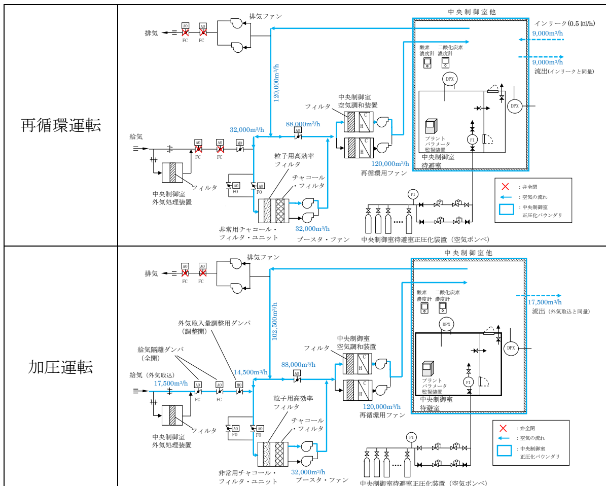
図1 中央制御室換気系 系統概要
