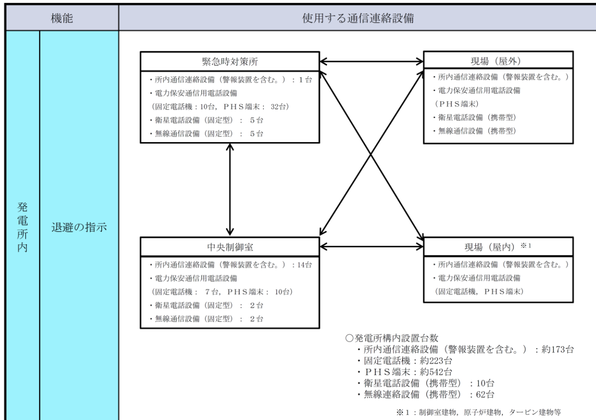
図 59-6-3 機能毎に必要な通信連絡設備（発電所内）
