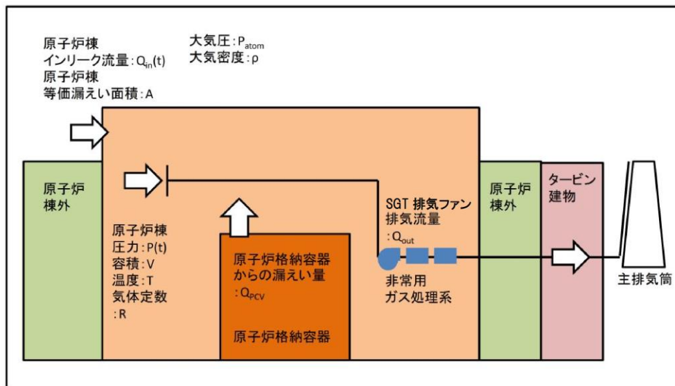
図1 原子炉棟の圧力評価モデル
