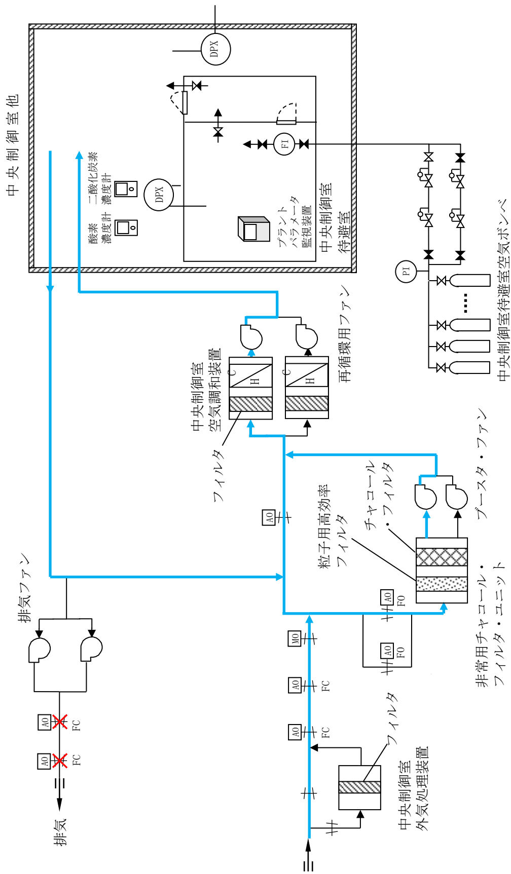
図3 中央制御室換気系の概要図
