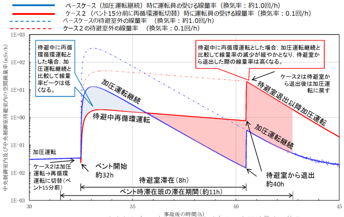
図24-2 中央制御室内の空間線量率の推移
