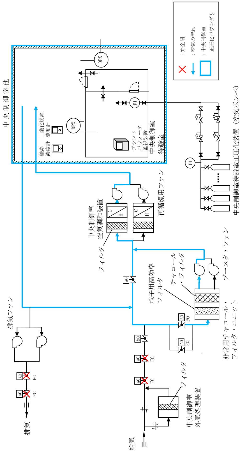
図 59-4-2 中央制御室換気系及び中央制御室待避室正圧化装置 (空気ポンプ) 概略系統図 (非常時運転モード (系統隔離運転))
