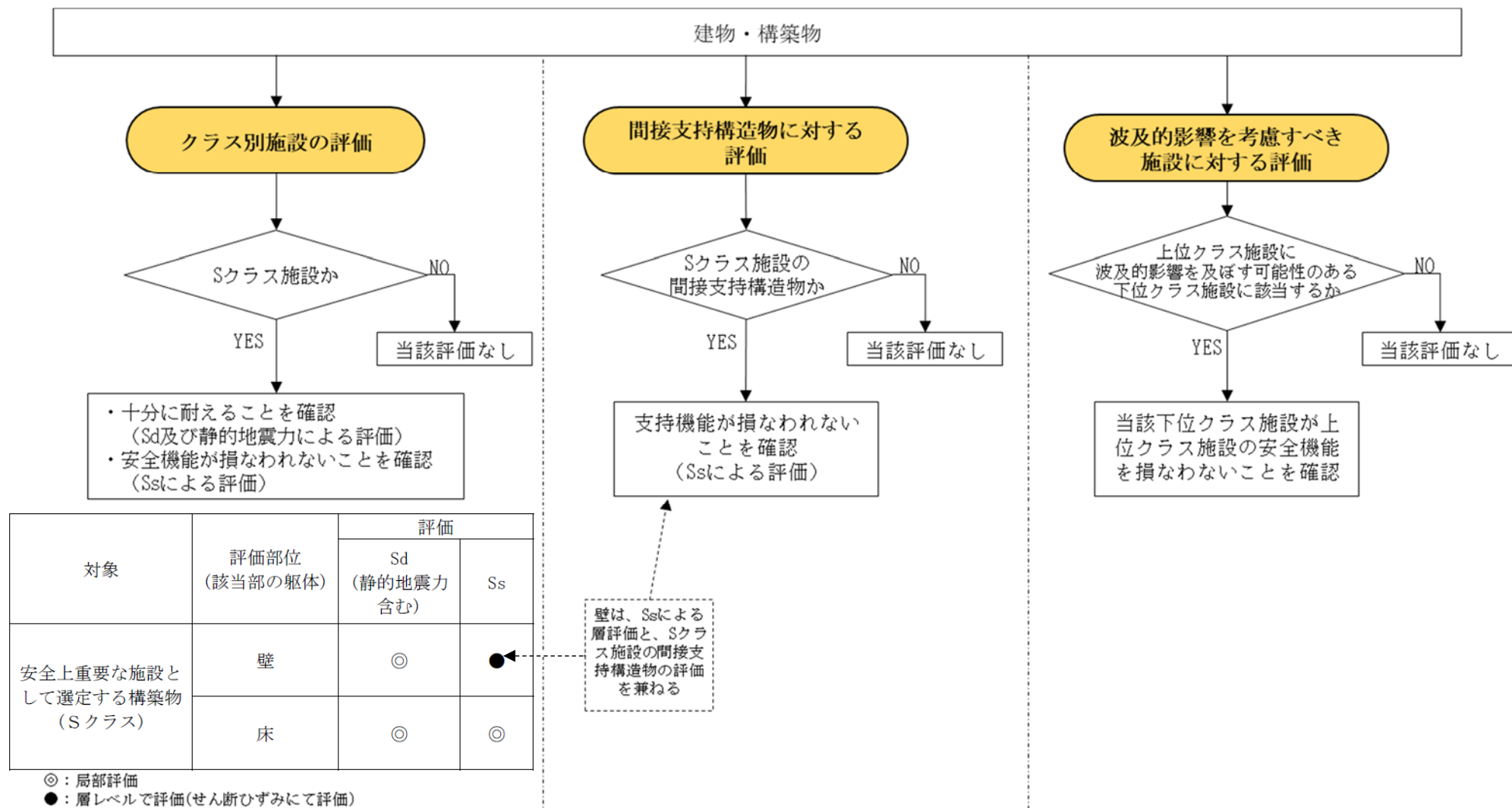
別添1図 建屋の耐震評価の考え方
