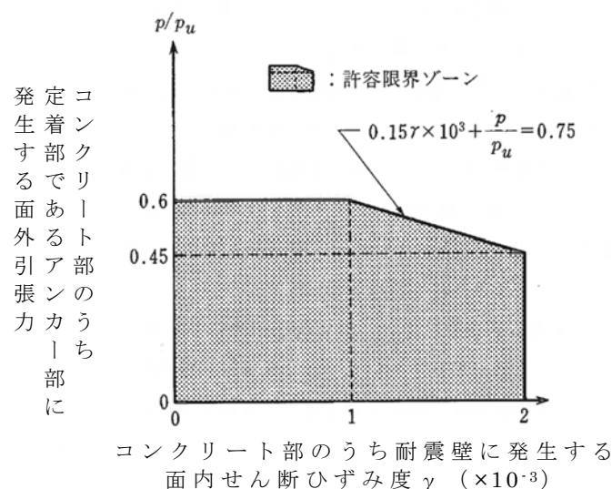
第 3-1 図 面内せん断ひずみ度と面外引張力に関する許容 限界ゾーン
