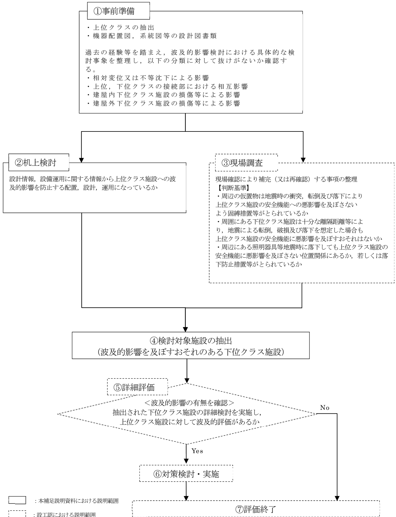
第 2-16-1 図 波及的影響評価に係る検討フロー
