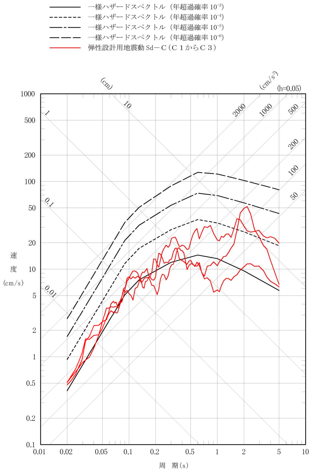
添5第15図(2) 弾性設計用地震動 Sd-C (C 1 から C 3) と 同様ハザードスペクトルの比較 (鉛直方向)
