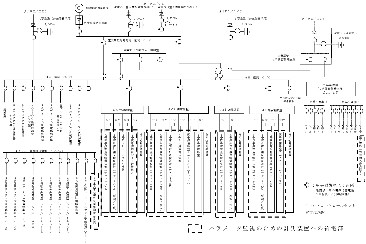
第 2 図 重大事故等対処用制御盤及び重大事故等対処用入出力盤の電源系統概略図 (4 号機)
