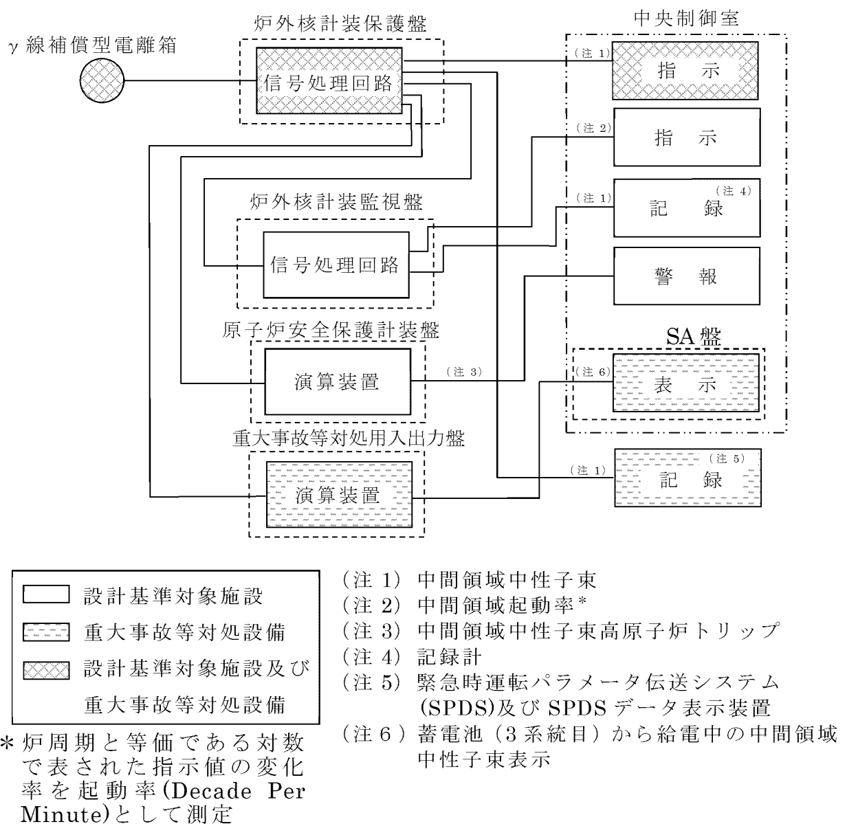
第2図 中間領域計測装置の概略構成図
