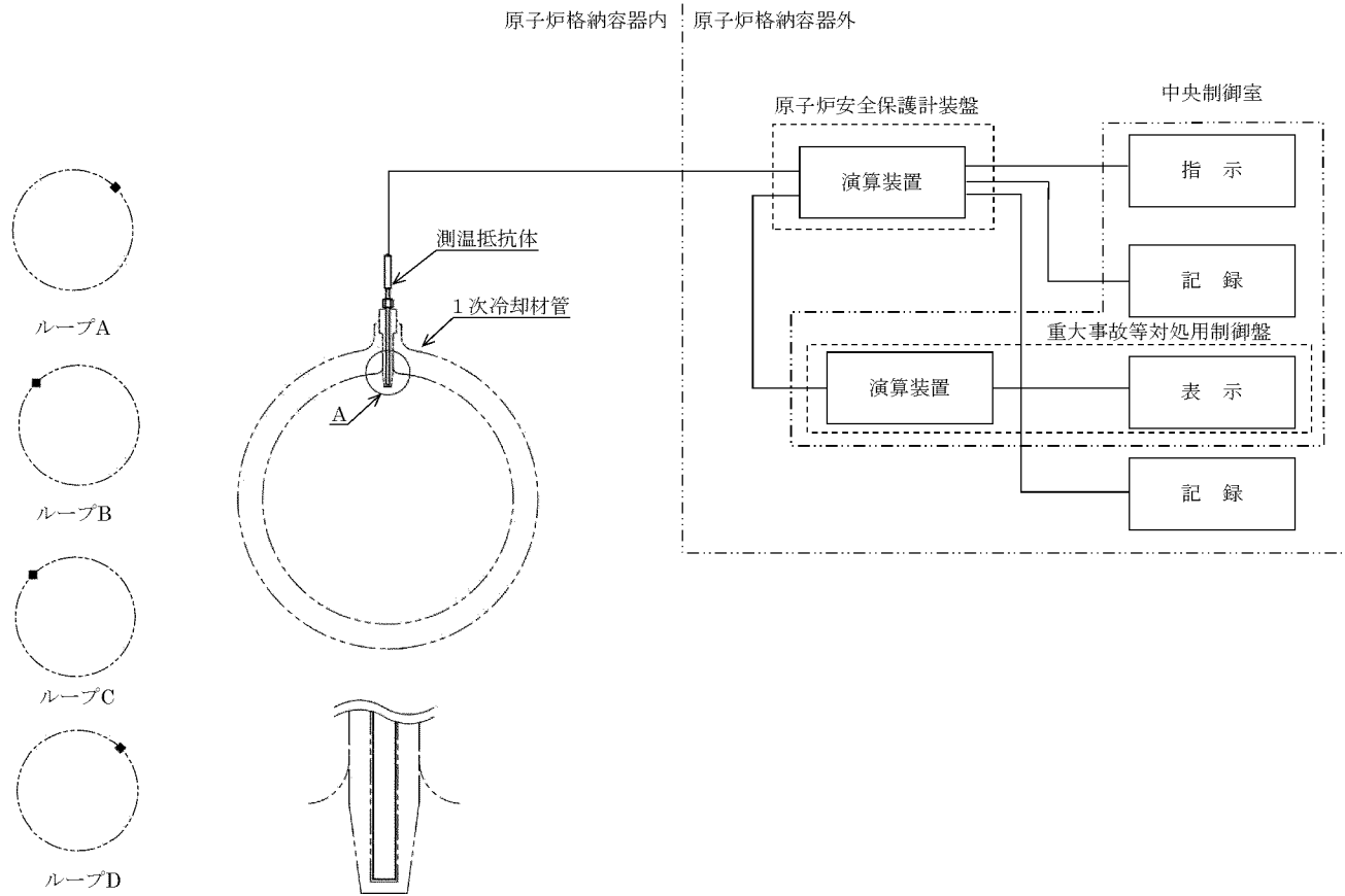
1次冷却材高温側温度(広域) ※上に示すループ A,B,C,D の流れ 方向は全て⊗
