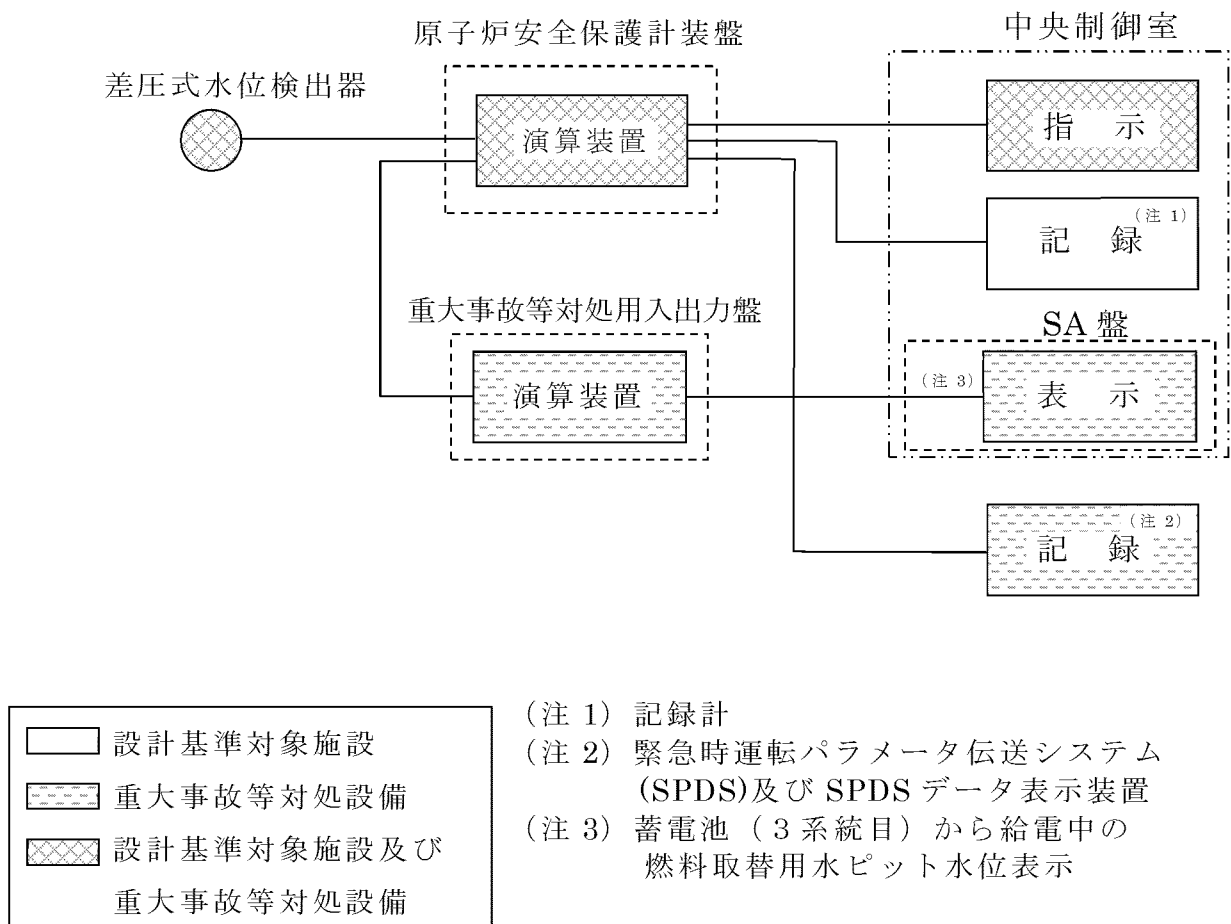
第 17 図 燃料取替用水ピット水位の概略構成図
