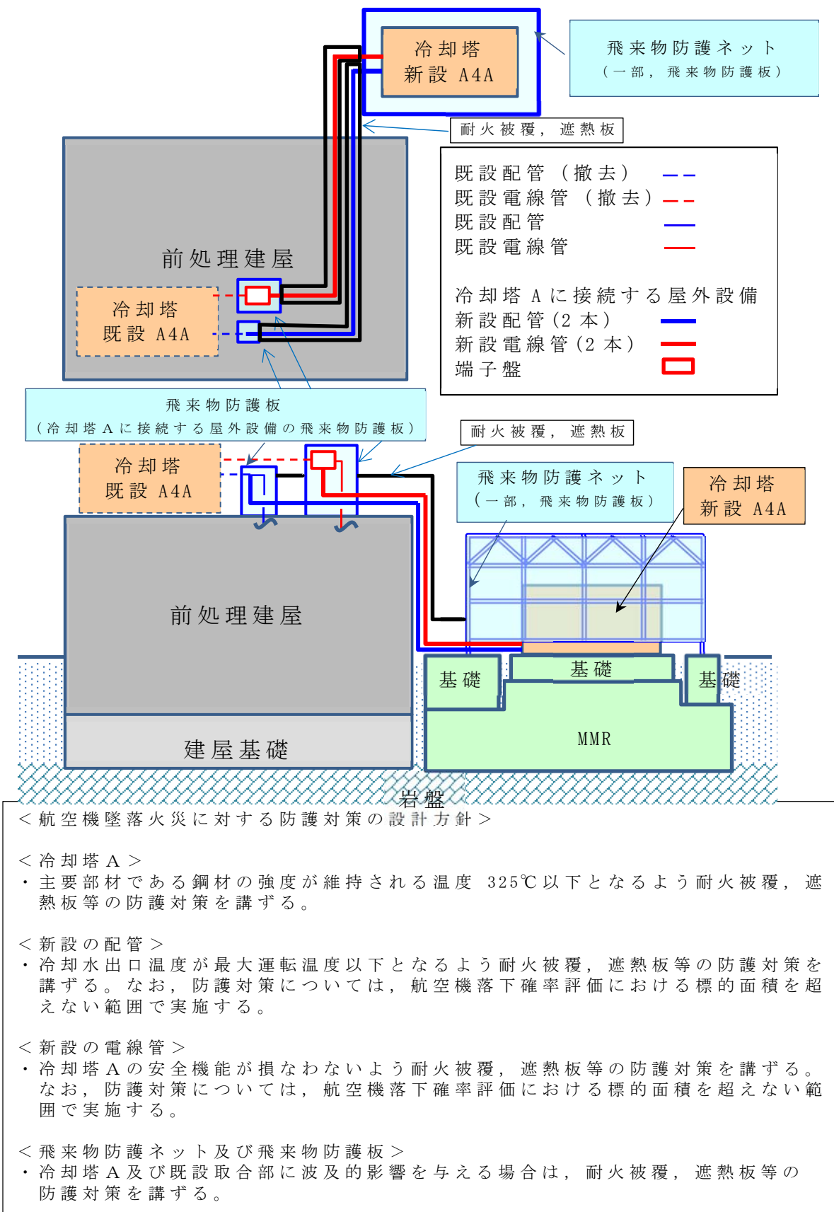
第 5 図 航空機墜落火災に対する防護対策の設計方針
