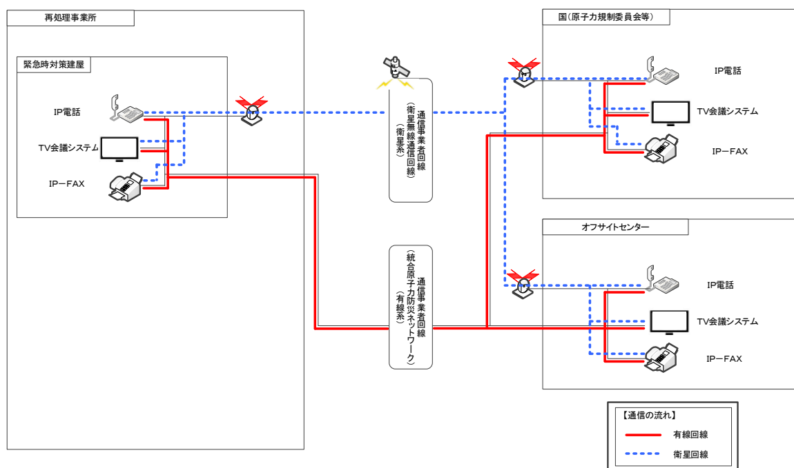
第2-12-8図 再処理事業所外への通信設備の概要
