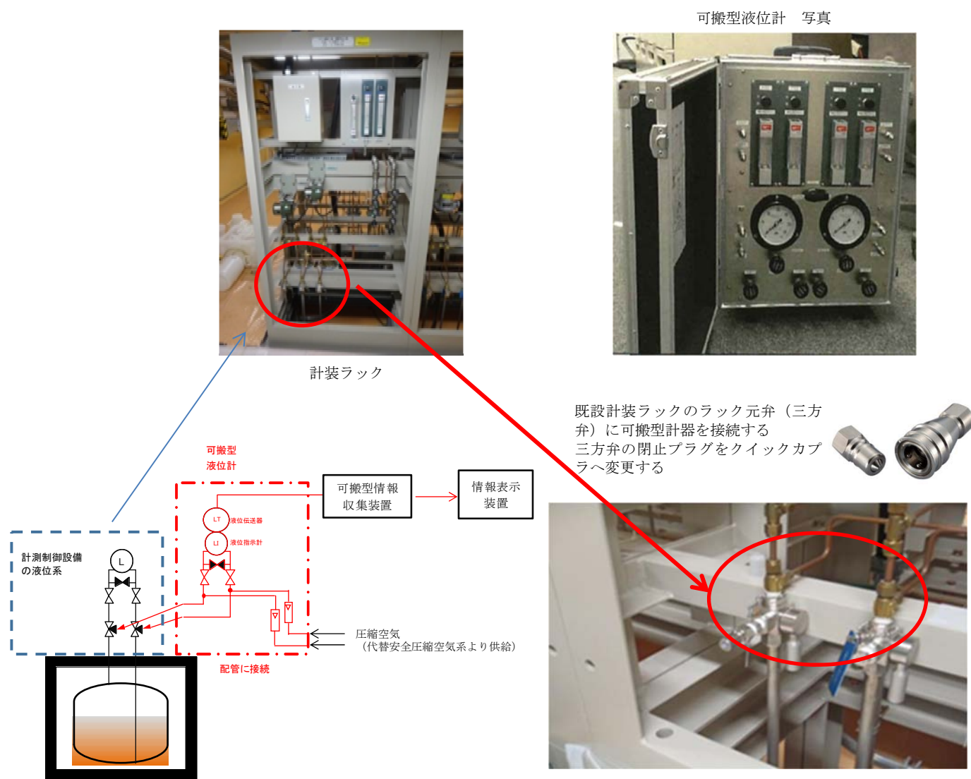
図4 貯槽液位の計測（エアパージ式）の接続図
