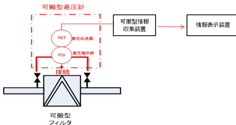
図5 フィルタ差圧の計測（差圧式）の接続図
