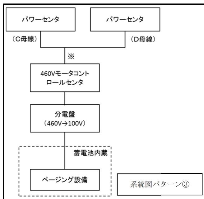
第13-1図 ページング設備における蓄電池への給電パターン系統図
