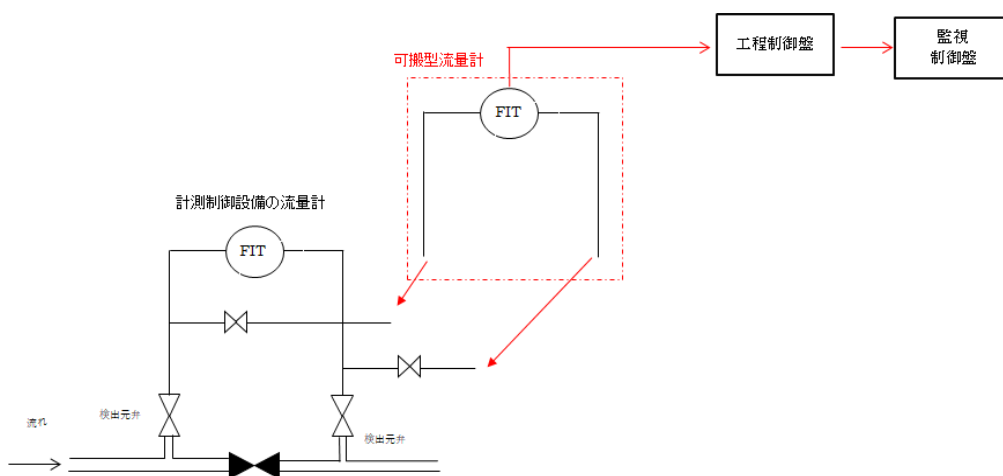
図2-1 臨界事故の拡大を防止するための設備 貯槽掃気圧縮空気流量の計測（熱式）の接続図
