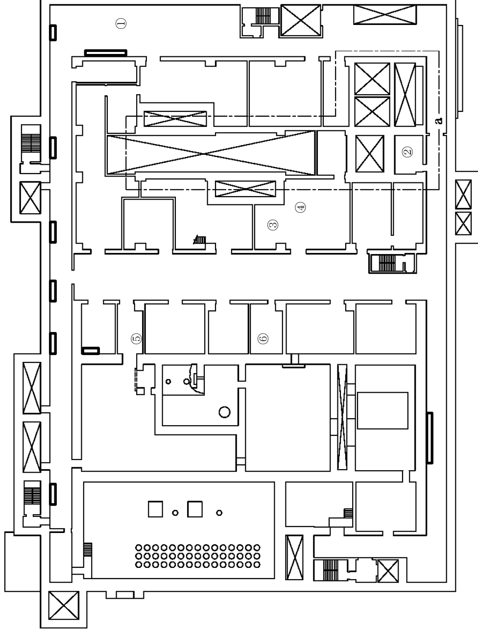
第6.2.1-69図 放射線分解により発生する水素による爆発に対処するために必要な計装設備の機器配置図 (高レベル廃液ガラス固化建屋 地下1階)
