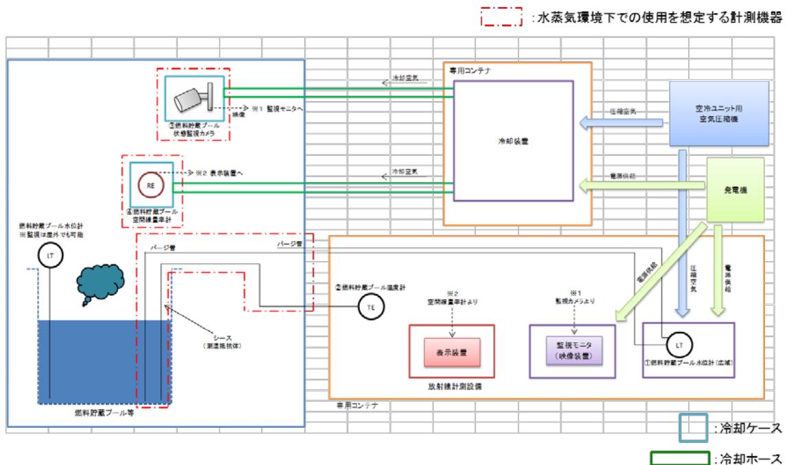
燃料貯蔵プール等の監視設備の全体概要図
