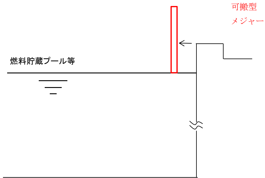
図 1 3 燃料貯蔵プール等の水位計測（メジャー）の接続図
