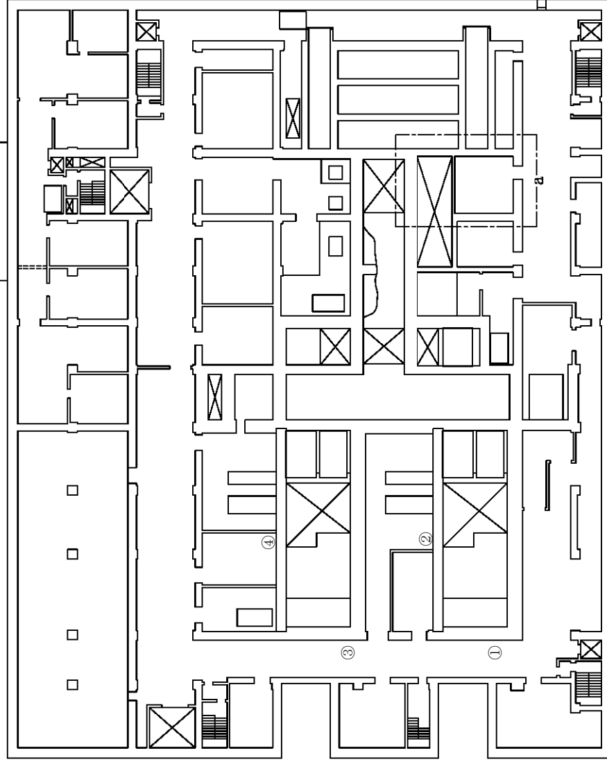
第6.2.1-6 図 臨界事故の拡大を防止するために必要な計装設備の機器配置図 (前処理建屋 地下1階)
