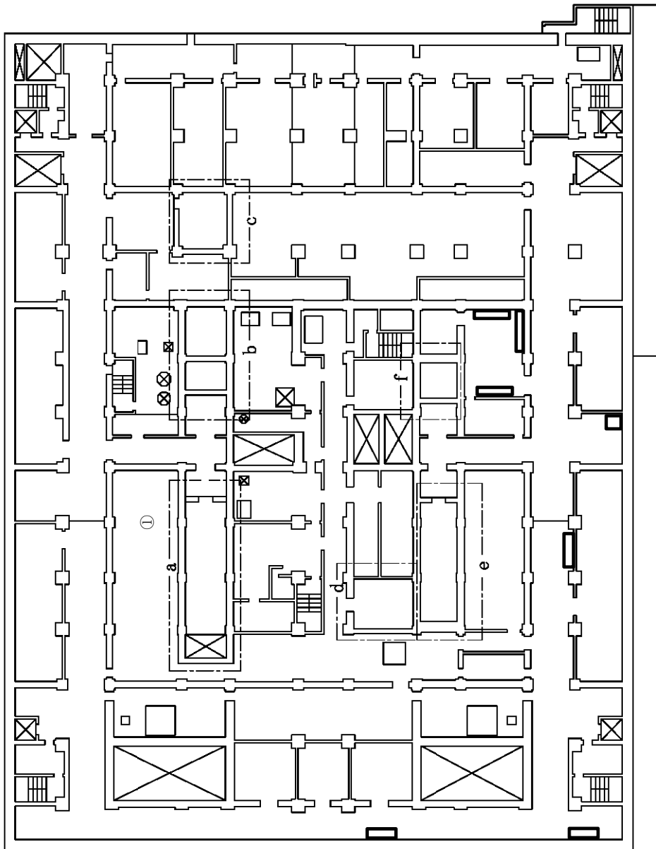
第6.2.1-35図 冷却機能の喪失による蒸発乾固に対処するために必要な計装設備の機器配置図 (精製建屋 地上4階)
