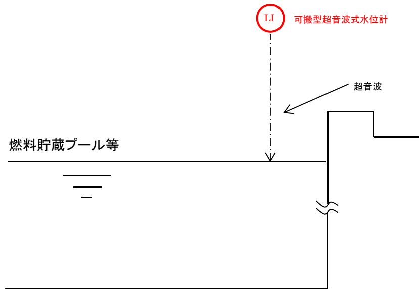
図10 燃料貯蔵プール等の水位計測（超音波式）の接続図
