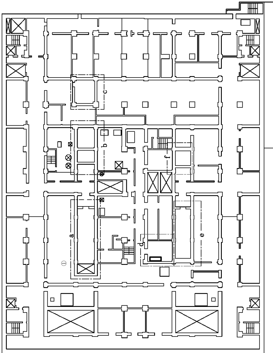
第6.2.1-14図 臨界事故の拡大を防止するために必要な計装設備の機器配置図 (精製建屋 地上4階)
