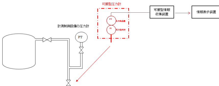
図7 圧縮空気自動供給貯槽圧力の計測（圧力式）の接続図
