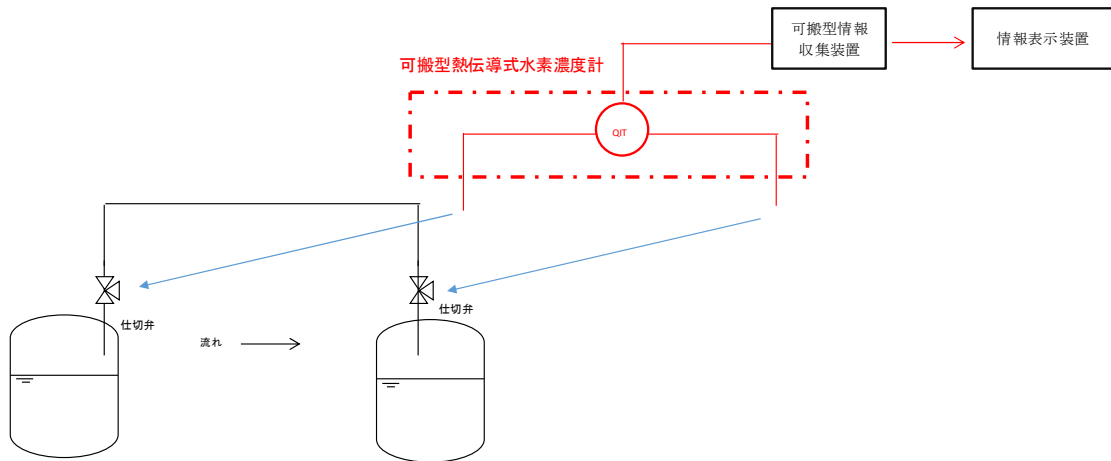
図9 水素濃度の計測（熱伝導式）の接続図
