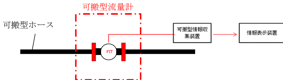
図8 送水流量の計測（電磁式）の接続図
