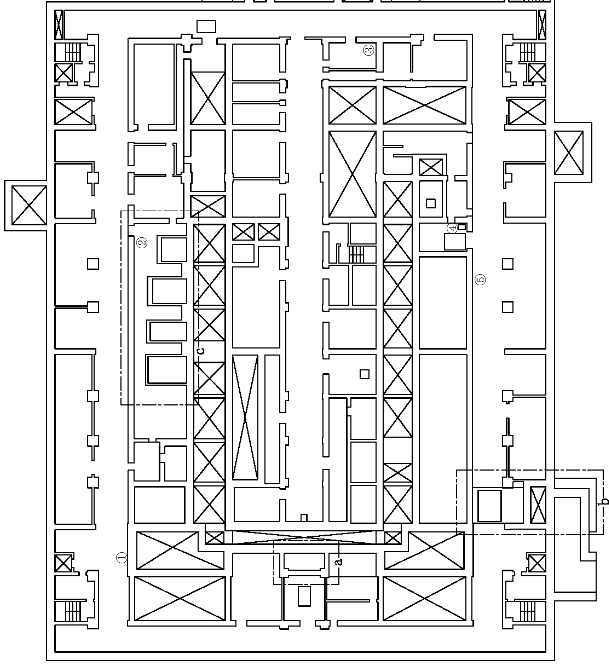
第6.2.1-96図 工場等外への放射性物質等の放出を抑制するために必要な計装設備の機器配置図 (精製建屋 地下1階)
