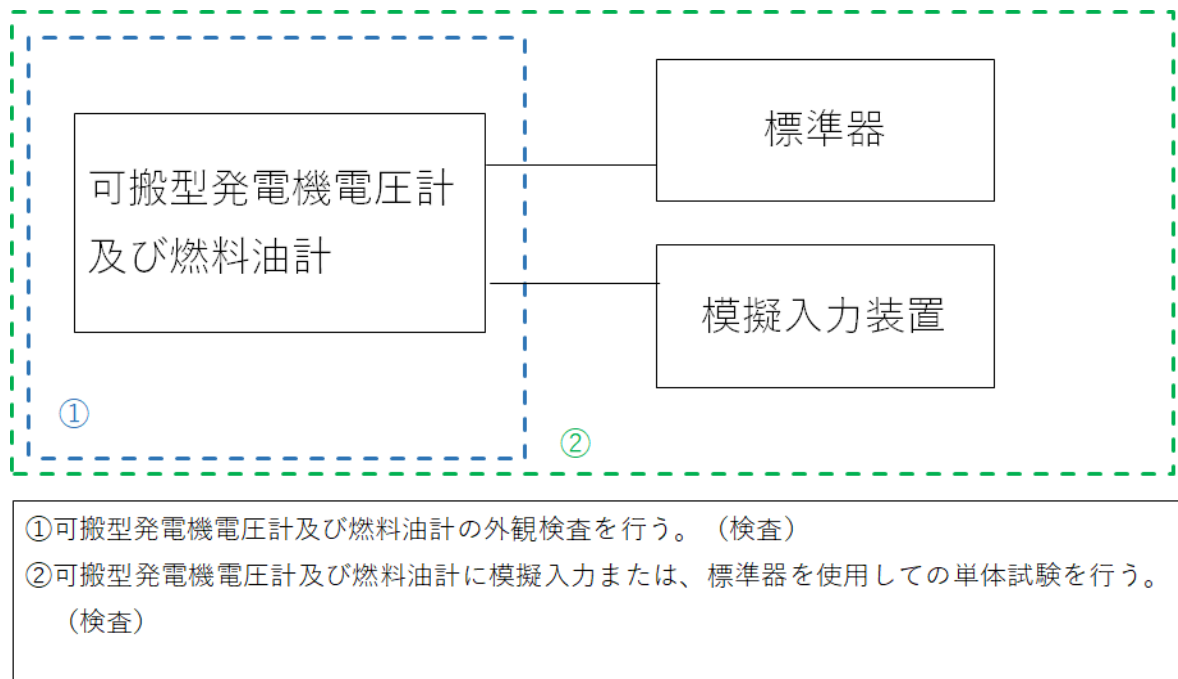
第 2 - 5 - 9 図 電圧計／燃料油計の試験検査
