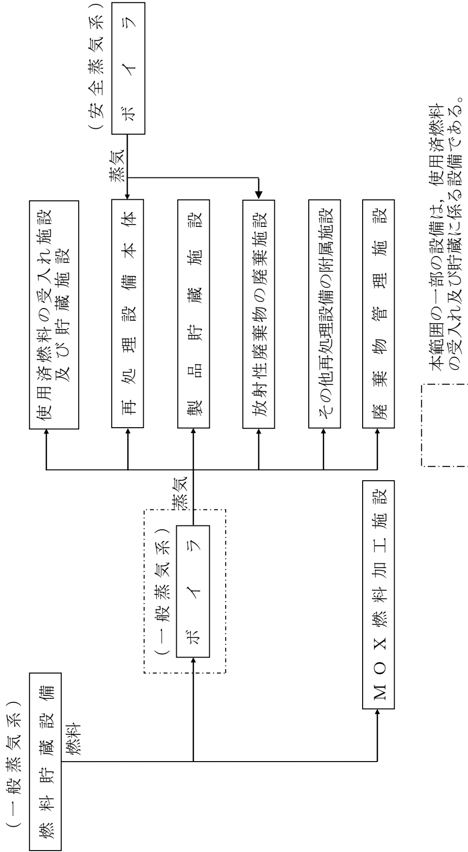
第 9.6-1 図 蒸気供給設備系統概要図
