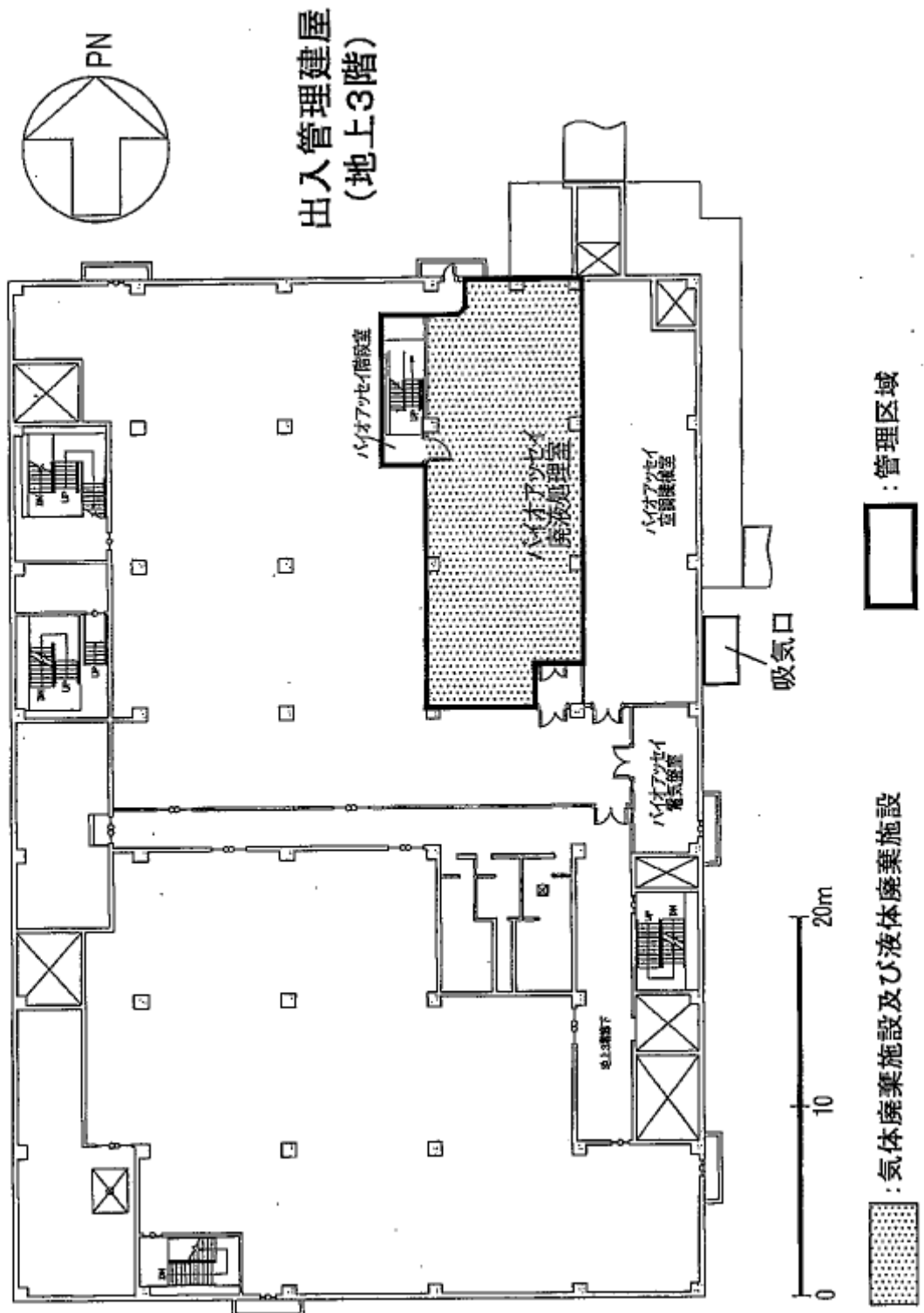
図5.1-(15)-1 出入管理建屋の気体廃棄施設及び液体廃棄施設及び位置図 (地上3階)
