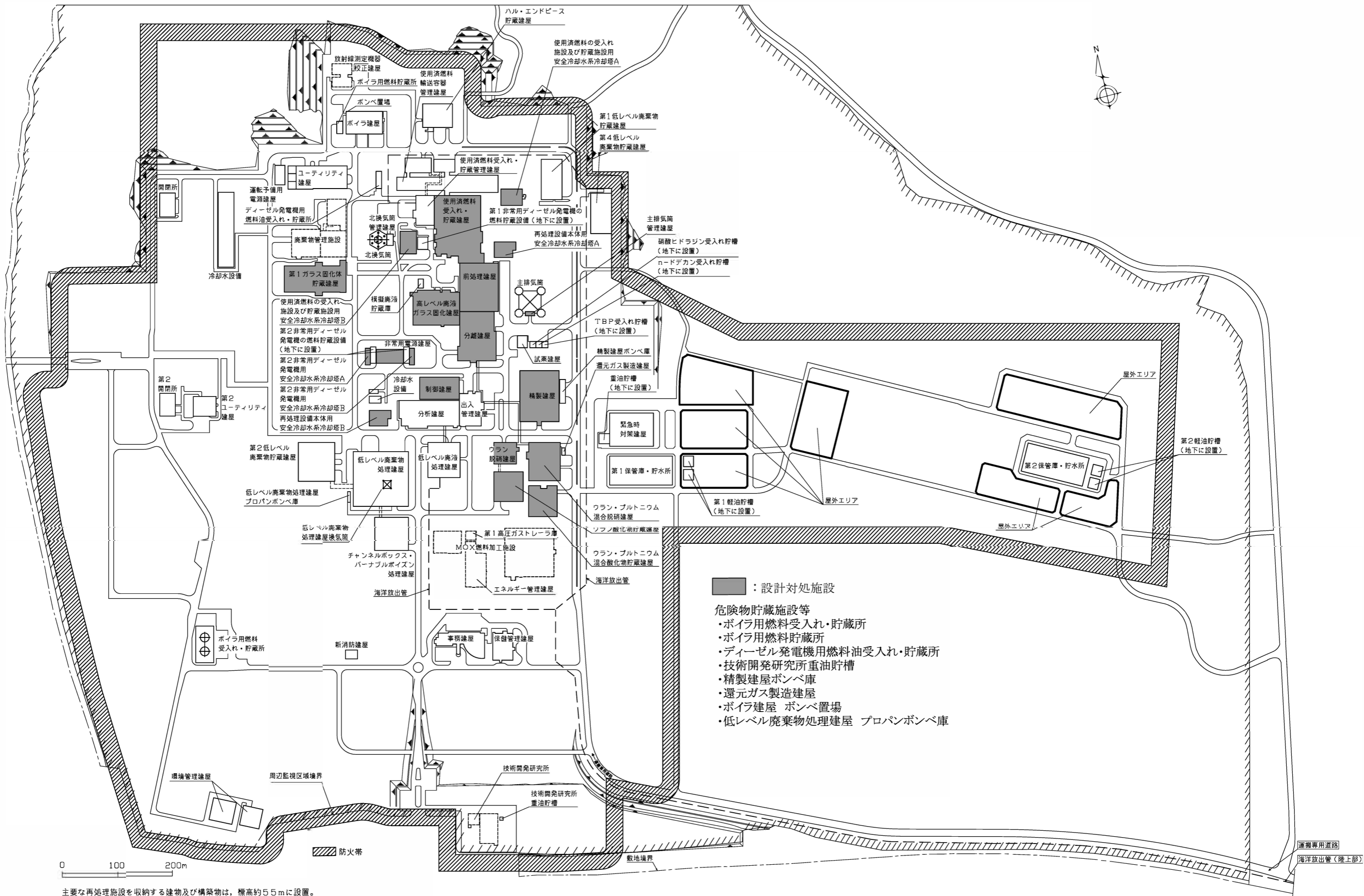
第1.7.11-1図 防火帯, 設計対処施設, 危険物貯蔵施設等の配置図
