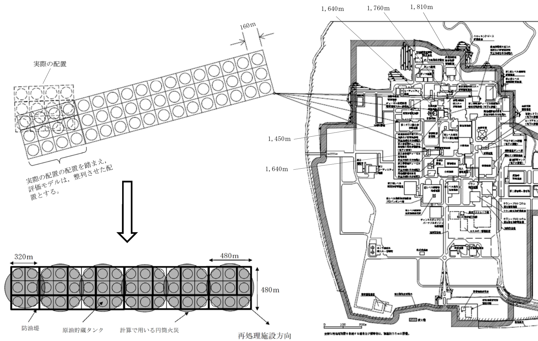
第9.12図 (外部火災) 円筒火災モデルのイメージ
