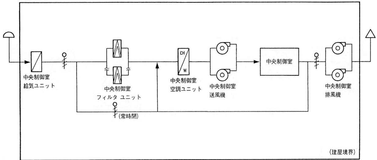
第9. 13図 (外部火災) 制御建屋中央制御室換気設備系統概要
