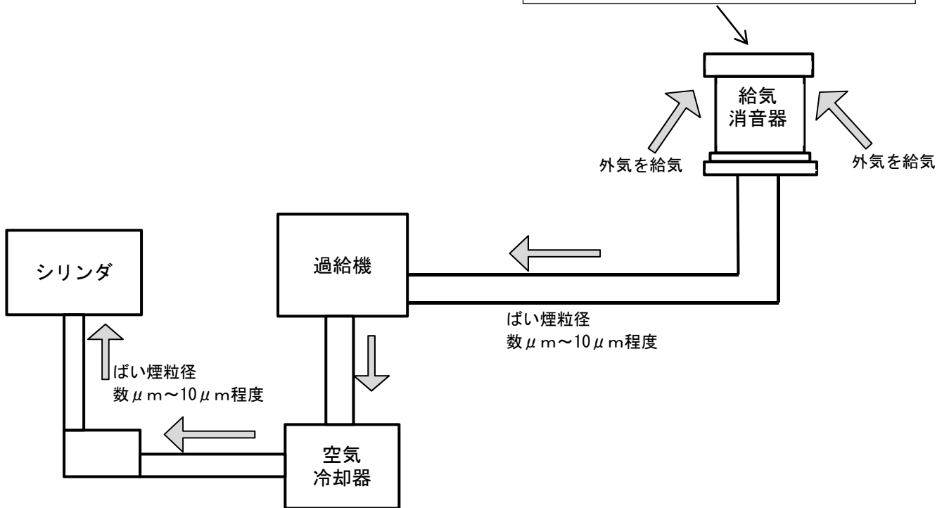
図1 非常用ディーゼル発電機の吸気系の概要
