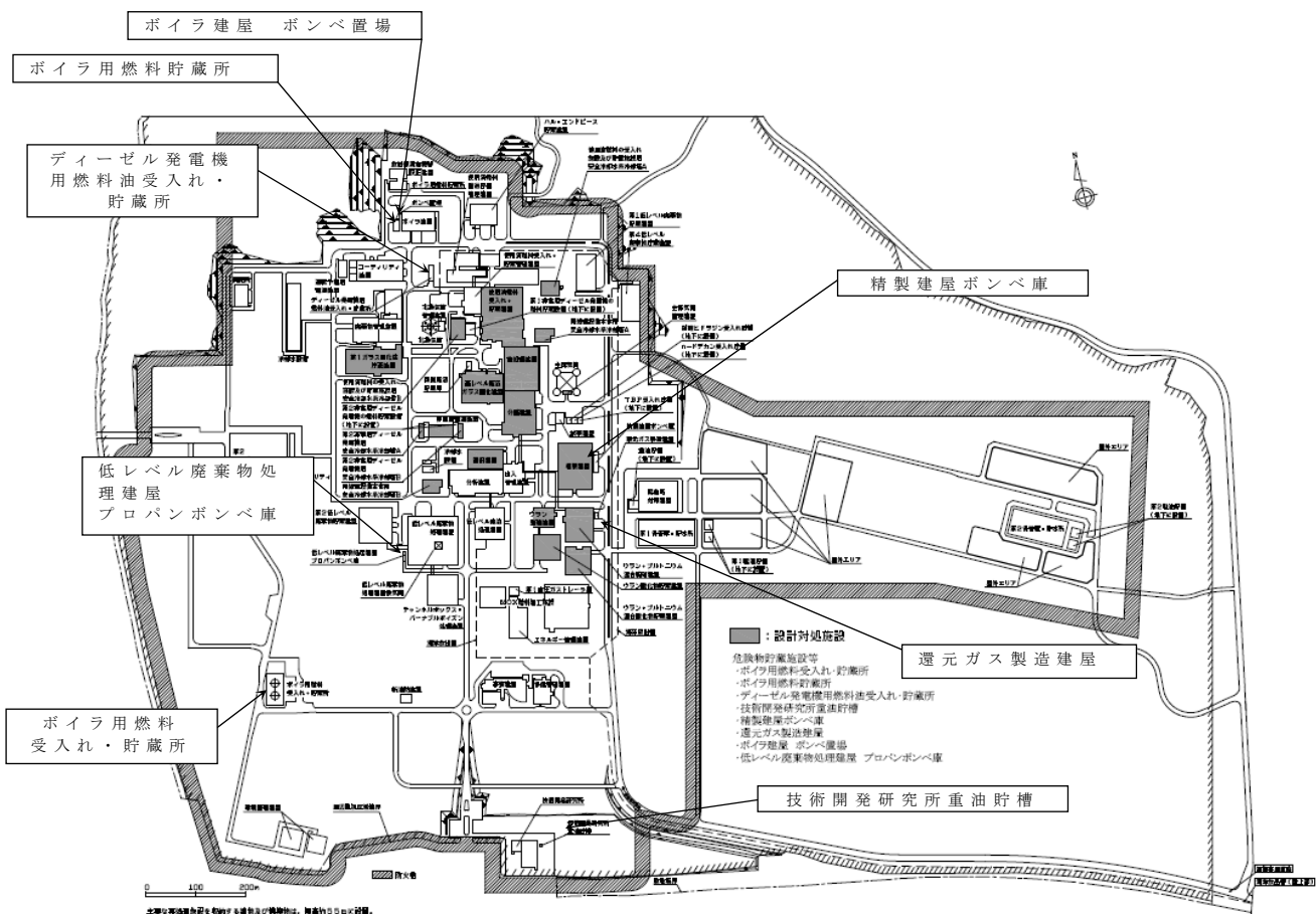
第6図 敷地内の危険物タンク等の配置図
