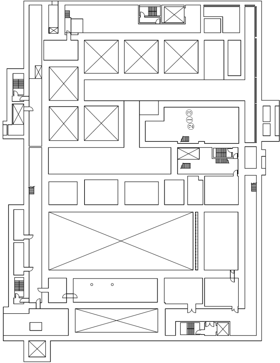
第 35.3 図(II) 代替安全冷却水系（貯槽等への注水）の注水接続口配置図及び接続口一覧 高レベル廃液ガラス固化建屋（地下3階）
