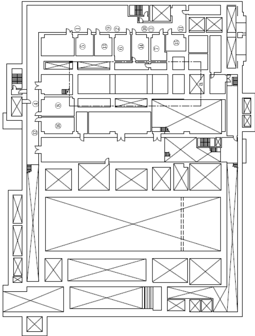
第 35.2 図(9) 代替安全冷却水系（内部ループへの通水による冷却）の通水接続口配置図及び接続口一覧 高レベル廃液ガラス固化建屋（地下2階）
