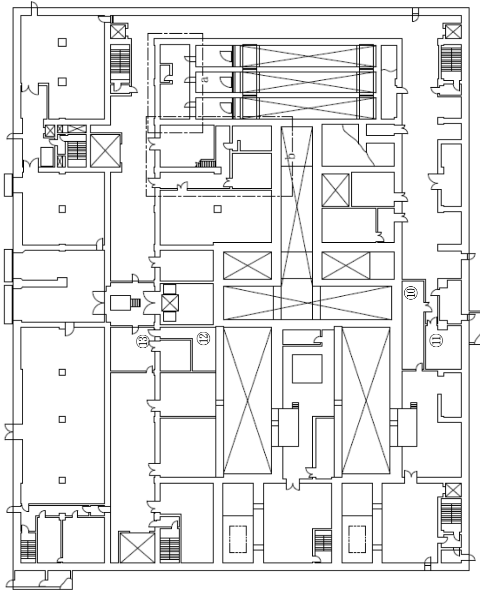
第 35.4 図(3) 代替安全冷却水系 (冷却コイル等への通水による冷却) の通水接続口配置図及び接続口一覽 前処理建屋 (地上1階)
