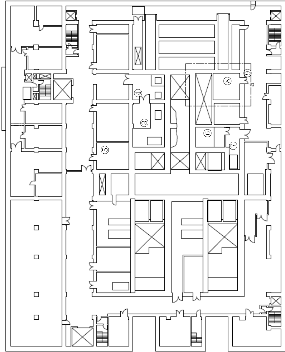
第9.5-15 図(2) 代替安全冷却水系（冷却コイル等への通水による冷却）の通水接続口配置図及び接続口一覧 前処理建屋（地下1階）
