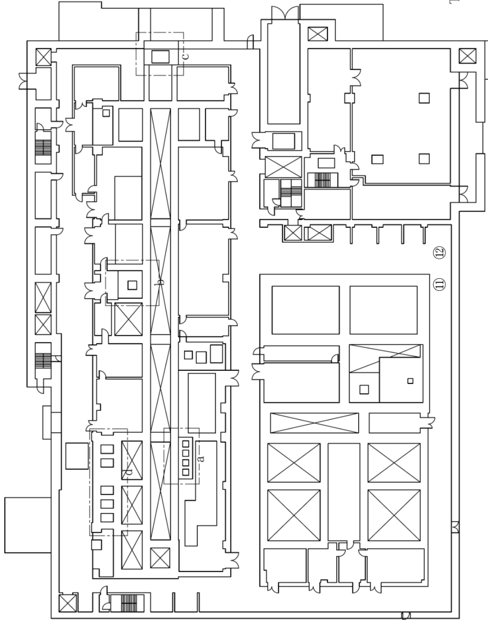
第9.5-9図(4) 代替安全冷却水系（内部ループへの通水による冷却）の通水接続口配置図及び 接続口一覧 分層建屋（地上1階）
