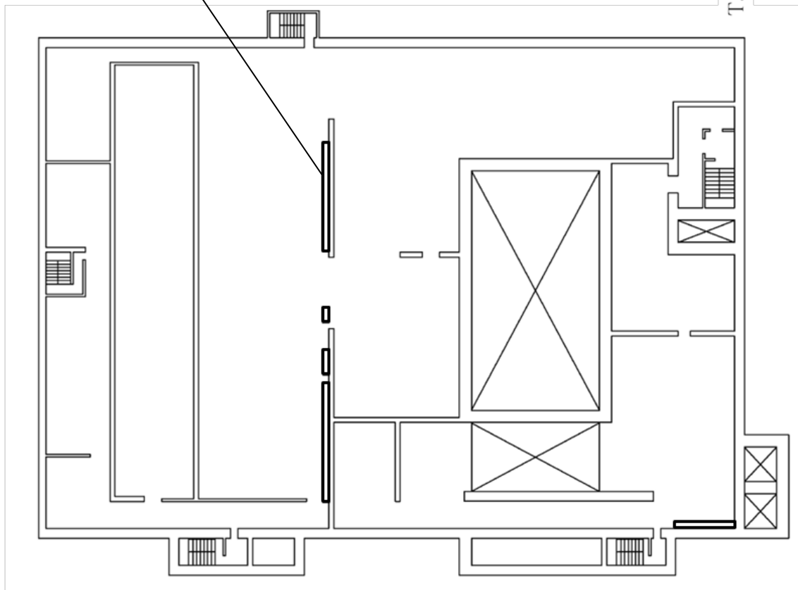
第 9.5-14 図(5) 代替安全冷却水系（冷却コイル等への通水による冷却）の機器及び 接続口配置概要図 高レベル廃液ガラス固化建屋（地上2階）
