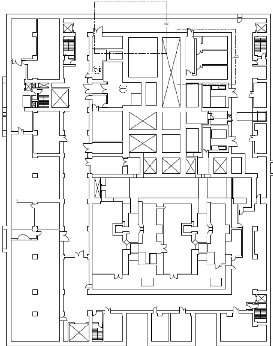
第 35.4 図(1) 代替安全冷却水系（冷却コイル等への通水による冷却）の通水接続口配置図及び接続口一覧 前処理建屋（地下3階）
