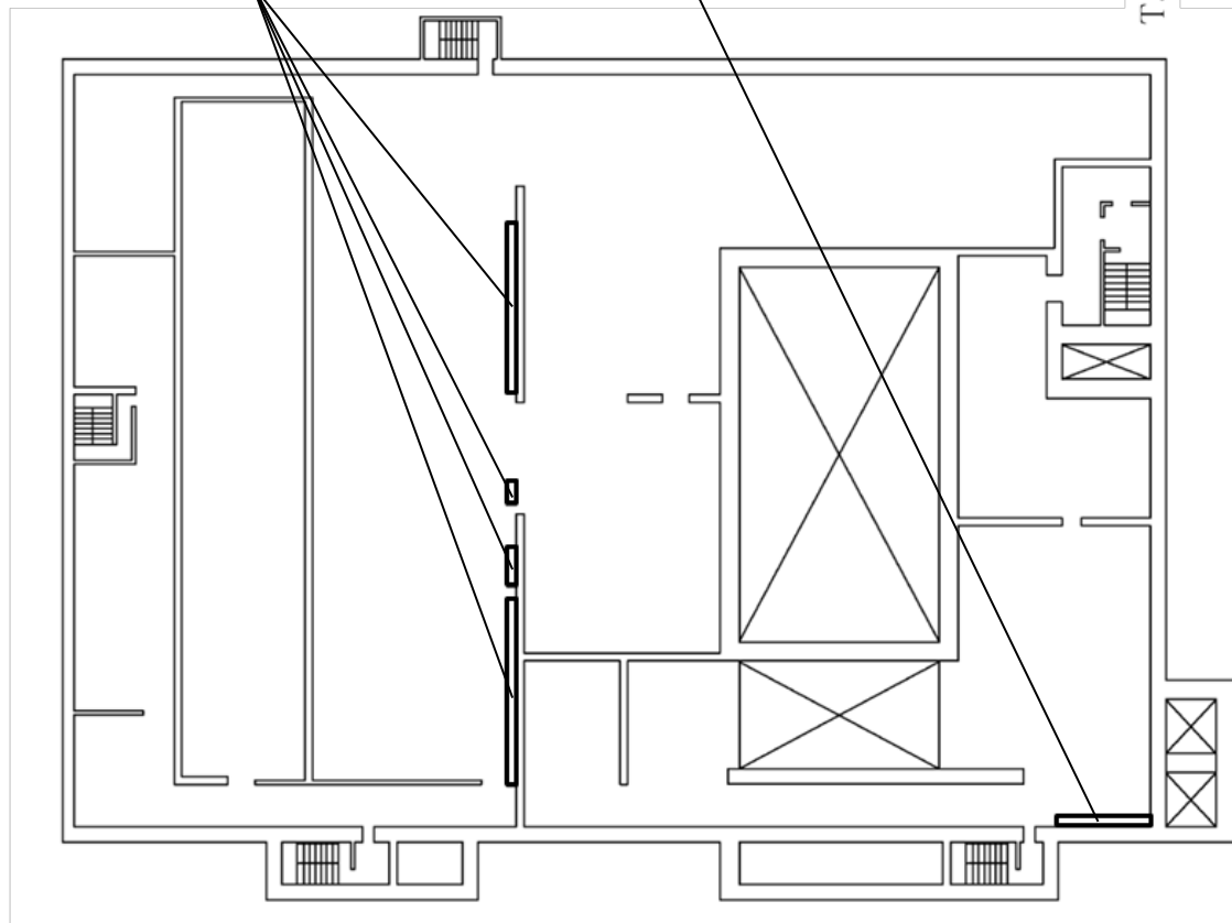
第9.5-11 図(27) 代替安全冷却水系（貯槽等への注水）の機器及び接続口配置概要図 高レベル廃液ガラス固化建屋（地上2階）
