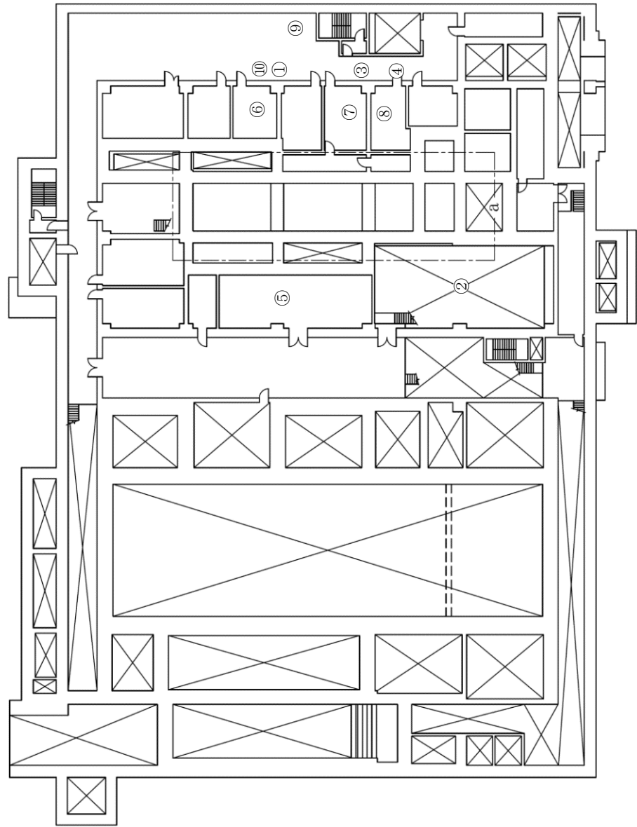
第 35.3 図(12) 代替安全冷却水系（貯槽等への注水）の注水接続口配置図及び接続口一覧 高レベル廃液ガラス固化建屋（地下2階）
