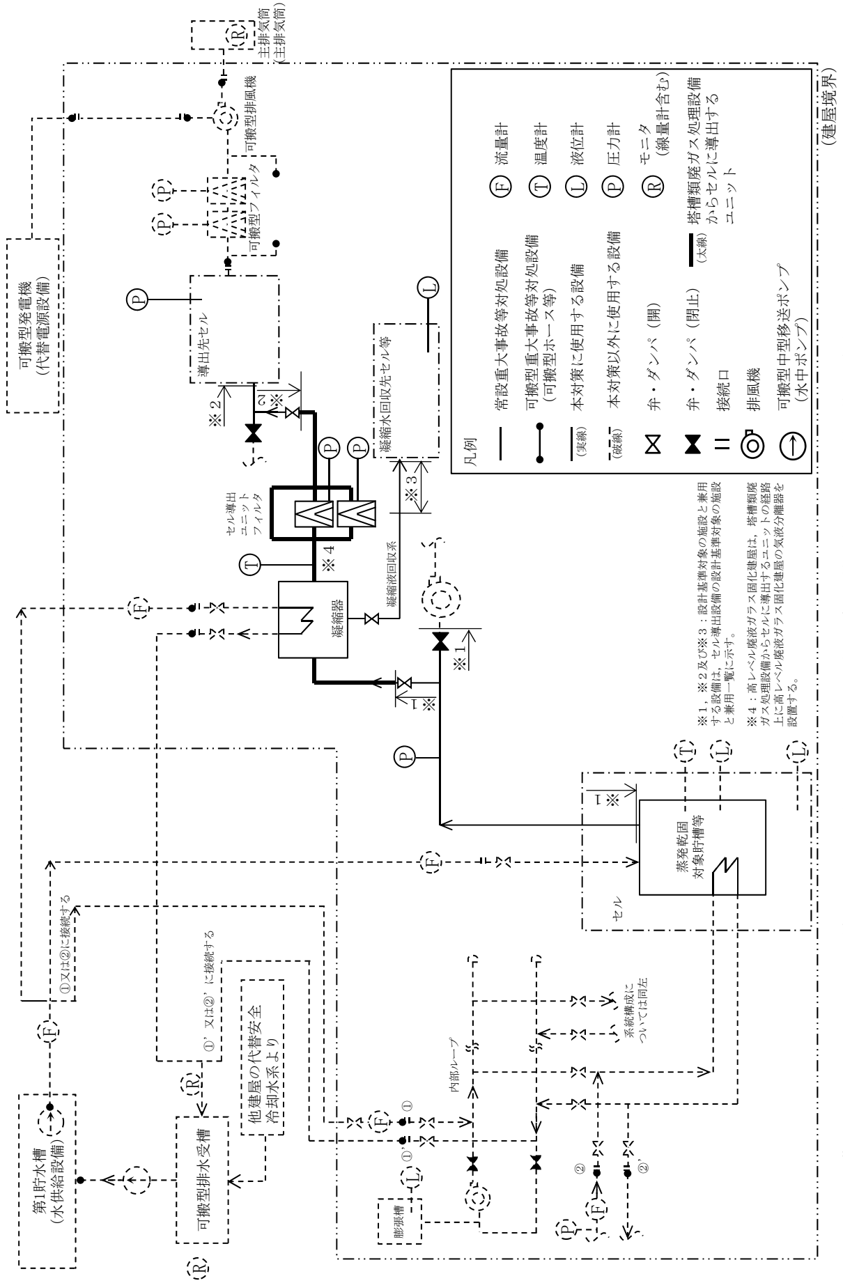
本図は、蒸発乾固に対処するための系統概要である。可搬型ホース等及び可搬型ダクト等の敷設ルート、接続箇所、個数及び位置については、ホース敷設ルートごとに異なる。
