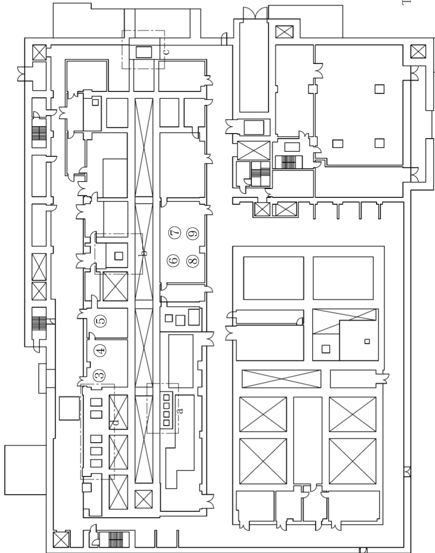
第 35.3 図(4) 代替安全冷却水系（貯槽等への注水）の注水接続口配置図及び接続口一覧 分離建屋（地上1階）
