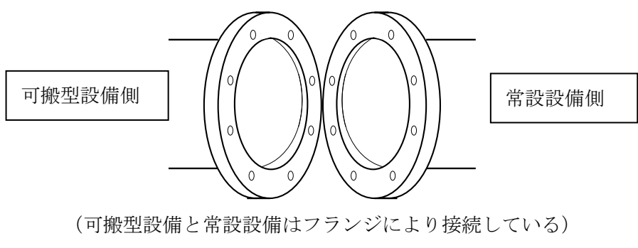
蒸発乾固に対処するための設備における可搬型設備と常設設備の接続図 高レベル廃液ガラス固化建屋 (地下1階) その3
