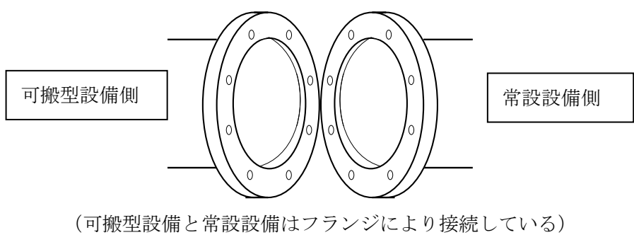
蒸発乾固に対処するための設備における可搬型設備と常設設備の接続図 高レベル廃液ガラス固化建屋（地下1階）その4
