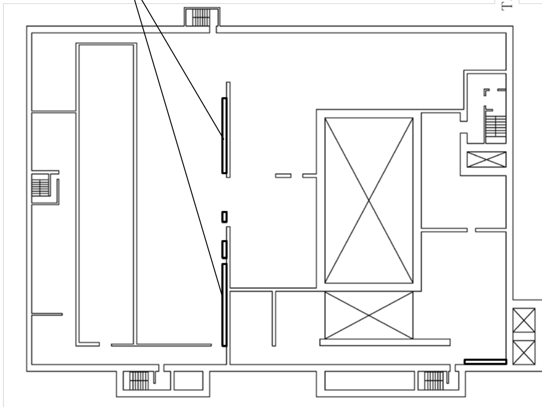
第7.2-39 図(28) 代替換気設備（セルへの導出経路の構築及び代替セル排気系による対応（蒸発乾固）の機器及び接続口配置概要図 高レベル廃液ガラス固化建屋（地上2階）
