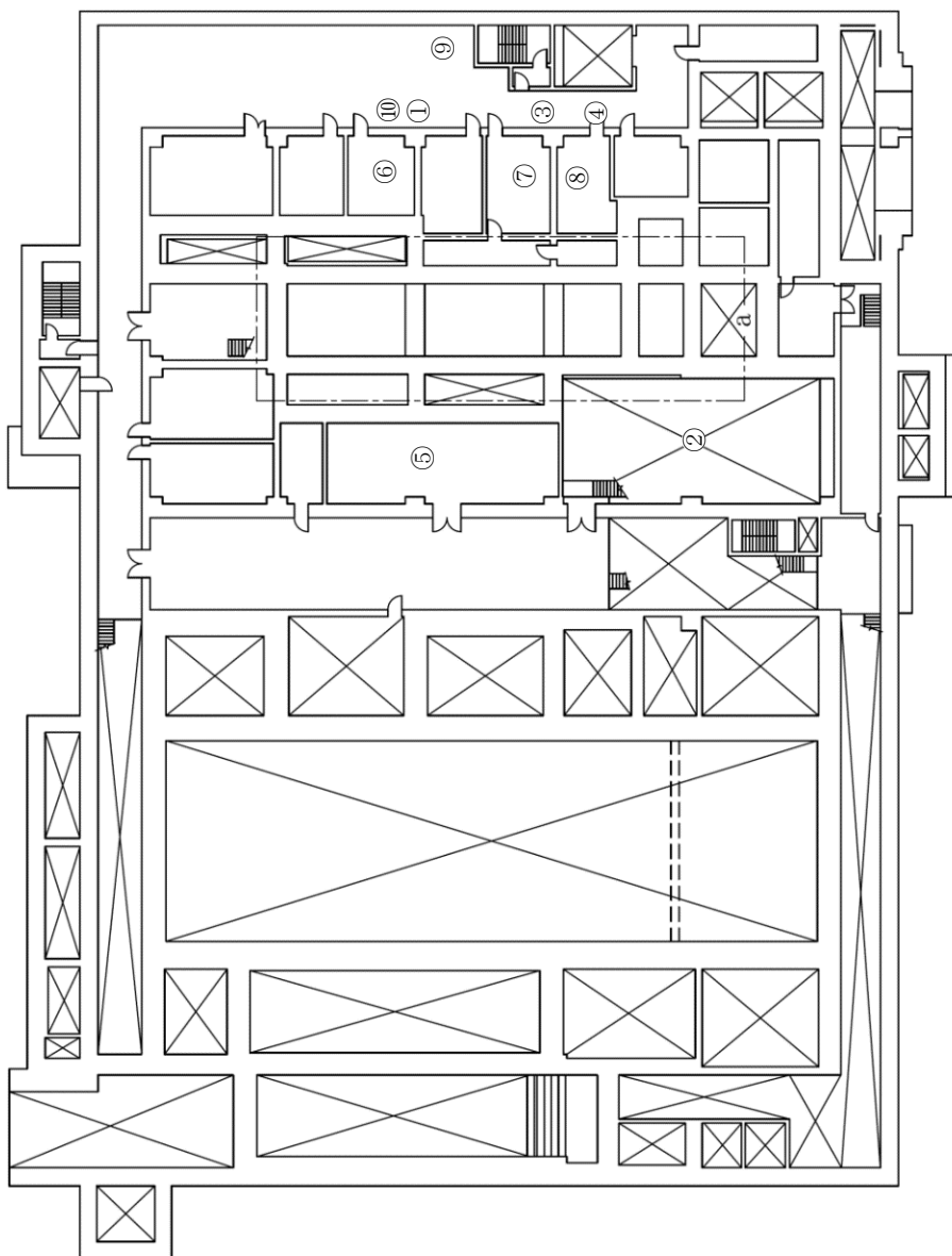
第 9.5-12 図(12) 代替安全冷却水系（貯槽等への注水）の注水接続口配置図及び接続口一覧 高レベル廃液ガラス原化建屋（地下2階）
