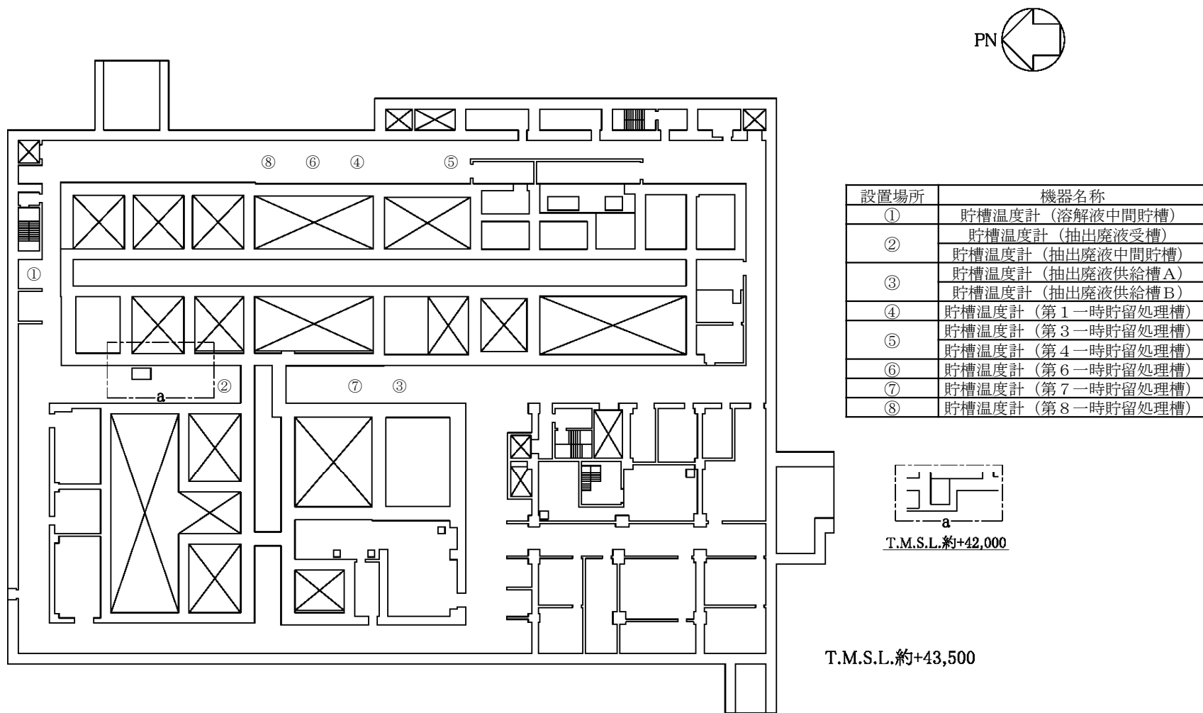
第6. 2. 1-23図 冷却機能の喪失による蒸発乾固に対処するために必要な計装設備の機器配置図 (分離建屋 地下 2 階)
