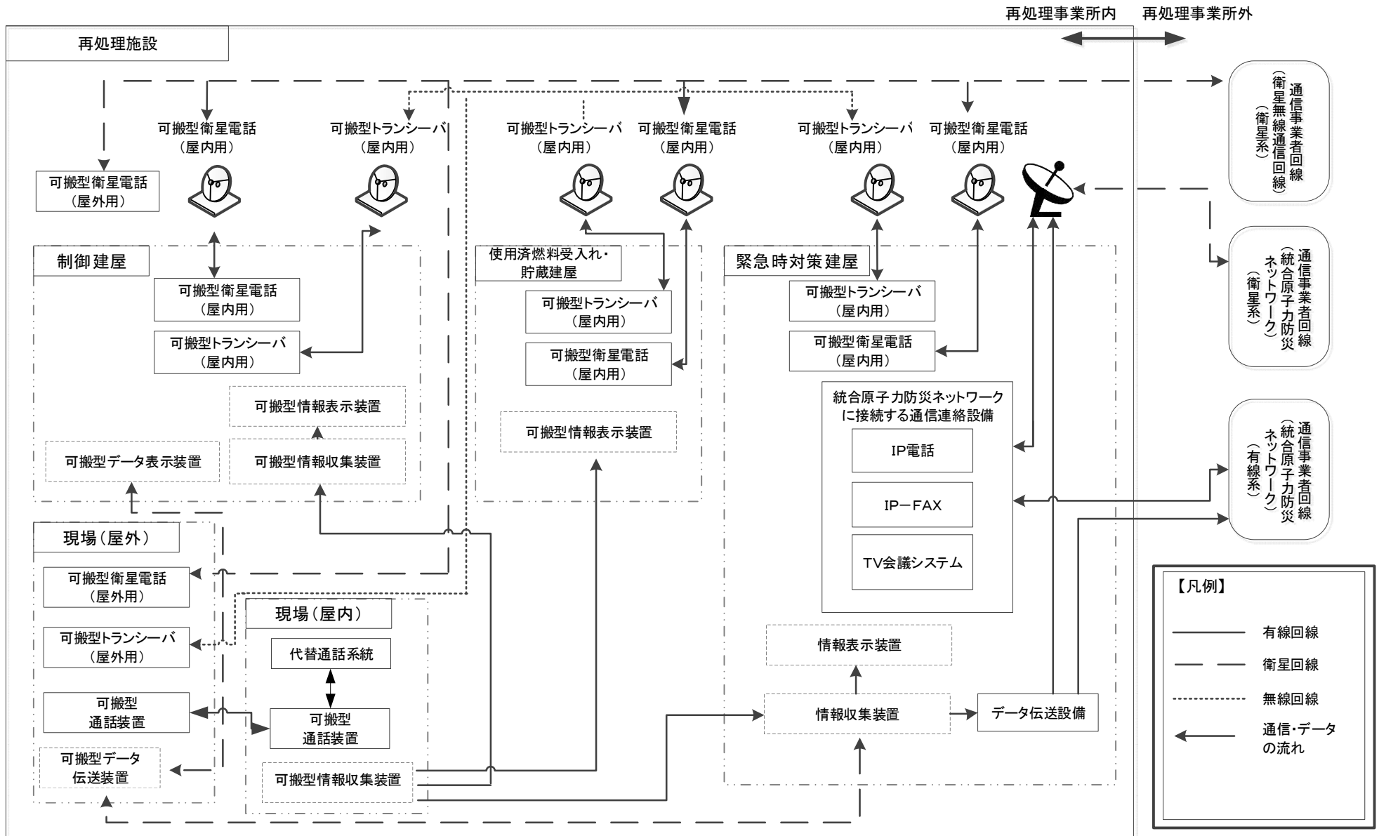
第 9.17.2-2 図 代替通信連絡設備の系統概要図
