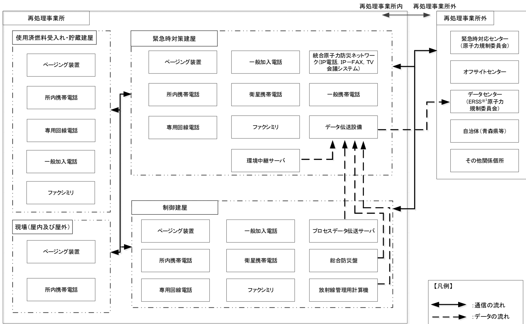
第 9.17.2-1 図 通信連絡設備の系統概要図
