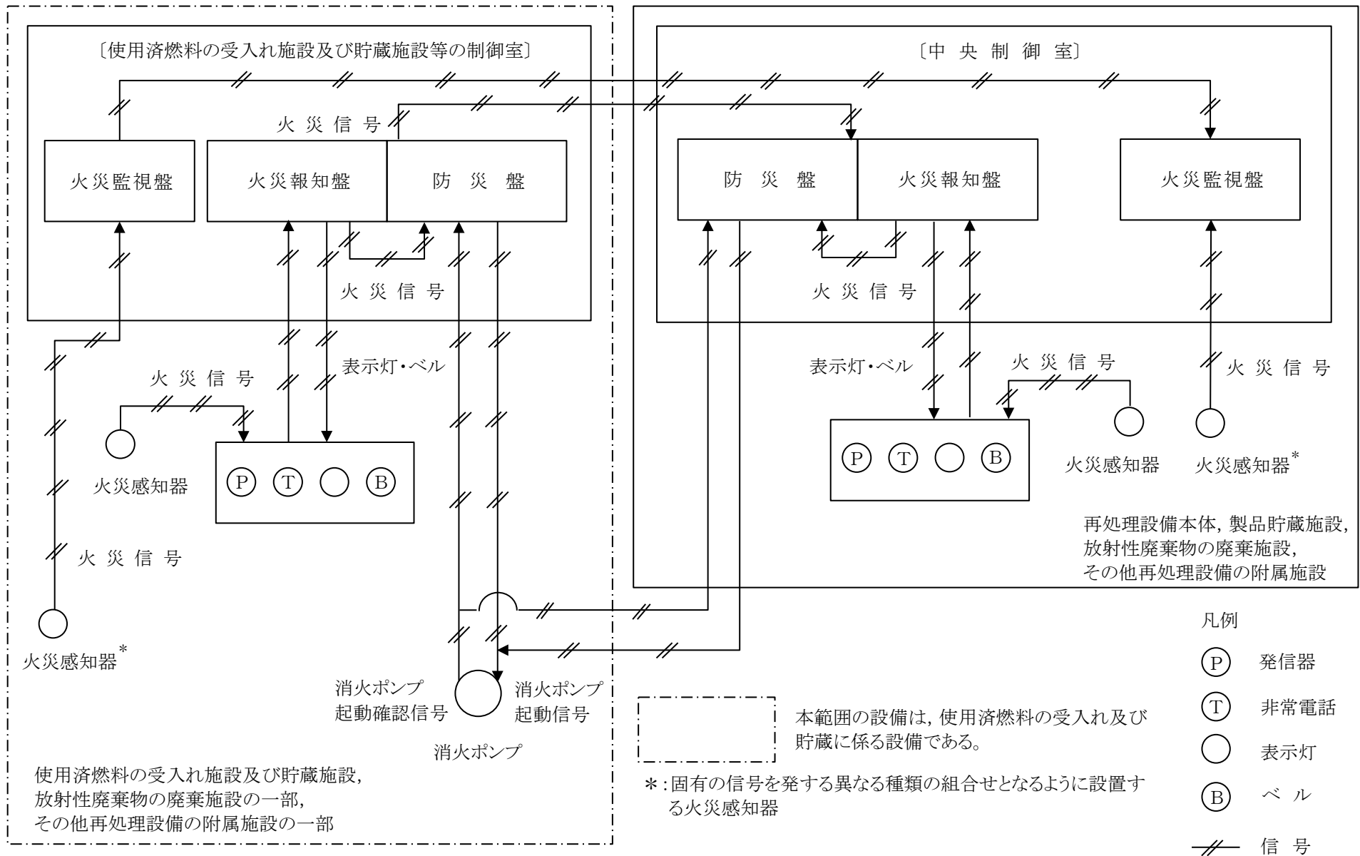
第 9.10-1 図 火災感知設備系統概要図
