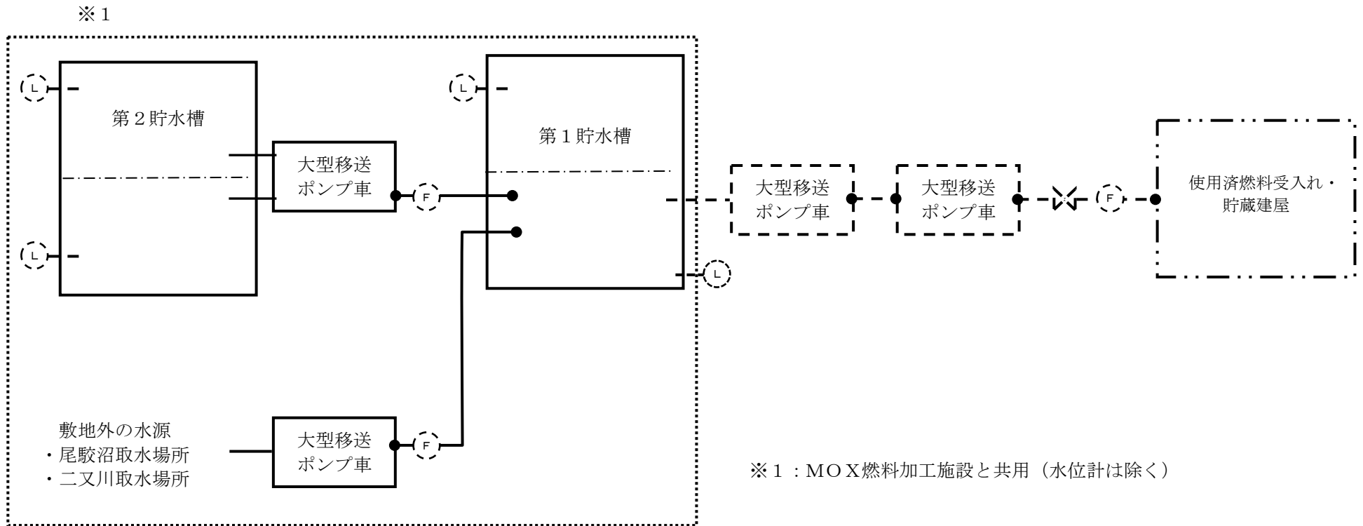
第9.4-3図 水供給設備の系統概要図 (燃料貯蔵プール等への水のスプレイ, 燃料貯蔵プール等への大容量の注水に係る 第1貯水槽への水の補給)
