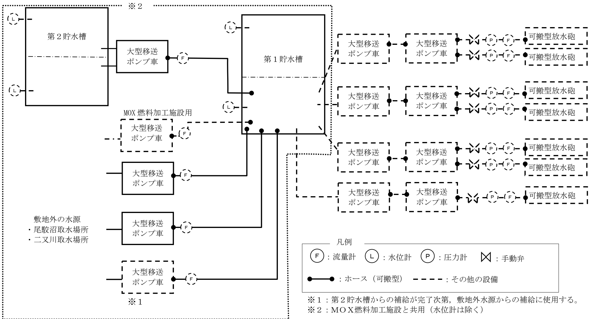
第9.4-4図 水供給設備の系統概要図 (大気中への放射性物質の放出抑制への対処に係る第1貯水槽への水の補給)
