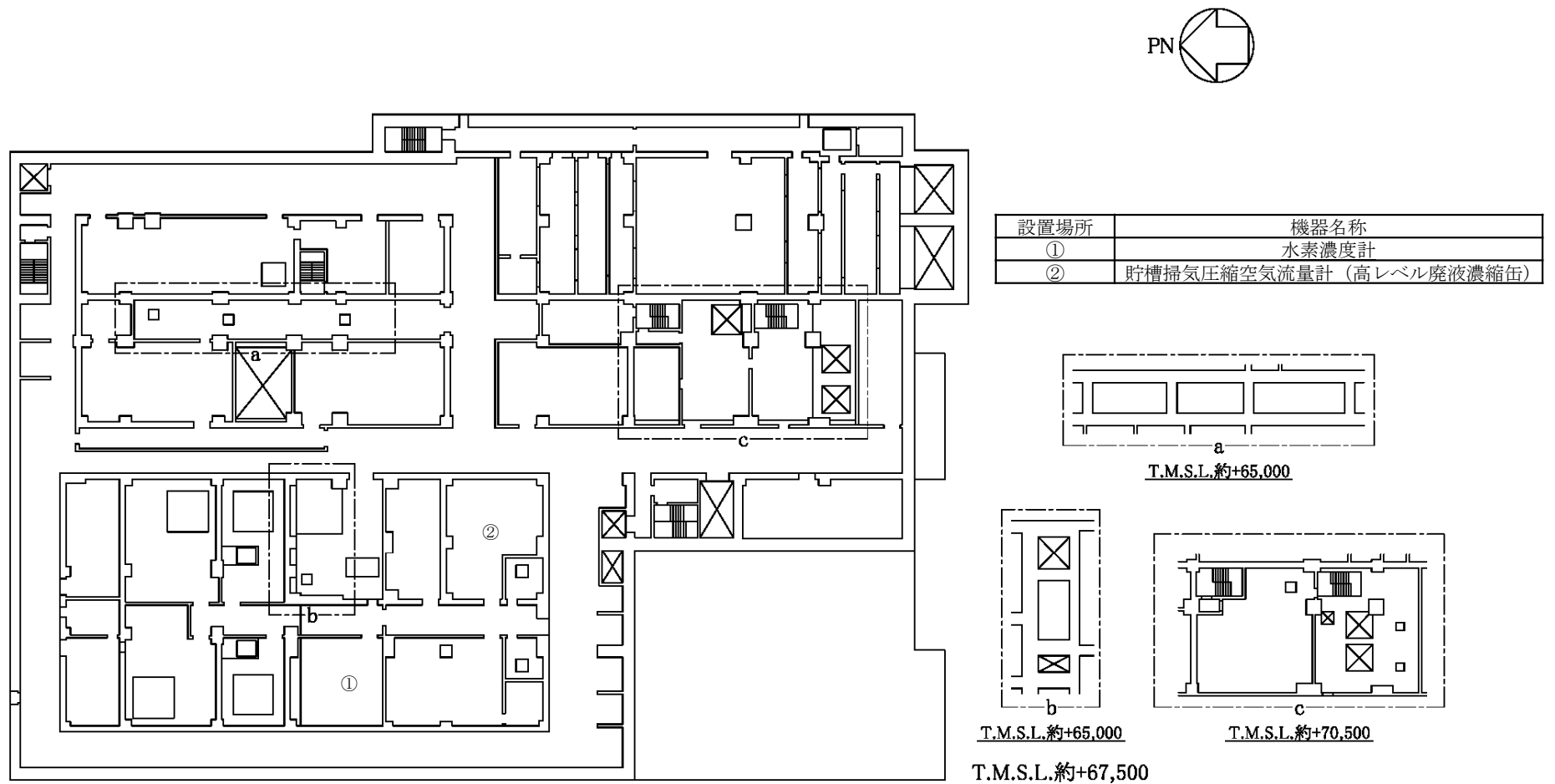
第6.2.1-54図 放射線分解により発生する水素による爆発に対処するために必要な計装設備の機器配置図（分離建屋 地上3階）
