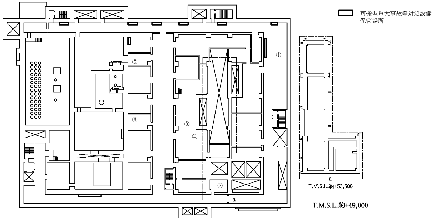
第6.2.1-69図 放射線分解により発生する水素による爆発に対処するために必要な計装設備の機器配置図 (高レベル廃液ガラス固化建屋 地下1階)
