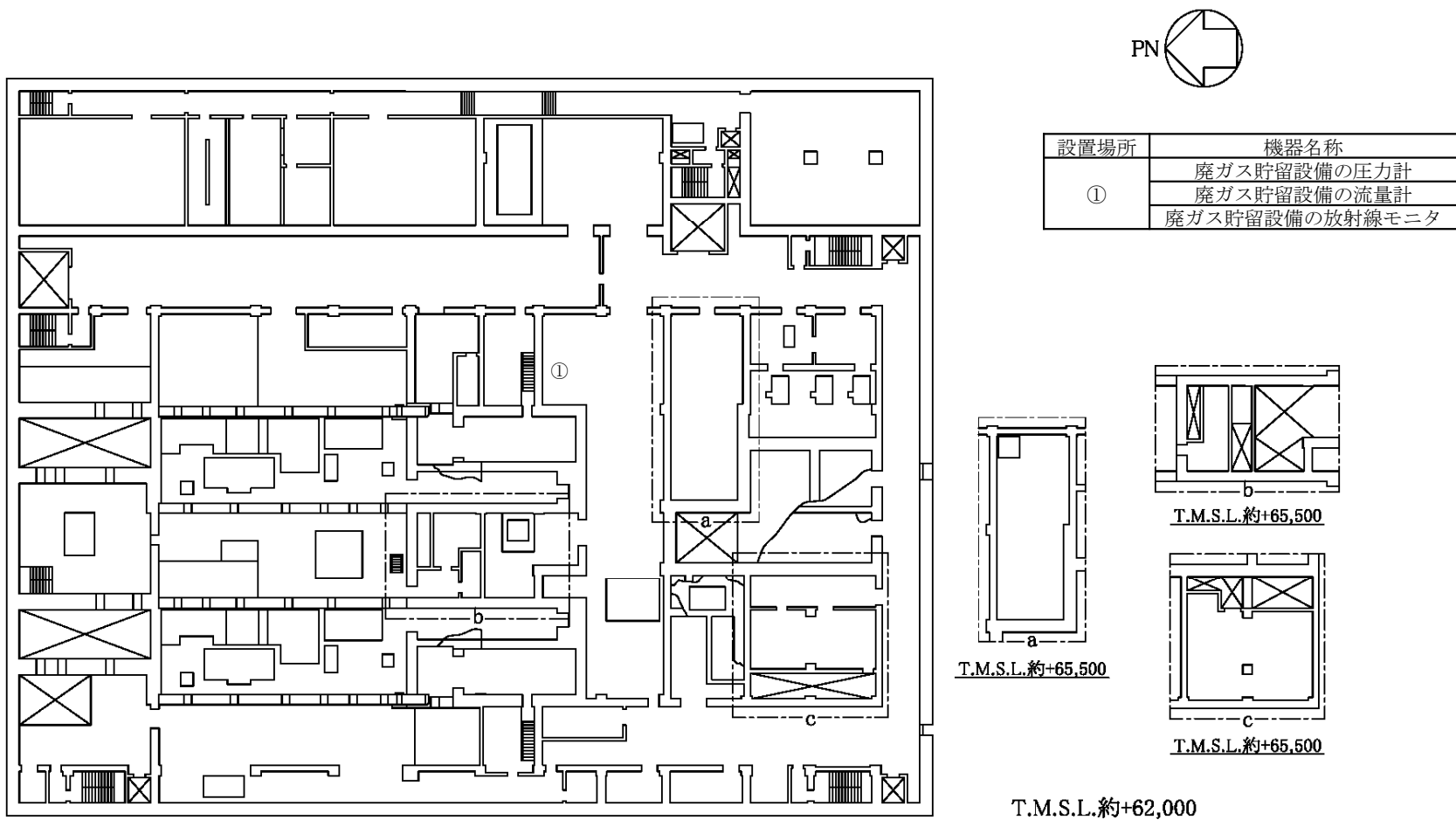
第6.2.1-8図 臨界事故の拡大を防止するために必要な計装設備の機器配置図（前処理建屋 地上2階）
