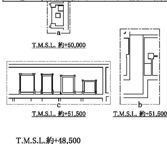
第6.2.1-58図 放射線分解により発生する水素による爆発に対処するために必要な計装設備の機器配置図 (精製建屋 地下1階)
