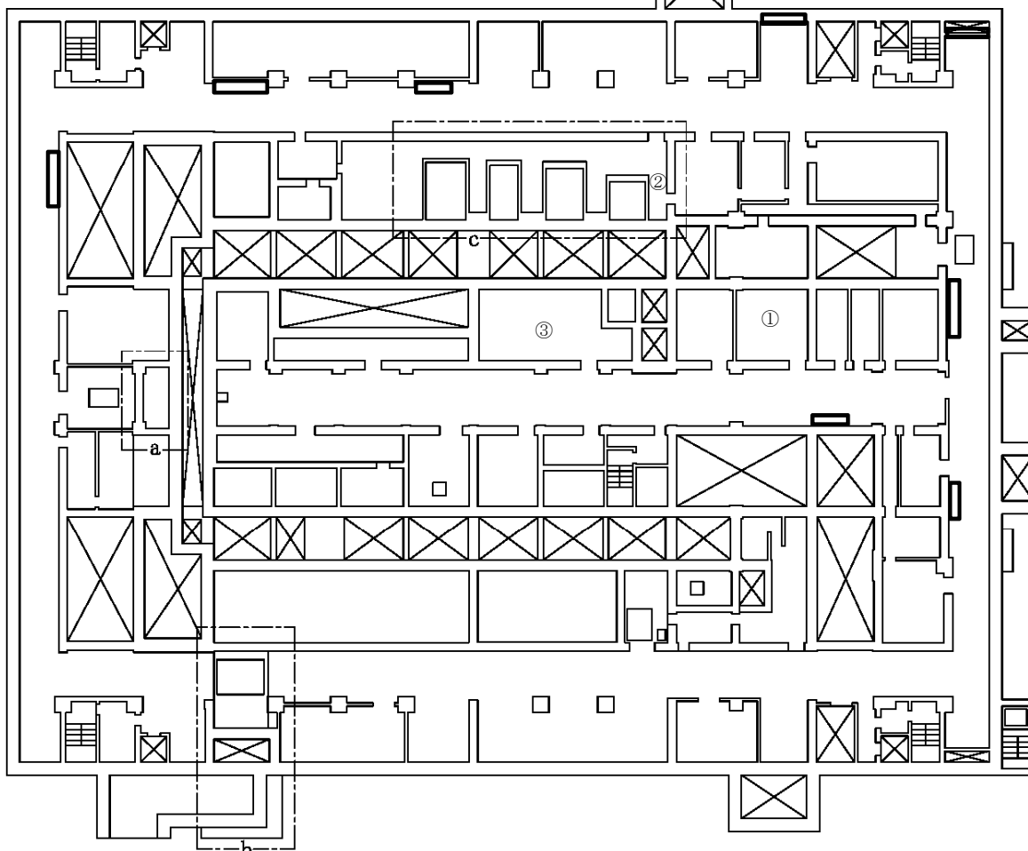
第6.2.1-58図 放射線分解により発生する水素による爆発に対処するために必要な計装設備の機器配置図 (精製建屋 地下1階)
