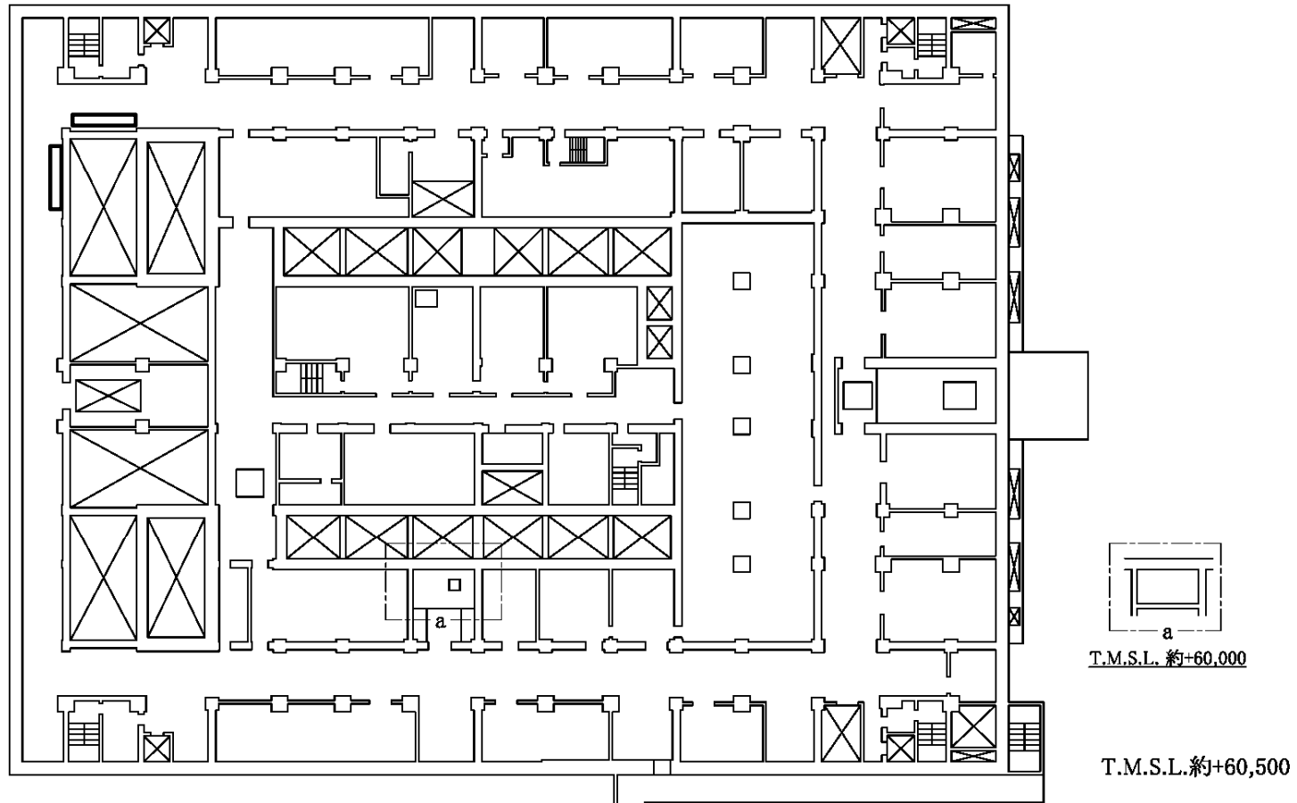
第6.2.1-60図 放射線分解により発生する水素による爆発に対処するために必要な計装設備の機器配置図（精製建屋 地上2階）
