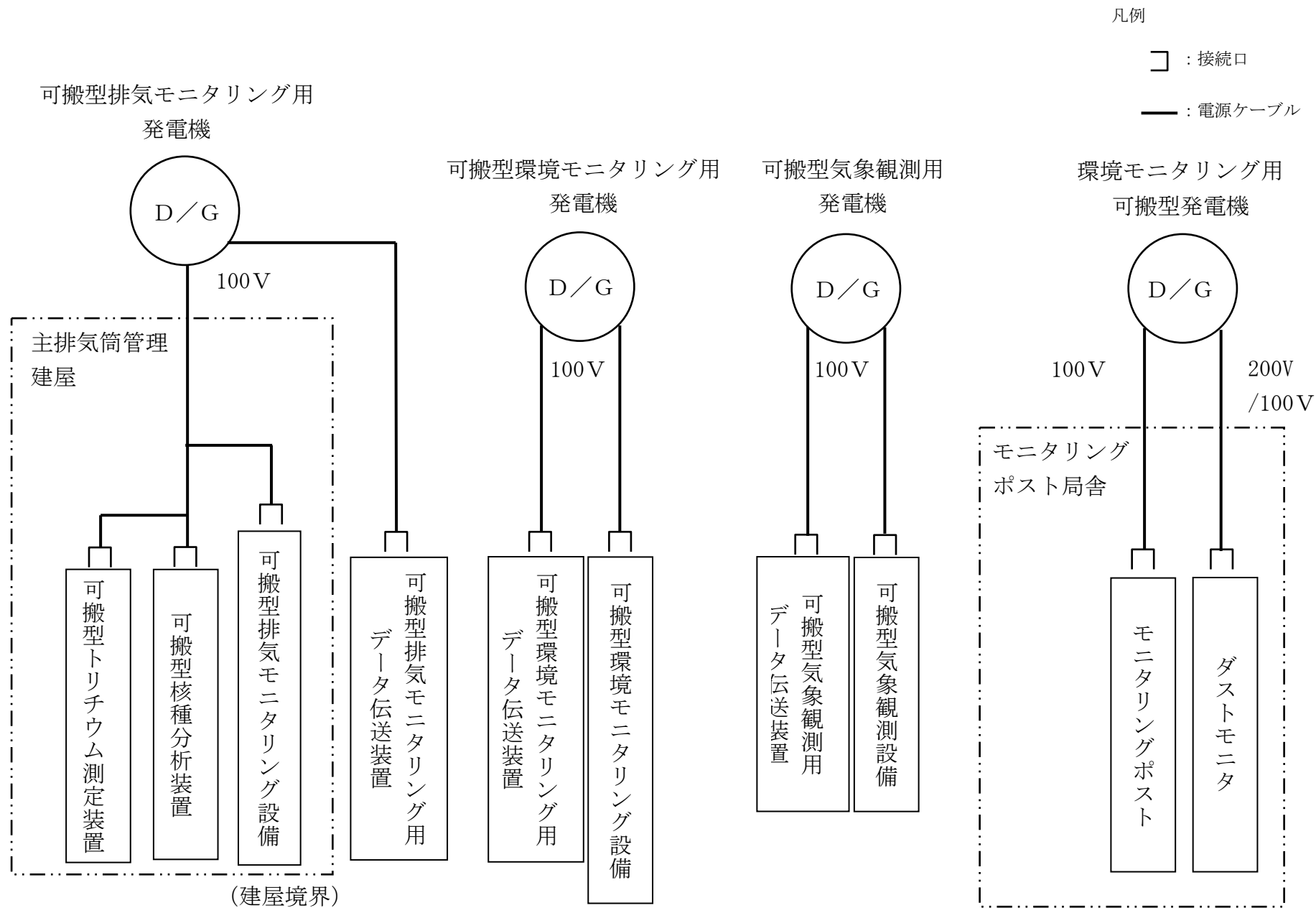
第 8.2-8 図 可搬型発電機接続時の系統図
