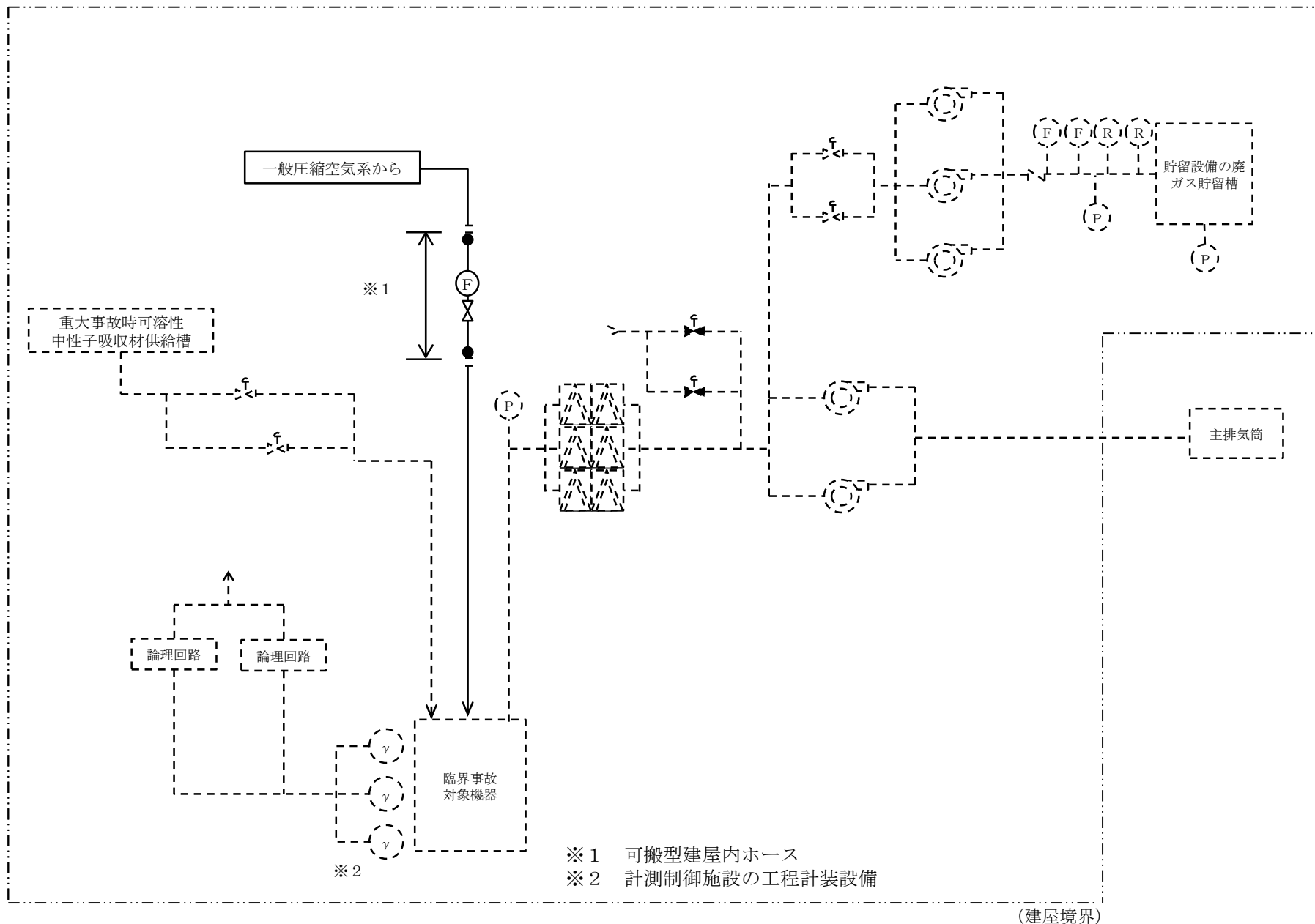
第34. 1 図 (その 6) その他再処理設備の附属施設の圧縮空気設備 臨界事故の拡大を防止するための設備の系統概要図 (臨界事故により発生する放射線分解水素の掃気に使用する設備)
