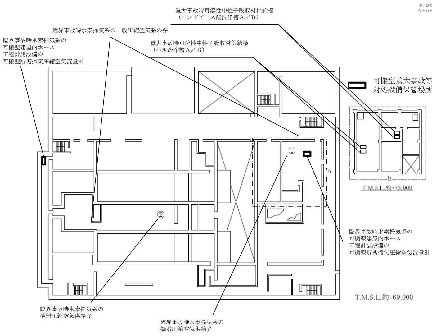
第34. 2 図 (その17) 前処理建屋 臨界事故の拡大防止対策の機器配置概要図 (地上3階) (放射線分解水素の掃気)
