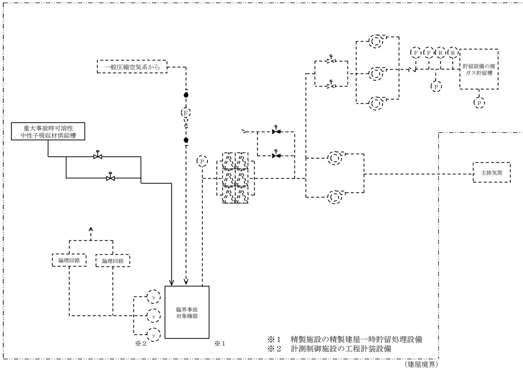
第4.3-8図 重大事故時可溶性中性子吸収材供給系の系統概要図
