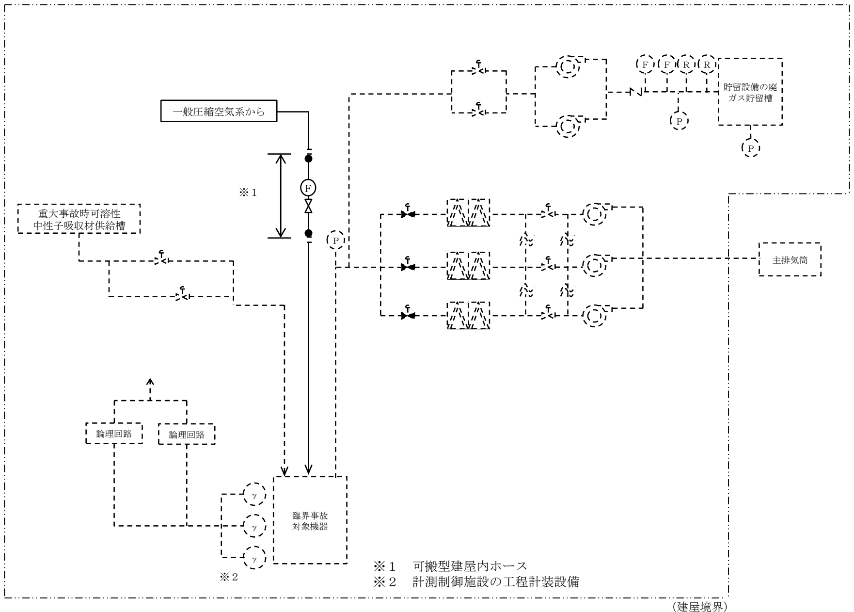
第34. 1 図 (その5) その他再処理設備の附属施設の圧縮空気設備 臨界事故の拡大を防止するための設備の系統概要図 (臨界事故により発生する放射線分解水素の掃気に使用する設備)
