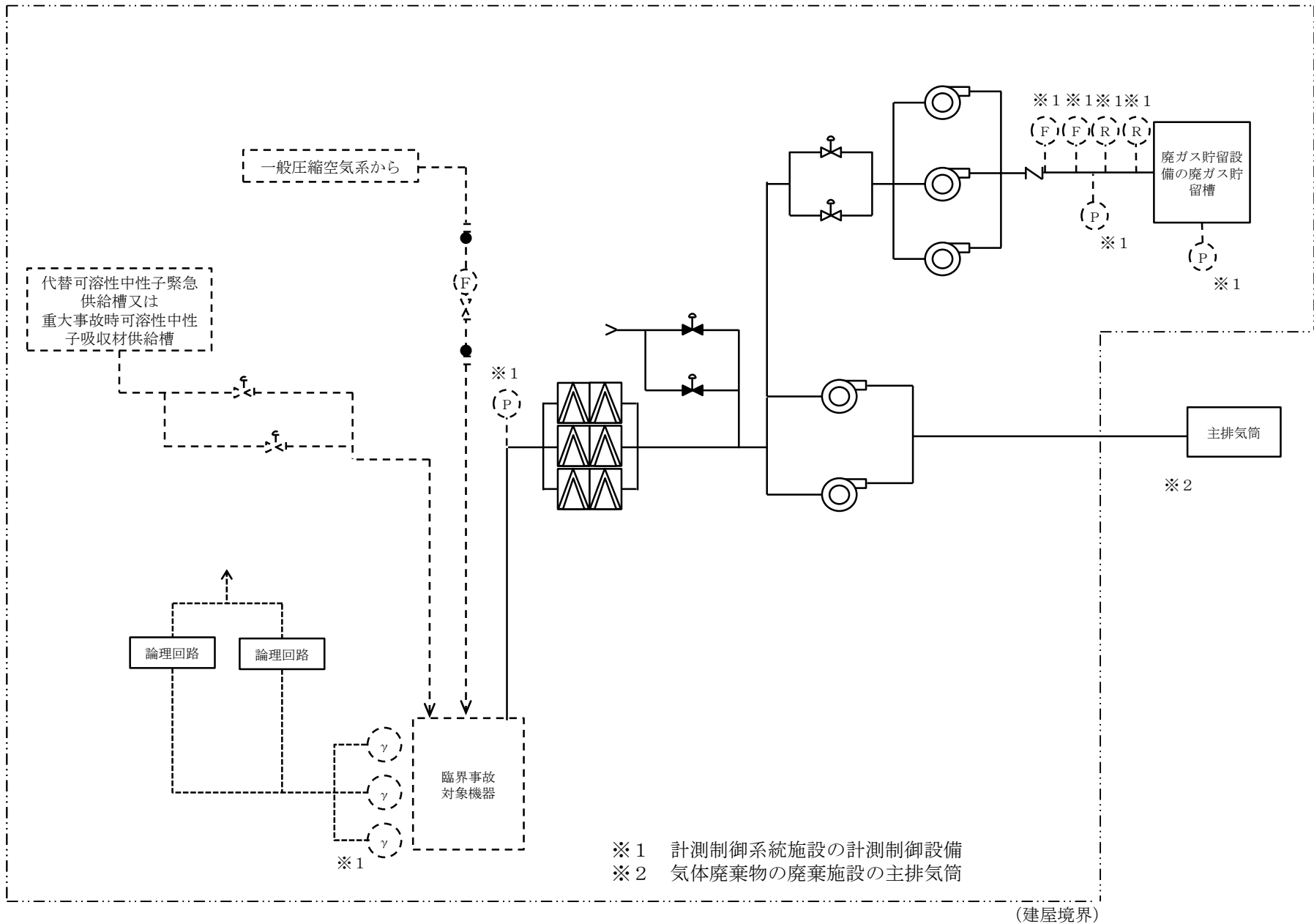
第7.2-38図 廃ガス貯留設備の系統概要図
