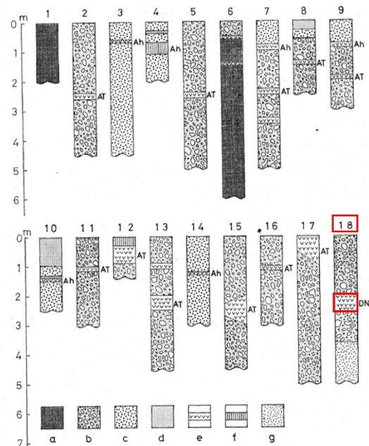
第5図 柱状図
