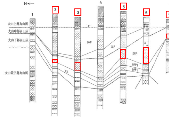
第3図 南北方向の柱状対比図。凡例は第4図。
