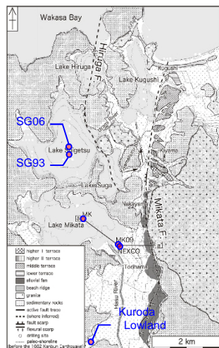
図2 三方五湖周辺の地形および断層帯分布
