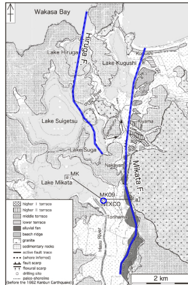
図2 三方湖周辺の地質および地形図。地質図は中井ほか(2002)、地形図の分布は岡田(1984)を一部修正。目録層帯は米野ほか(1989)および岡田・寛藤(2009)に従った。MK09、NEXCOコア、およびMKコア(竹村ほか,1994)の位置を示す。a-a'は図6の地形断面線を示す。
