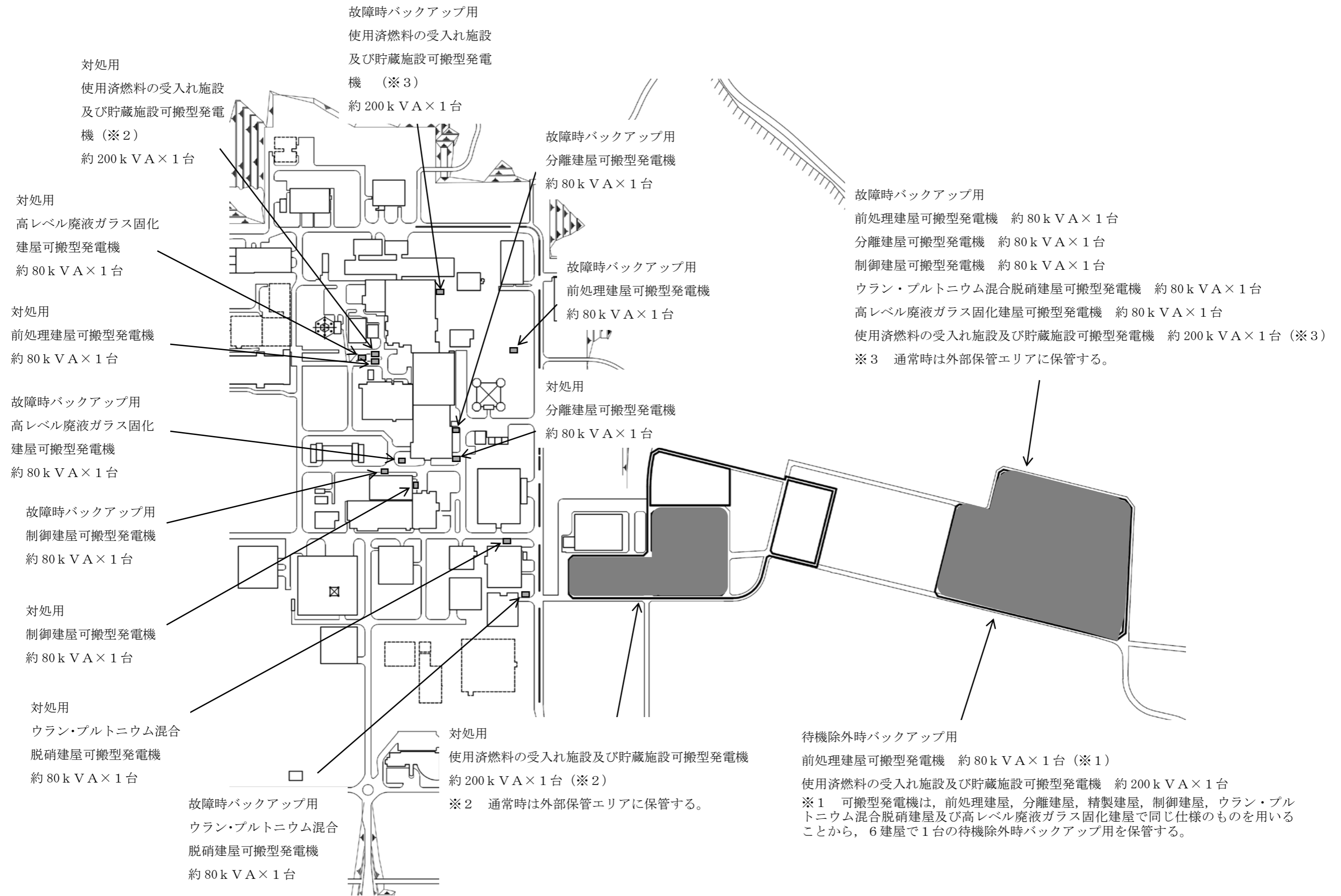
第9.2-8図 可搬型発電機の機器配置概要図
