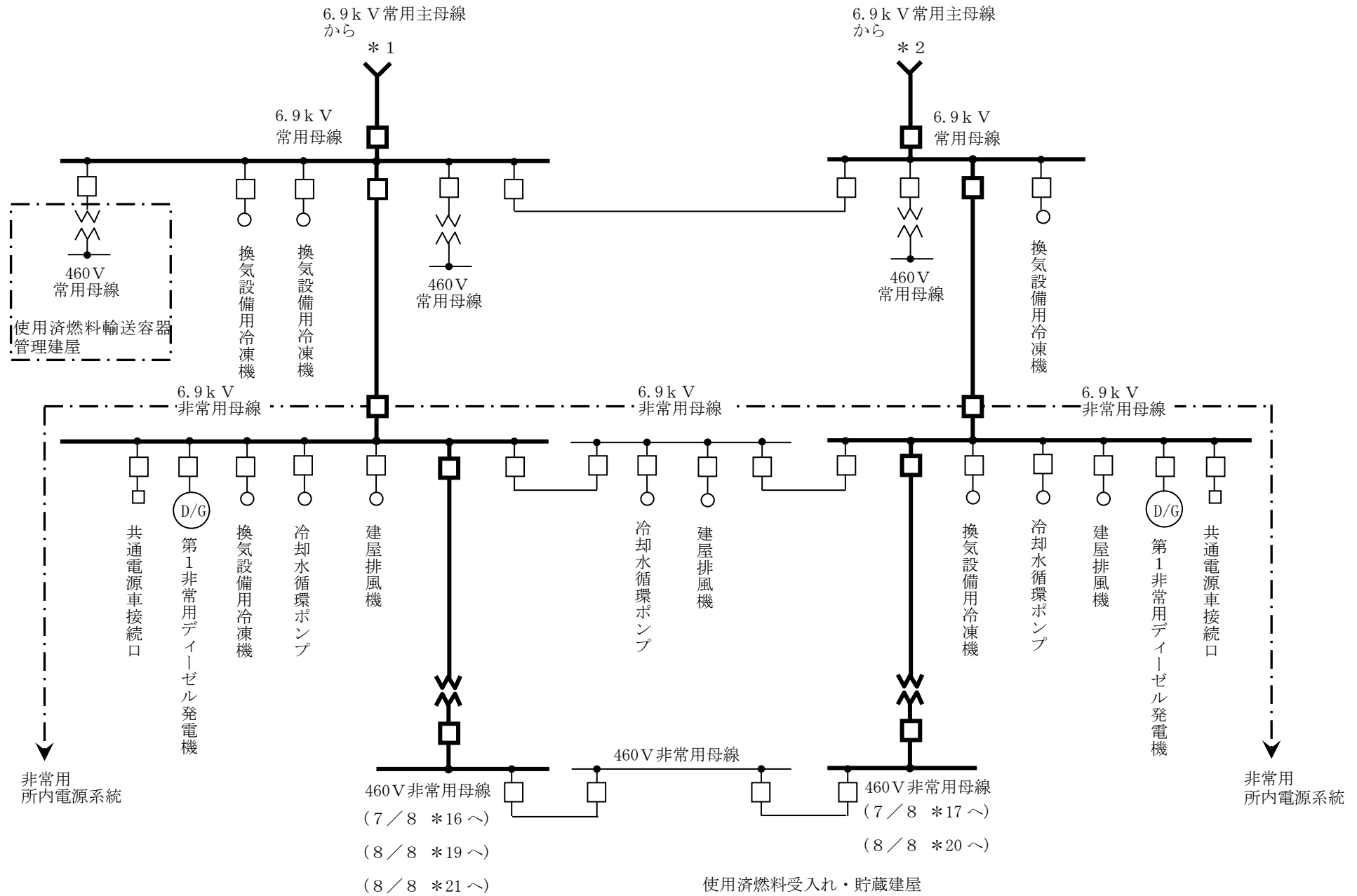
第 9.2-21(2) 図 全交流動力電源喪失を要因とせずに発生する重大事故等に対処するための設備の系統図(2/8)
