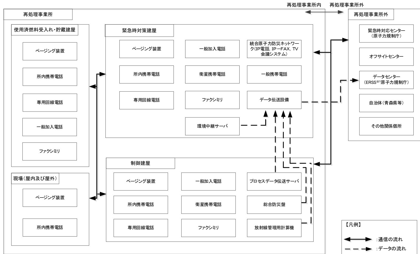
第 1.14-6 図 通信連絡設備の系統概要図
