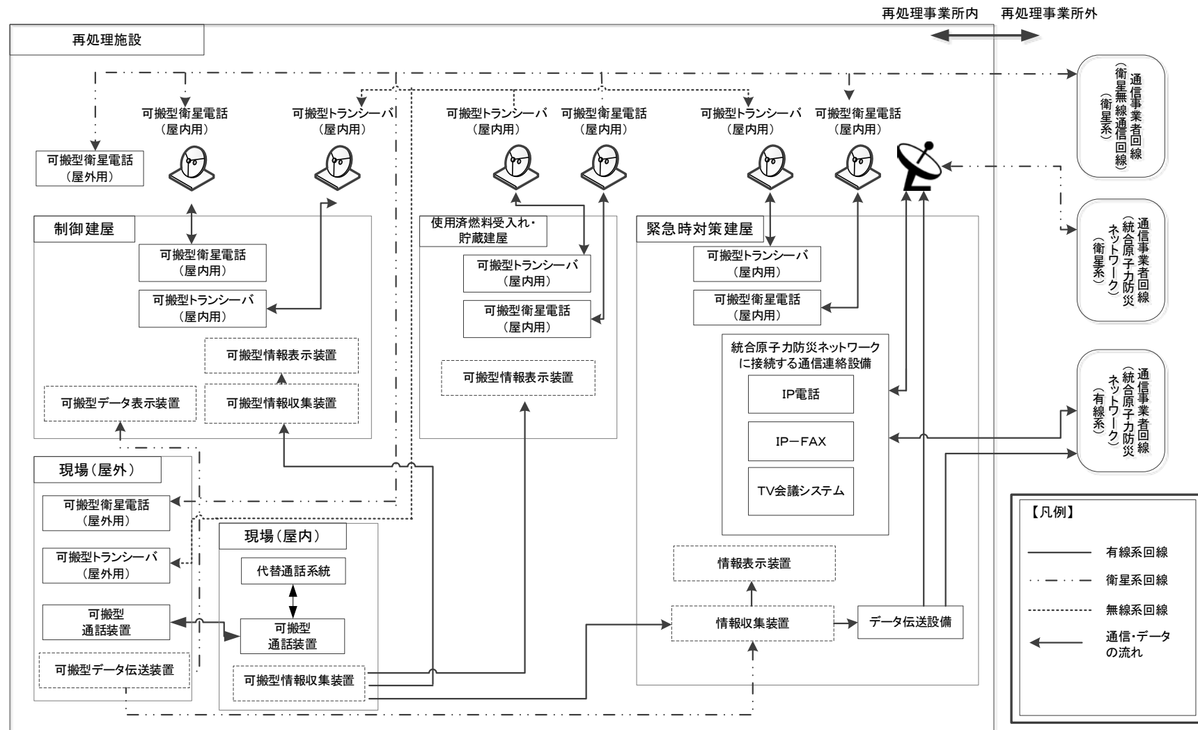
第 1.14-7 図 代替通信連絡設備の系統概要図
