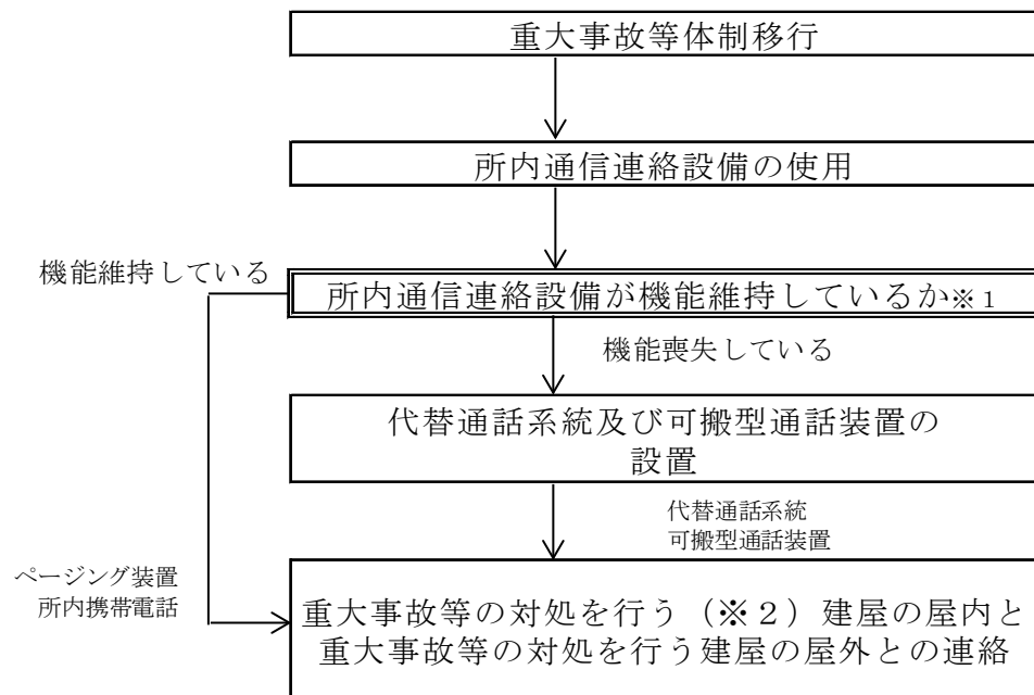
第1.14－1 図 屋内（現場）における再処理事業所内への通信連絡手順の概要
