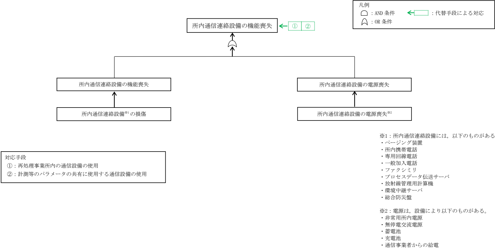
第 1.14-11 図 所内通信連絡設備における機能喪失原因対策分析
