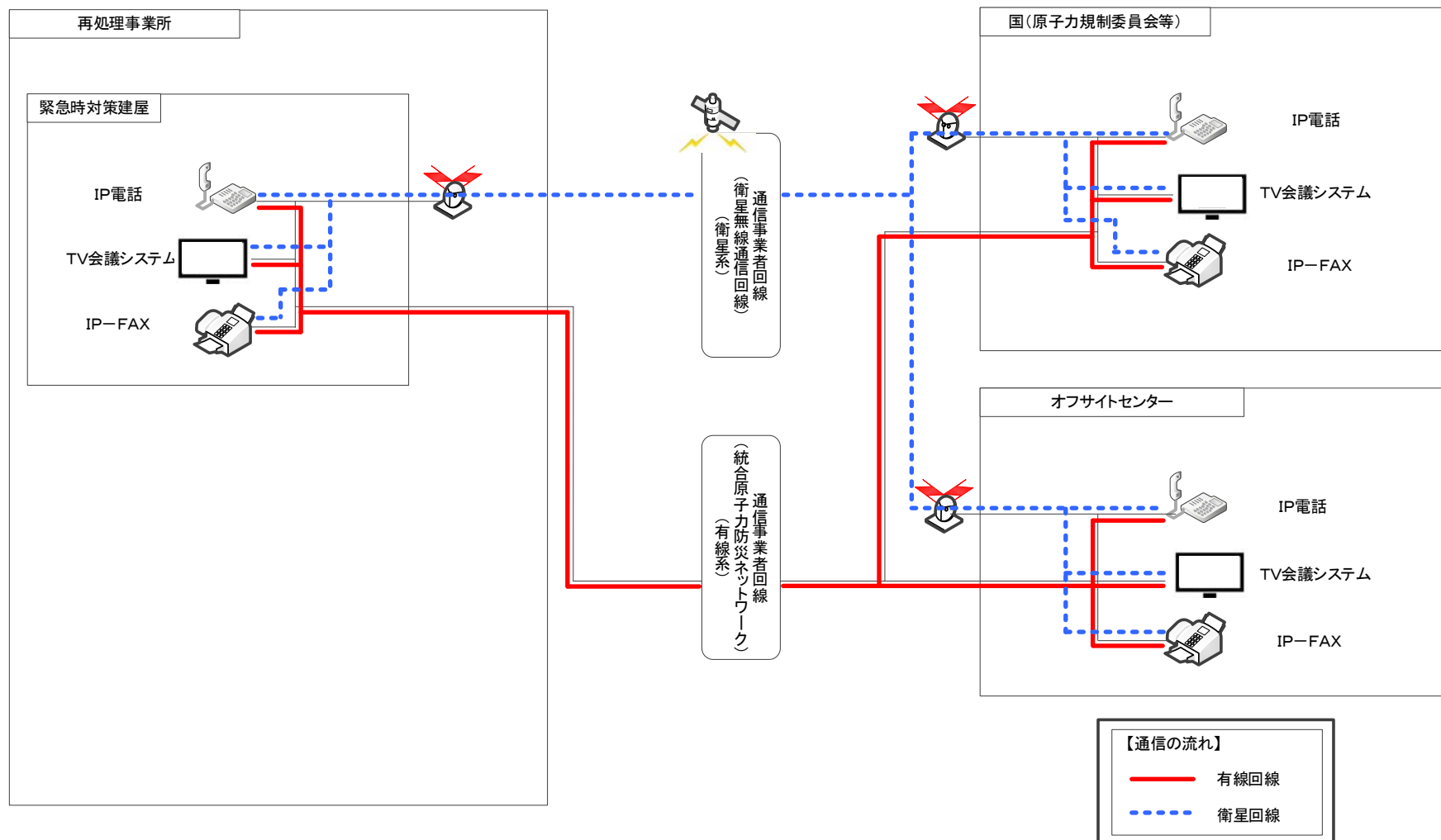
第 1.14.4-5 図 所外通信設備（再処理事業所外〔社外関係箇所〕）の概要（その 2） （統合原子力防災ネットワークに接続する通信連絡設備）
