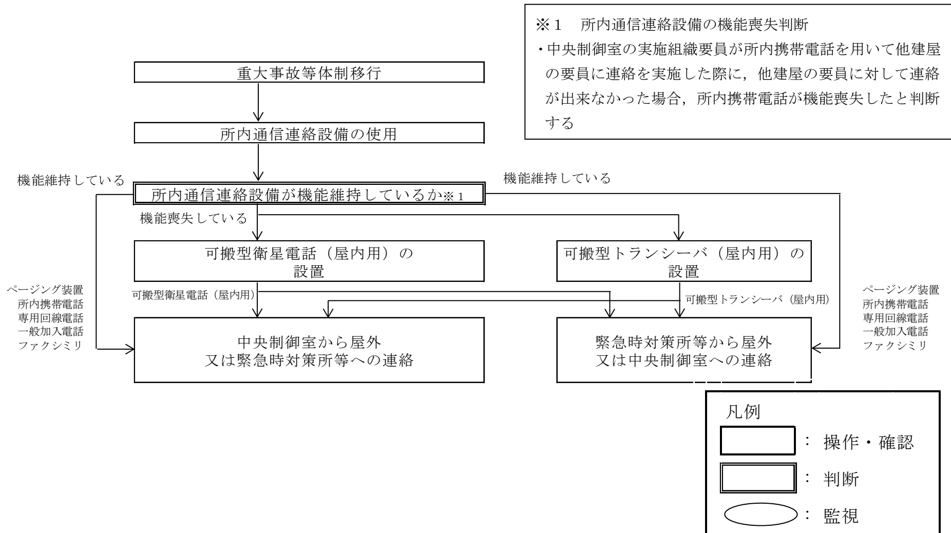
第1.14－3図 屋内（中央制御室及び緊急時対策所等）における再処理事業所内への通信連絡手順の概要
