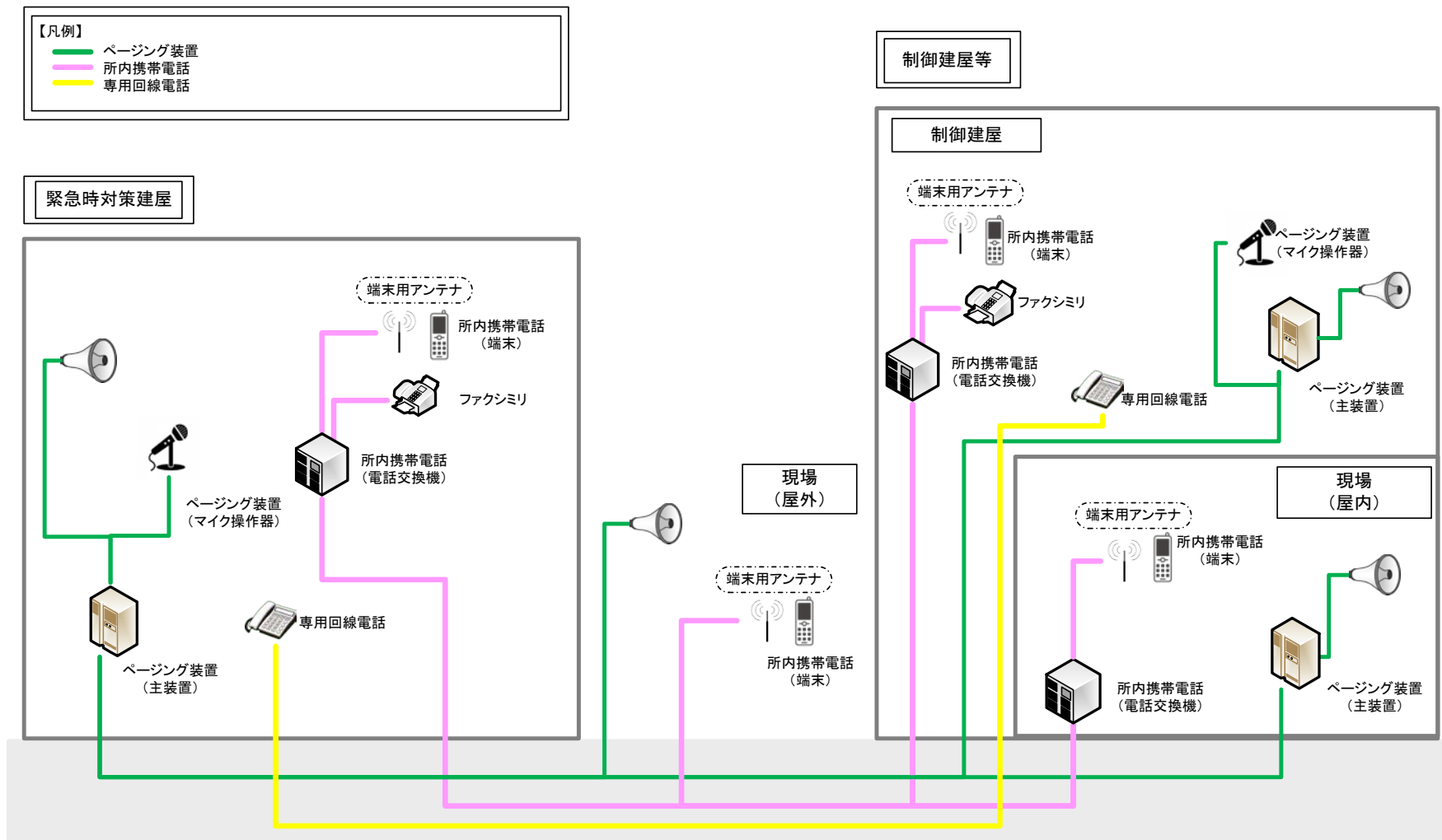
第 1.14.4-2 図 所内通信連絡設備の概要
