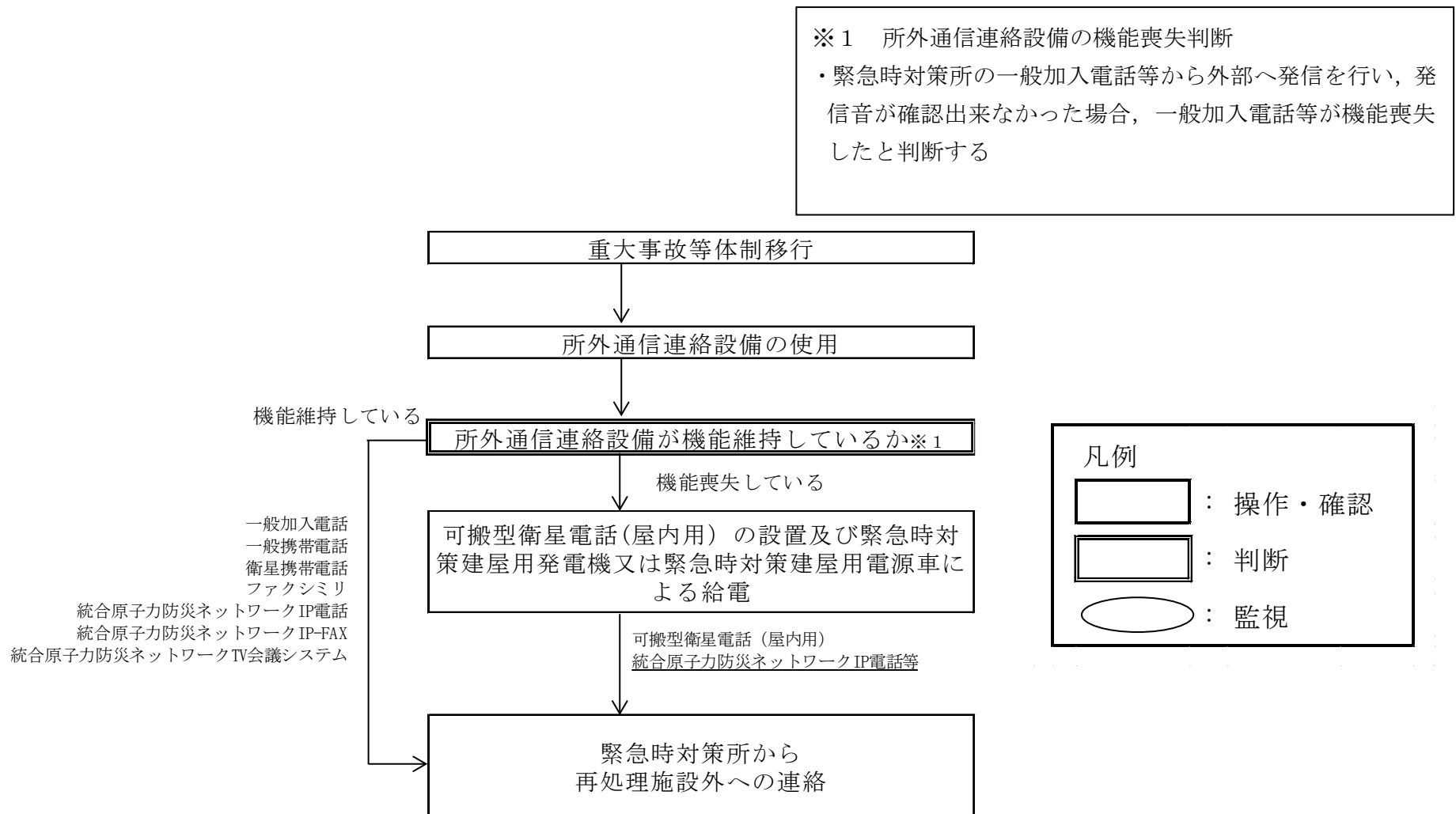
第1.14-5図 緊急時対策所における再処理事業所外への通信連絡手順の概要
