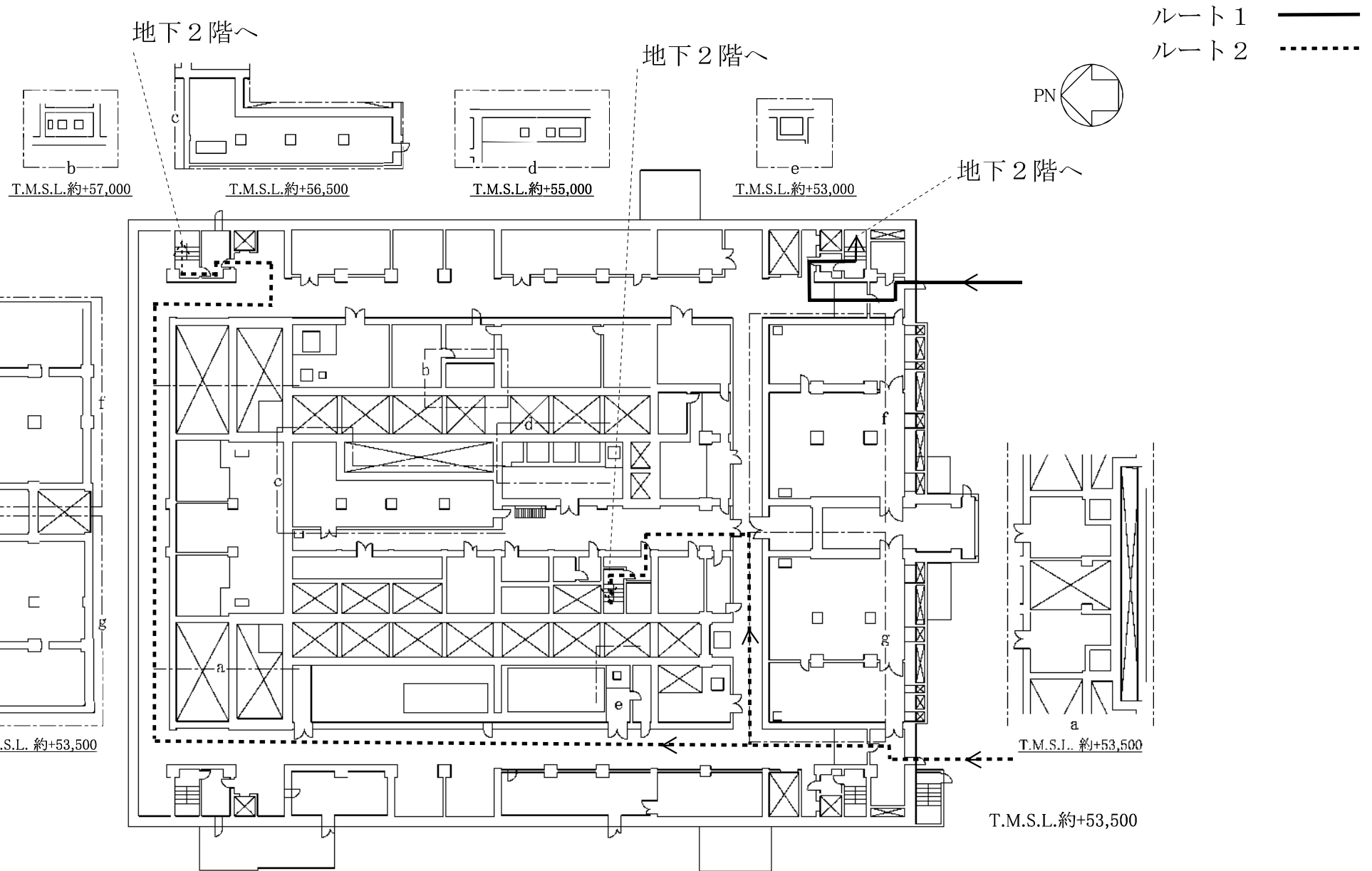
第1.0.1.2-1図 アクセスルート図 屋内 その5(1/3)
