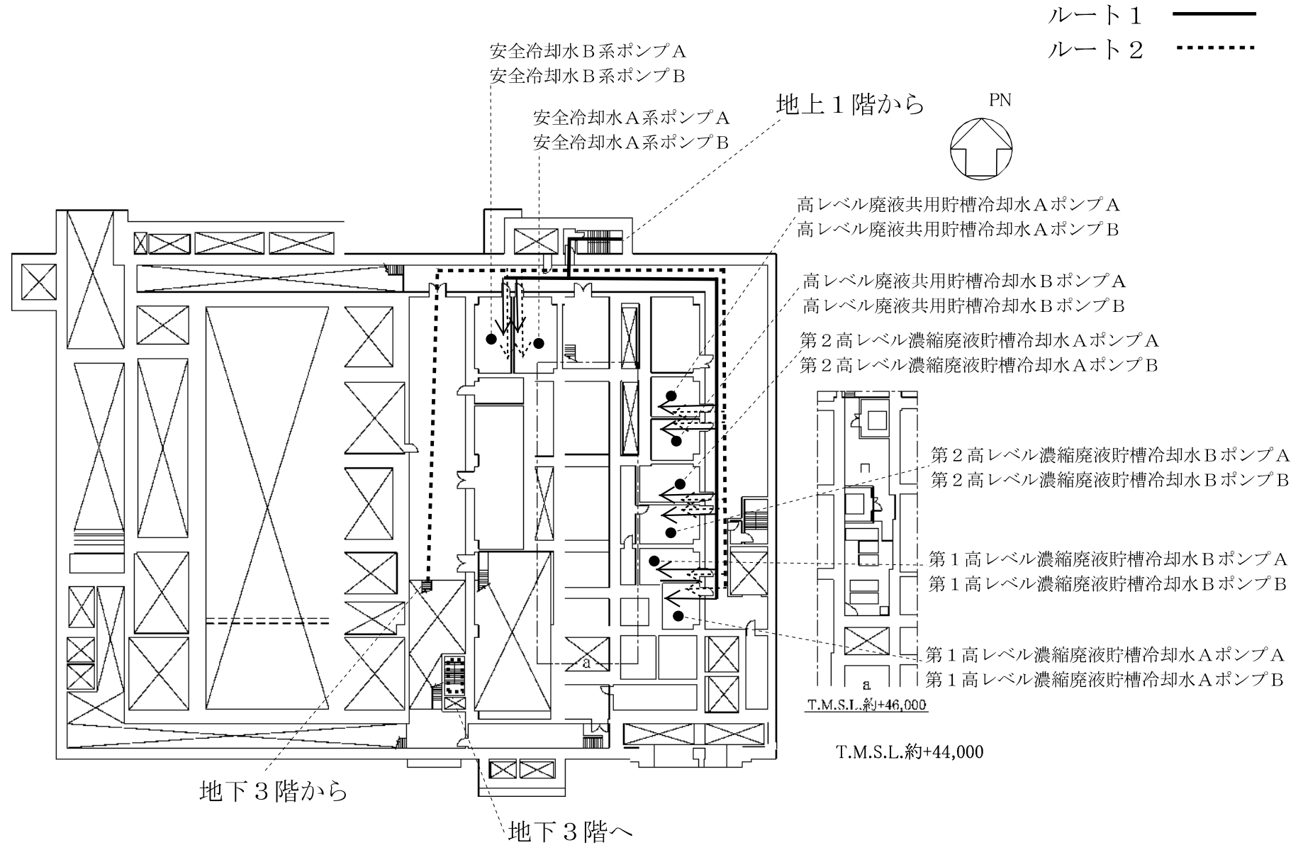
第1.0.1.2-1 図 アクセスルート図 屋内 その 7 (3/4)
