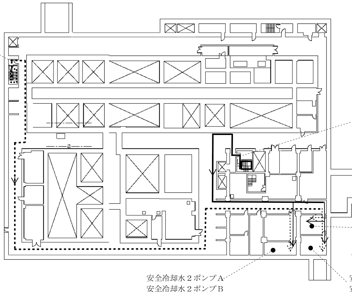
第1.0.1.2-1図 アクセスルート図 屋内 その4(3/4)
