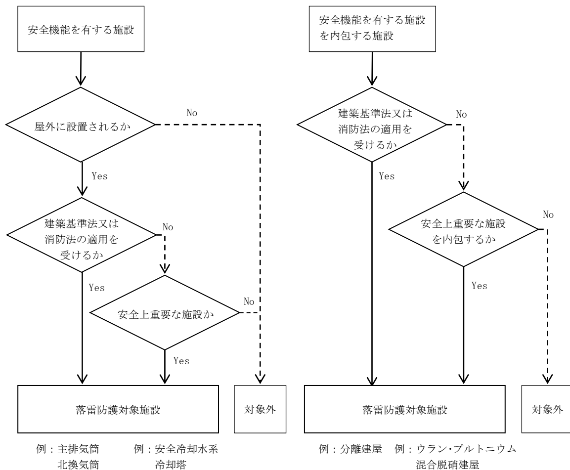
第４－１図 直撃雷に対する落雷防護対象施設の選定フロー
