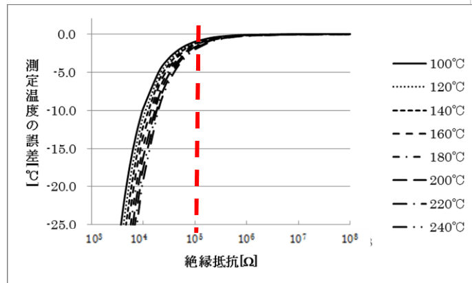
約 10^5 \Omega から計器誤差の懸念あり
