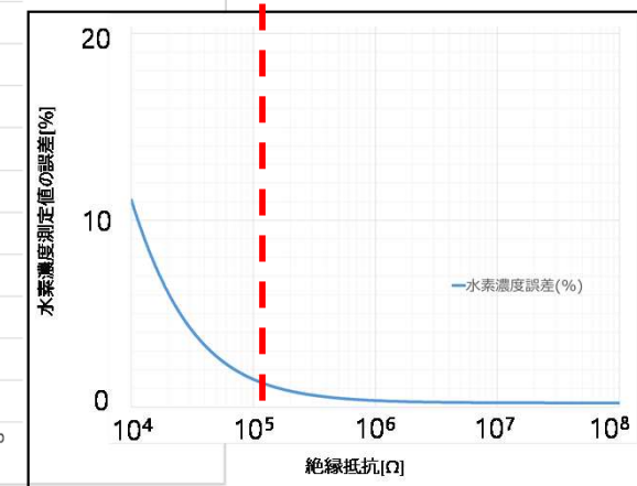
約 10^5 \Omega から計器誤差の懸念あり
