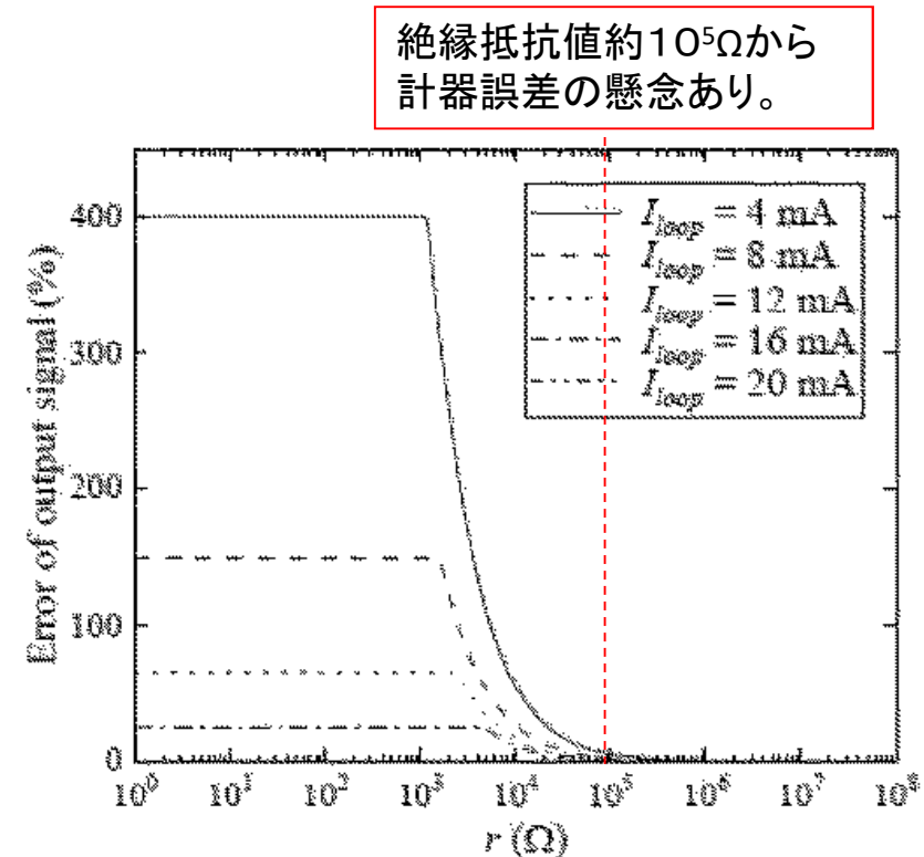
図5 伝送回路の絶縁抵抗と出力信号の誤差の関係 [4]
