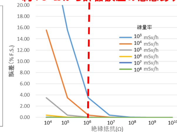
約 10^6 \Omega から計器誤差の懸念あり
