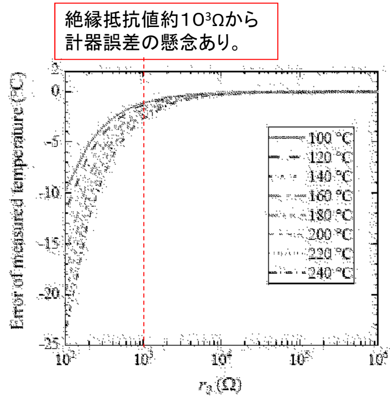
図4 熱電対回路の絶縁抵抗と測定温度の誤差の関係 [4]
