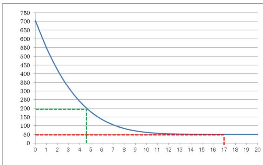
第2図 建屋外壁を対象とした熱影響評価結果
