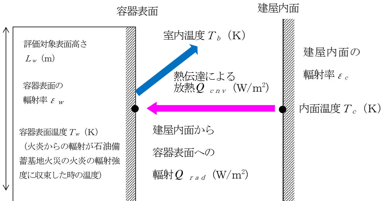
第2図 温度上昇の計算モデル (高压ガストレーラ庫)
