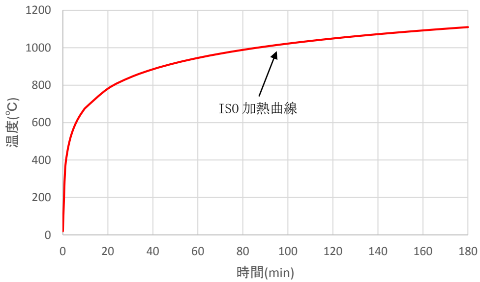
第1図 加熱曲線
