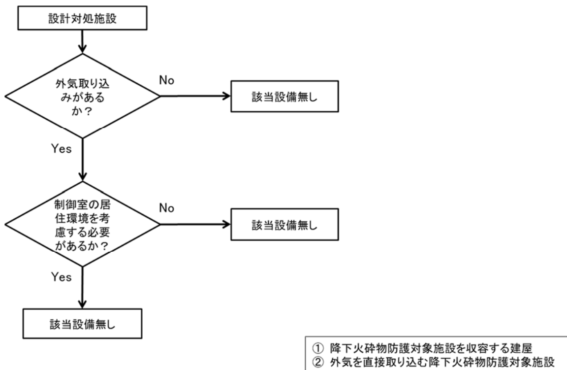
第 1 - 6 図 「大気汚染」に対し評価対象となる設計対処施設
