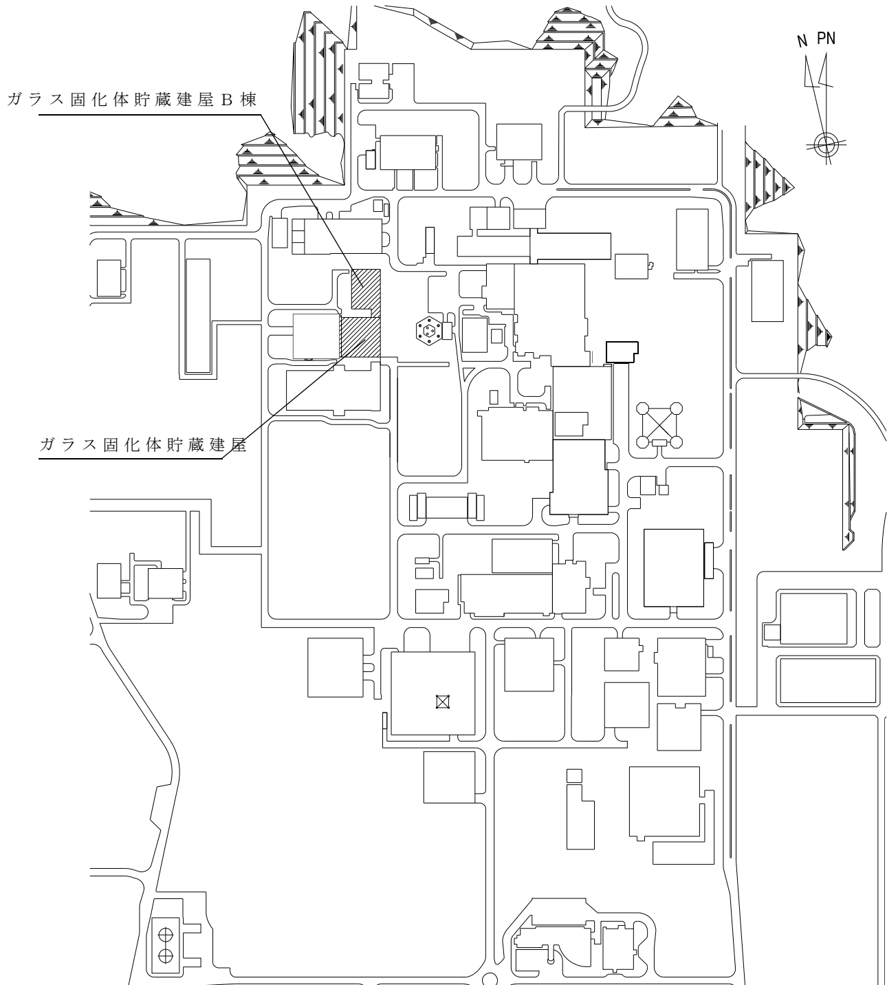
第 2.1 図 配置図
