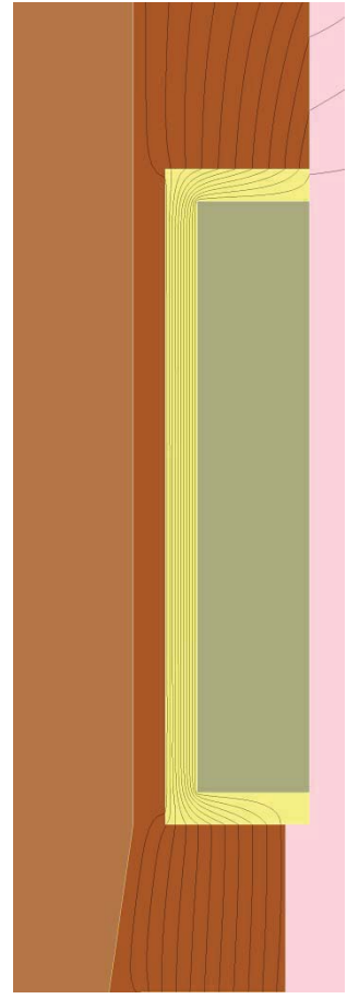
第 12 図 2 次元地下水浸透解析結果【2 号廃棄物埋設地 鉛直下方】(確からしい設定 1,000 年後) (2/5) <埋設設備 1 の流出点を通る流跡線>
