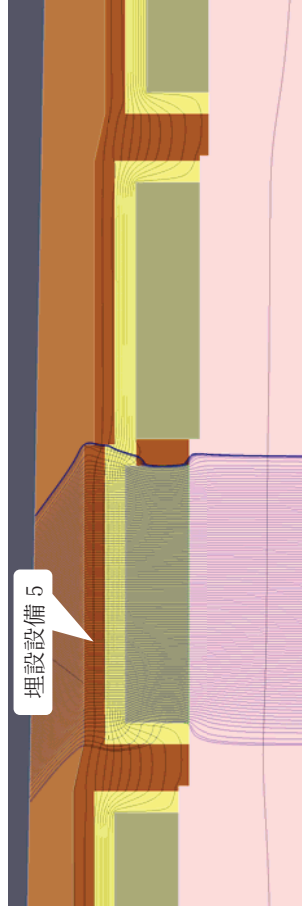
第 10 図 2 次元地下水浸透流解析結果【1 号廃棄物埋設地 鉛直下方】(確からしい設定 1,000 年後) (6/9) <埋設設備 5 の流出点を通る流跡線>
