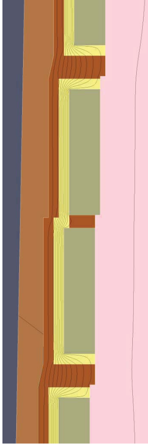
第 10 図 2 次元地下水浸透解析結果【1 号廃棄物埋設地 鉛直下方】(確からしい設定 1,000 年後) (1/9) <0.1m 間隔全水頭等高線>
