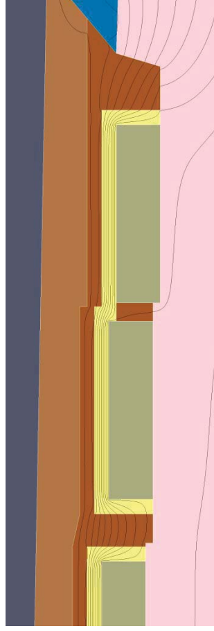
第 10 図 2 次元地下水浸透流解析結果【1号廃棄物埋設地 鉛直下方】(確からしい設定 1,000 年後) (3/9) <埋設設備 2 の流出点を通る流跡線>
