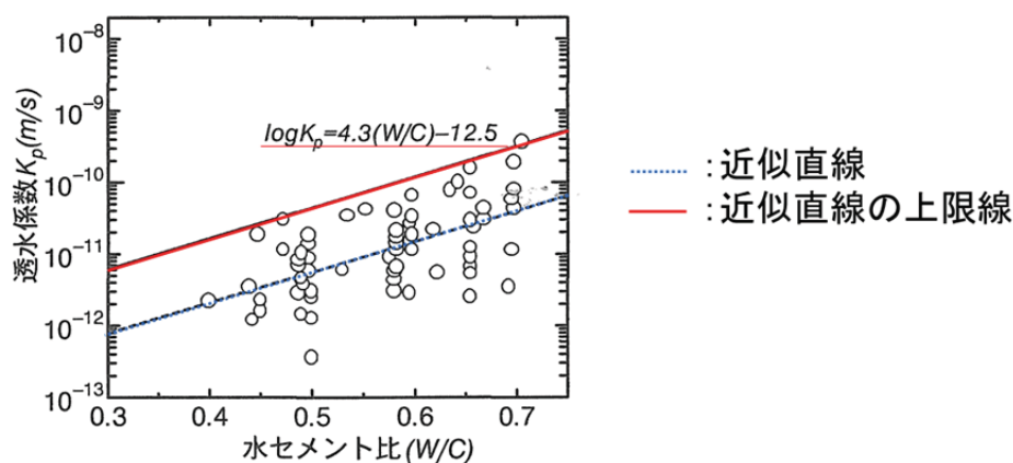
第1図 水セメント比と透水係数の関係
