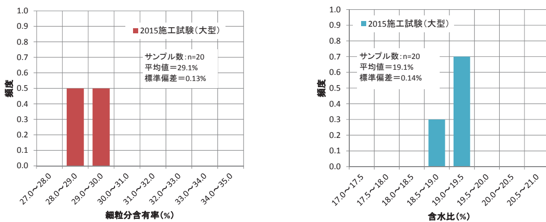
第4図 混合土の製造確認結果：大型施工機械分
