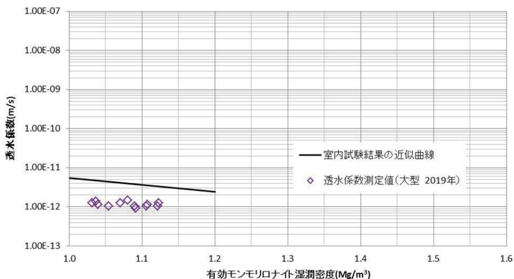
第6図 有効モンモリロナイト湿潤密度と透水係数の関係 (現地施工試験結果プロット、Na型ベントナイト混合土)
