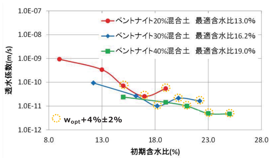
第3図 ベントナイト混合率ごとの含水比と透水係数の関係
