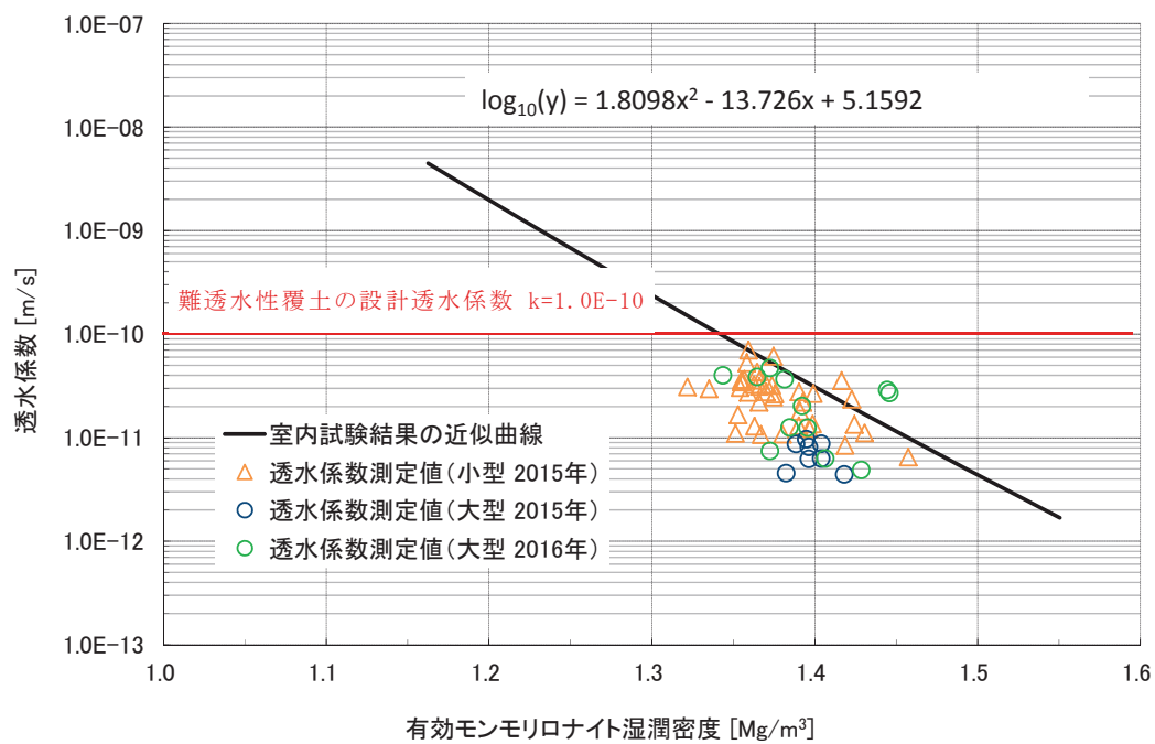
第5図 有効モンモリロナイト湿潤密度と透水係数の関係 (現地施工試験結果プロット、Ca型ベントナイト混合土)
