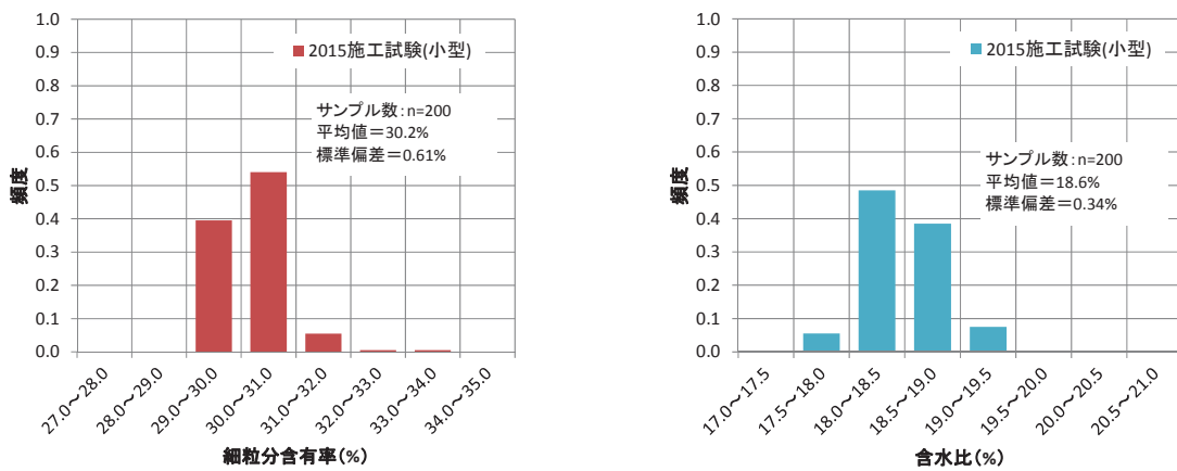
第3図 混合土の製造確認結果：小型施工機械分
