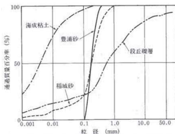
第4図 代表的な土の粒形加積曲線の例 (地盤工学会、地盤材料試験の方法と解説)
