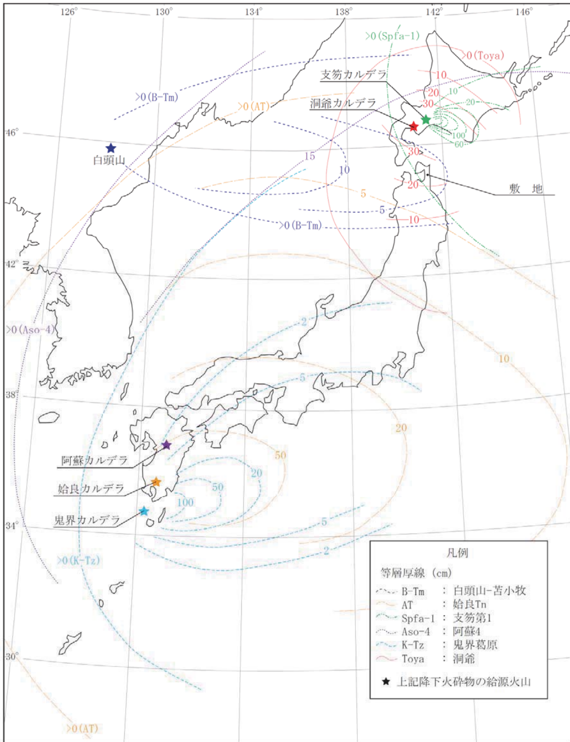
第13図 地理的領域外の第四紀火山起源の主な降下火砕物の分布
