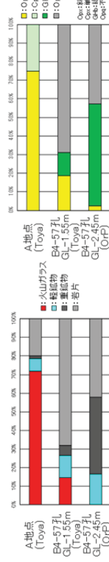
全鉱物組成分析結果
