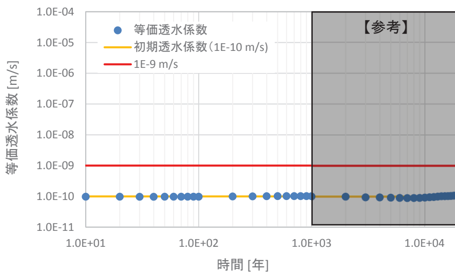
第 5 図 3号廃棄物埋設施設のうち難透水性覆土におけるの等価透水係数の時間変化の結果
