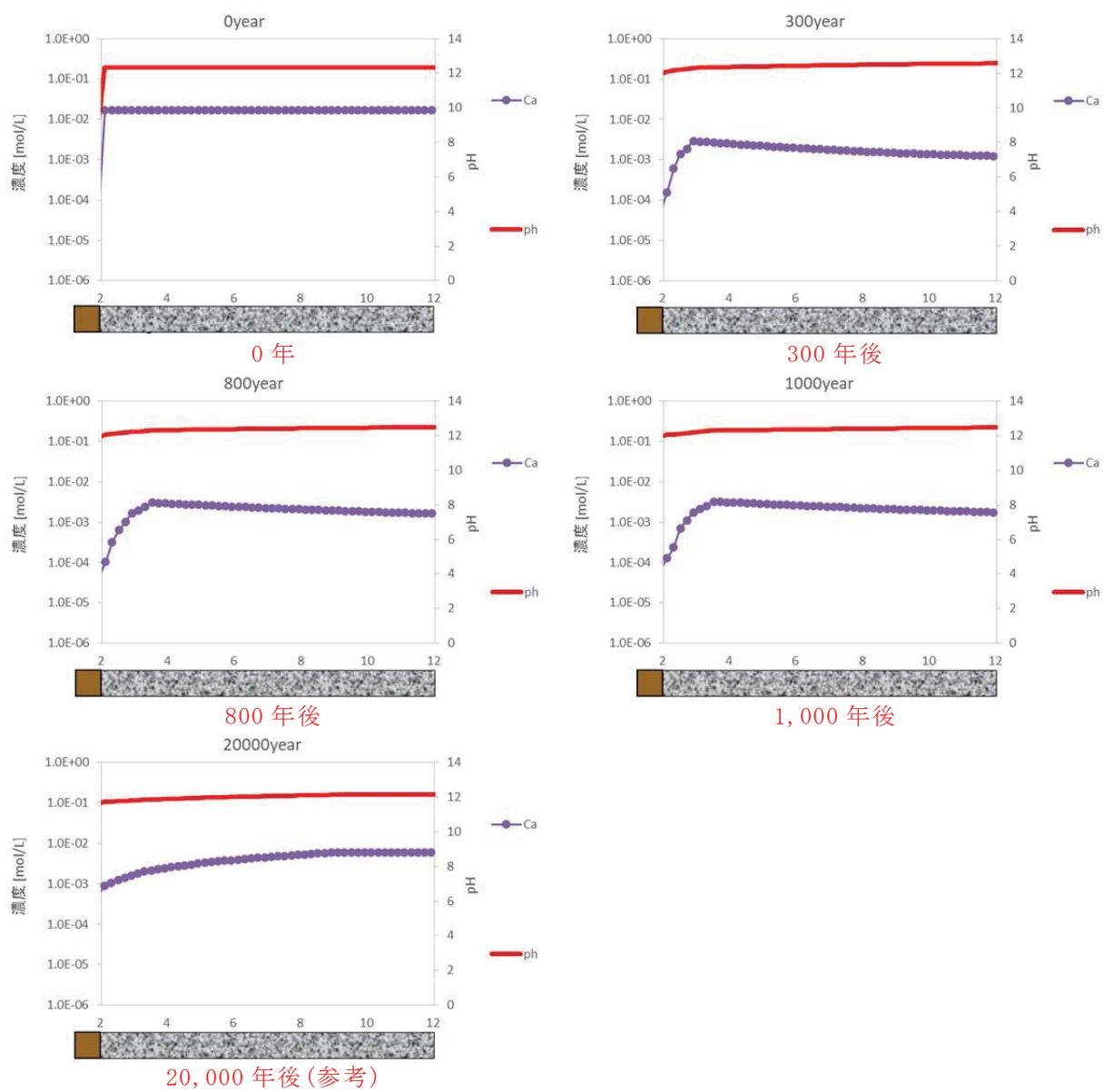
第 13 図 3 号廃棄物埋設施の埋設設備内の液相組成 (pH、Ca 濃度) の分布図 (ケース②)：難透水性覆土の拡散を単純なモデルとした場合)
