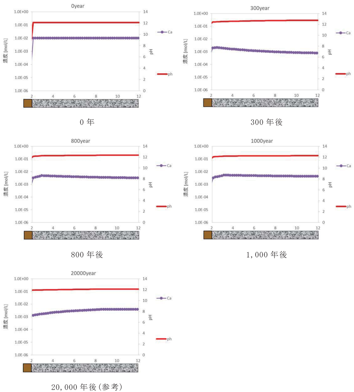
第 12 図 1 号廃棄物埋設施設のうち埋設設備内の液相組成(pH、Ca 濃度)の分布図 (ケース①：難透水性覆土の拡散を現実的なモデルとした場合)
