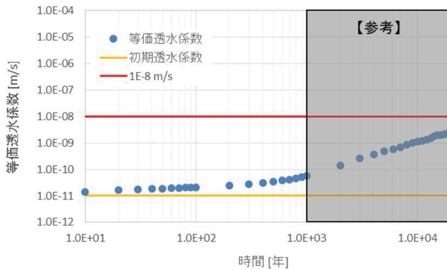
第 10 図 1号廃棄物埋設施設の難透水性覆土(Na型)における等価透水係数の時間変化の結果(ケース②：難透水性覆土の拡散を単純なモデルとした場合)
