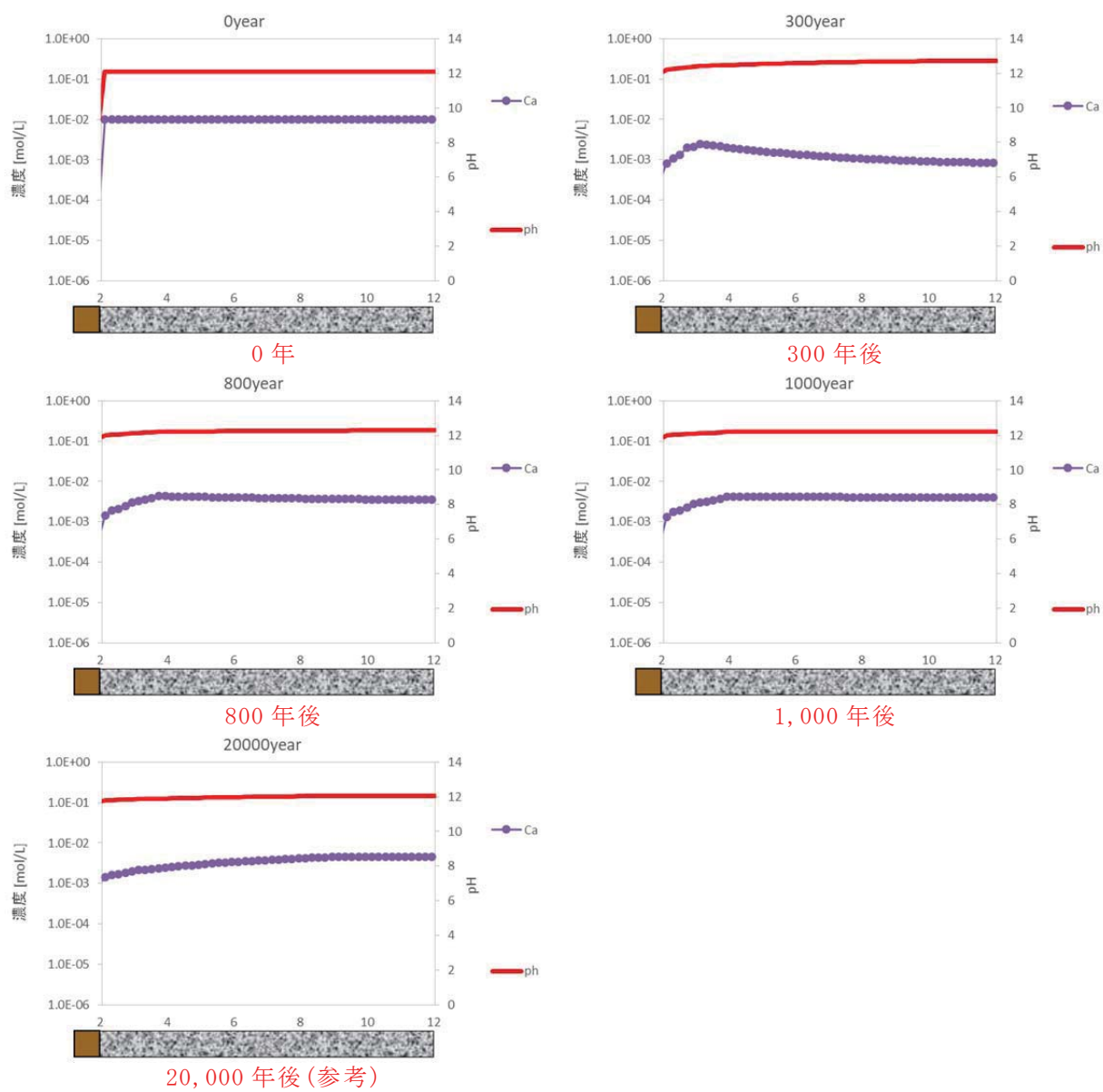
第 16 図 1 号廃棄物埋設施の埋設設備内の液相組成 (pH、Ca 濃度) の分布図 (ケース②)：難透水性覆土の拡散を単純なモデルとした場合)
