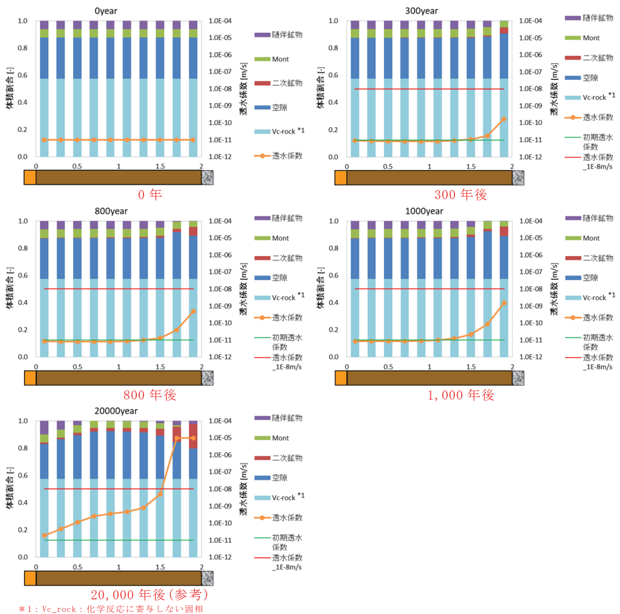
第11図 3号廃棄物埋設施設の難透水性覆土(Na型)における鉱物組成と透水係数の分布図 (ケース②: 難透水性覆土の拡散を単純なモデルとした場合)
