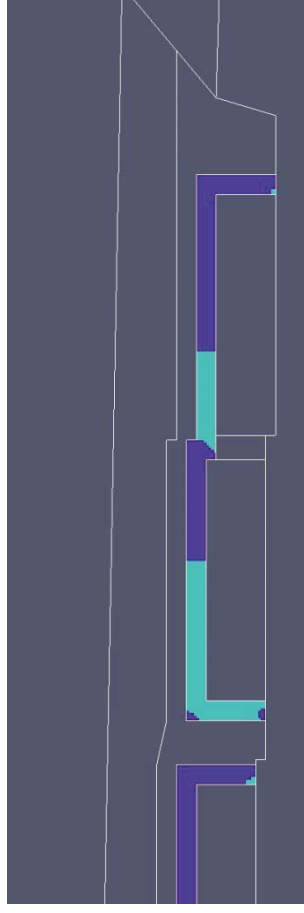
図 難透水性覆土内のペクレ数 ( P_e ) 分布 (4/6) 【1 号廃棄物埋設地】 (厳しい設定 1, 000 年後)
