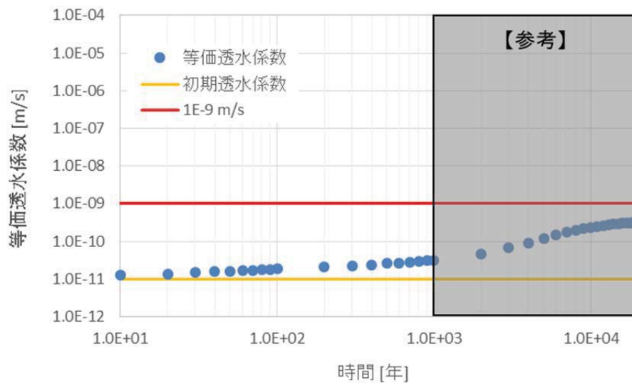
第 2 図 1号廃棄物埋設施設の難透水性覆土(Na型)における等価透水係数の時間変化の結果(ケース①：難透水性覆土の拡散を現実的なモデルとした場合)
