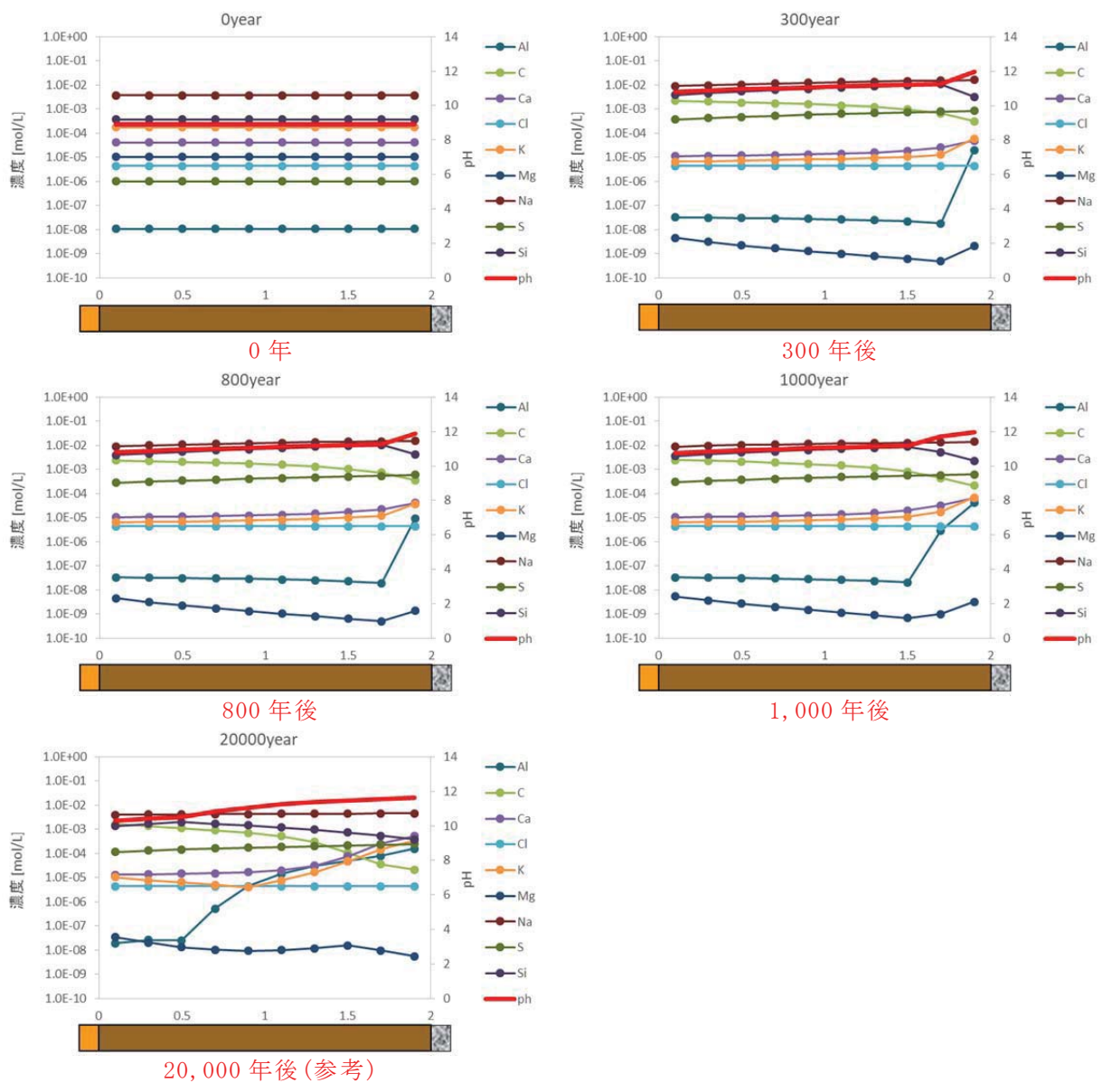
第 12 図 3 号廃棄物埋設施の難透水性覆土 (Na 型) における液相組成の分布図 (ケース②)：難透水性覆土の拡散を単純なモデルとした場合)
