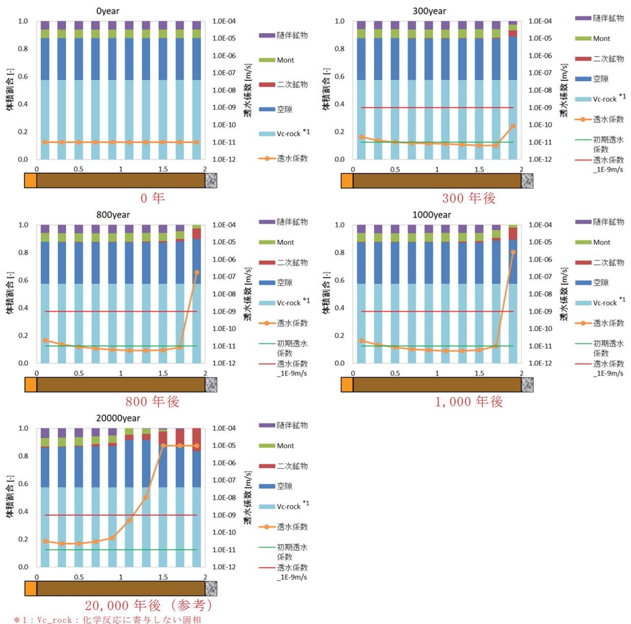
第3図 3号廃棄物埋設施の難透水性覆土(Na型)における鉱物組成と透水係数の分布図 (ケース①: 難透水性覆土の拡散を現実的なモデルとした場合)
