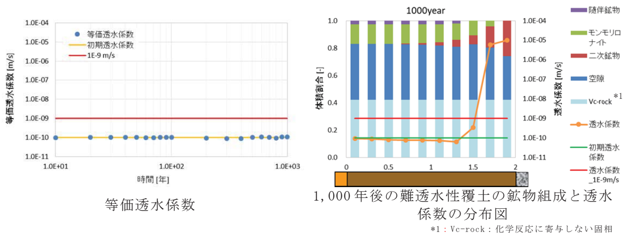
第 10 図 3号廃棄物埋設施設の解析結果(セメント系材料の仕様: OPC)
