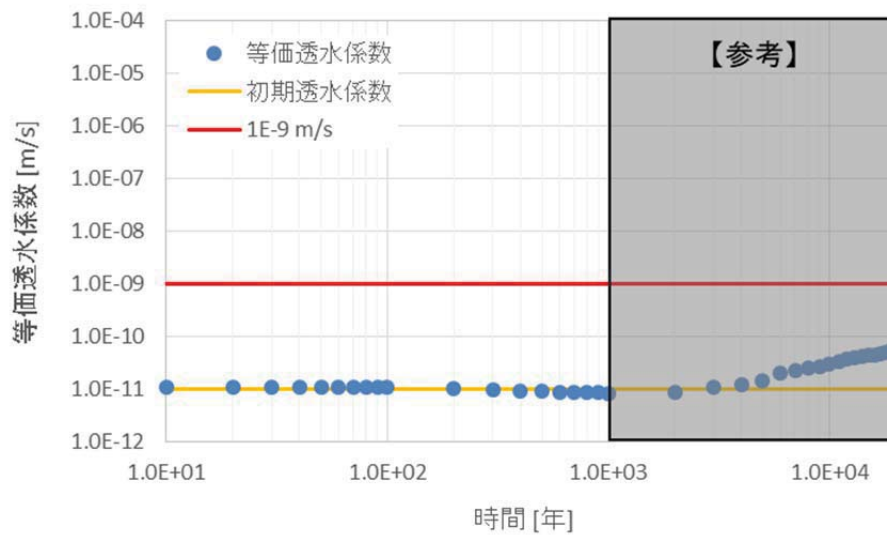
第 1 図 3号廃棄物埋設施設の難透水性覆土(Na型)における等価透水係数の時間変化の結果(ケース①：難透水性覆土の拡散を現実的なモデルとした場合)
