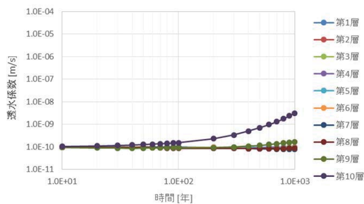
難透水性覆土の透水係数
