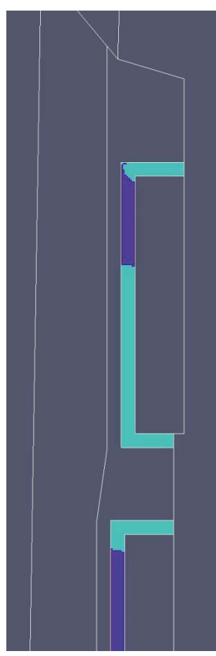
図 難透水性覆土内のペクレ数(P e )分布(6/6)【2号廃棄物埋設地】(厳しい設定 1,000年後)
