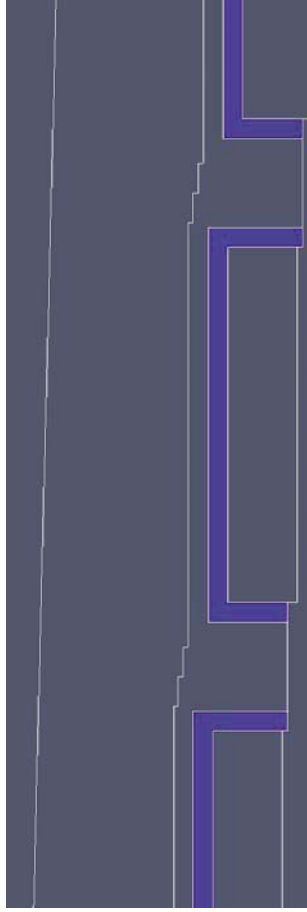
図 難透水性覆土内のペクレ数( P_e )分布(1/6)【3号廃棄物埋設地】(確からしい設定 1,000年後)
