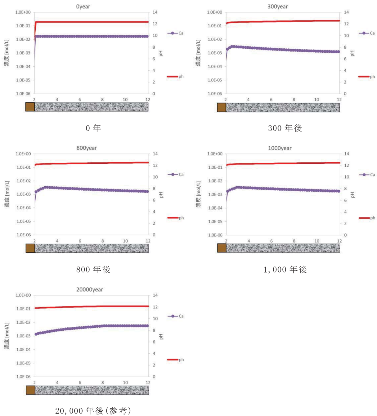
第 9 図 3 号廃棄物埋設施設の埋設設備内の液相組成 (pH、Ca 濃度) の分布図 (ケース①：難透水性覆土の拡散を現実的なモデルとした場合)
