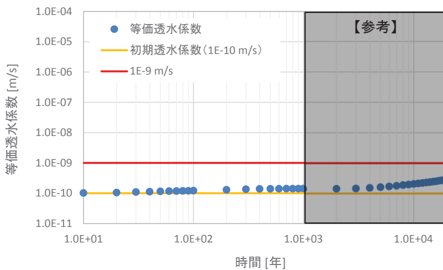
第 6 図 1号廃棄物埋設施設のうち難透水性覆土におけるの等価透水係数の時間変化の結果
