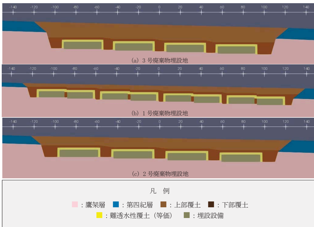
第1図 廃棄物埋設地付近の材料分布(等価透水係数モデル)
