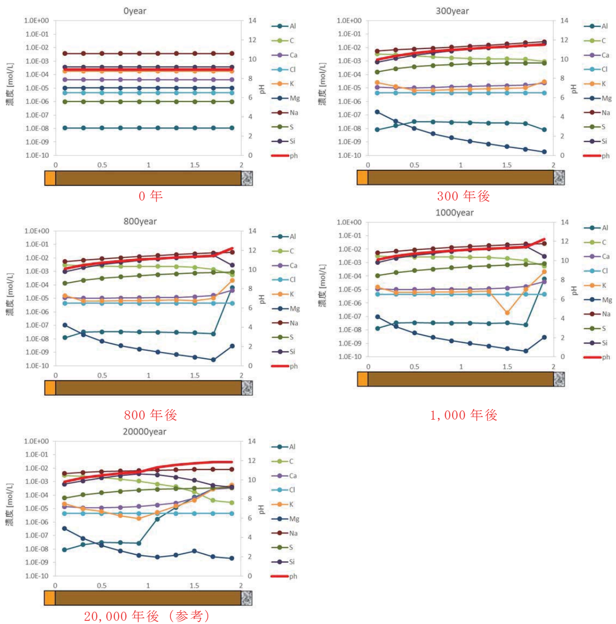
第4図 3号廃棄物埋設施設の難透水性覆土(Na型)内の液相組成の分布図 (ケース①: 難透水性覆土の拡散を現実的なモデルとした場合)
