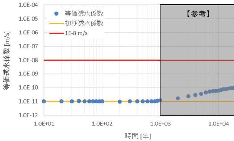
第 9 図 3号廃棄物埋設施設の難透水性覆土(Na型)における等価透水係数の時間変化の結果(ケース②：難透水性覆土の拡散を単純なモデルとした場合)
