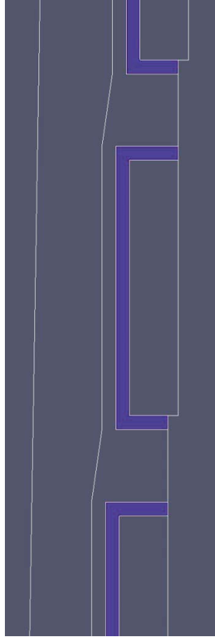
図 難透水性覆土内のペクレ数(P e )分布(5/6)【2号廃棄物埋設地】(確からしい設定 1,000年後)
