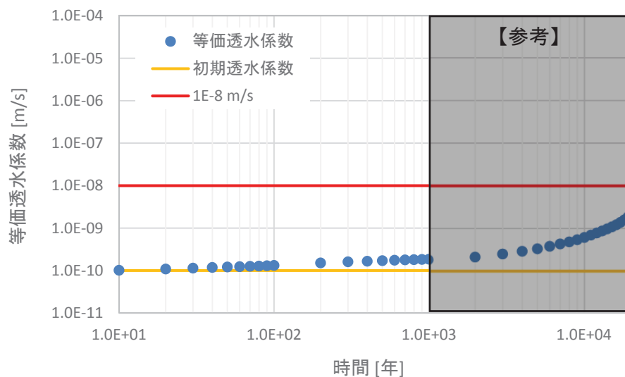
第14図 1号廃棄物埋設施設の うち 難透水性覆土における の 等価透水係数の時間変化の結果
