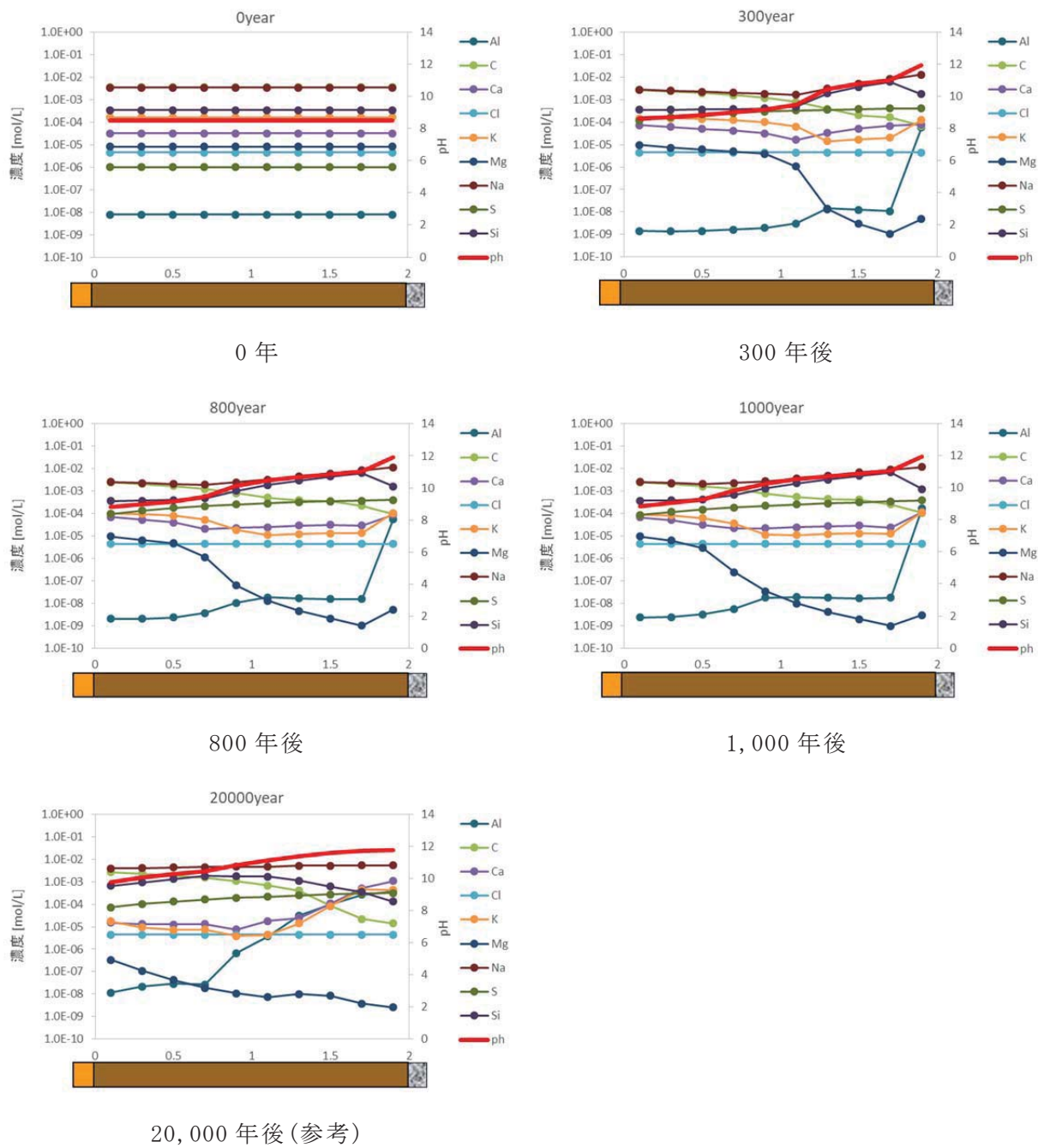
第 8 図 3 号廃棄物埋設施設の うち 難透水性覆土内の液相組成の分布図 (ケース①：難透水性覆土の拡散を現実的なモデルとした場合)
