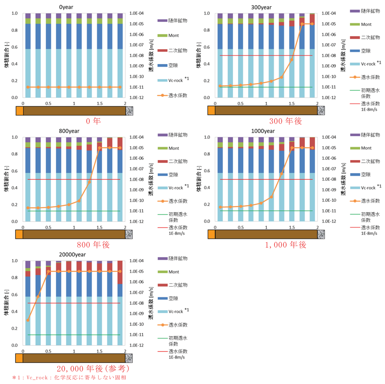
第14図 1号廃棄物埋設施設の難透水性覆土(Na型)における鉱物組成と透水係数の分布図 (ケース②: 難透水性覆土の拡散を単純なモデルとした場合)
