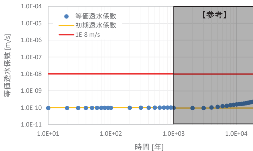
第13図 3号廃棄物埋設施設の うち 難透水性覆土における の 等価透水係数の時間変化の結果
