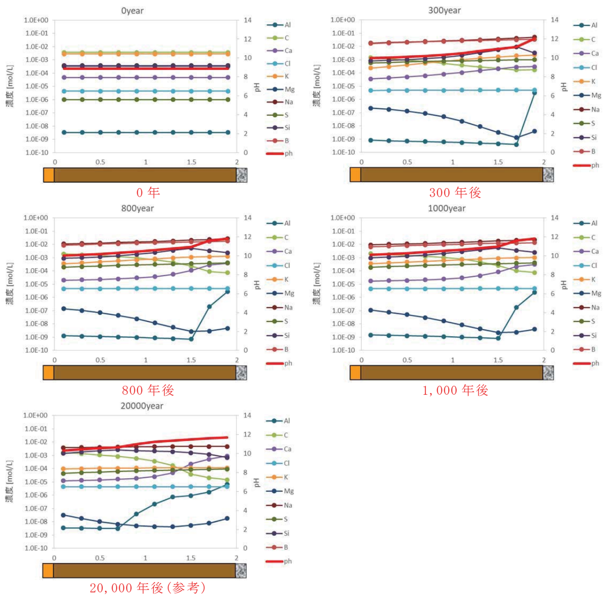
第 15 図 1 号廃棄物埋設施の難透水性覆土 (Na 型) における液相組成の分布図 (ケース②)：難透水性覆土の拡散を単純なモデルとした場合)
