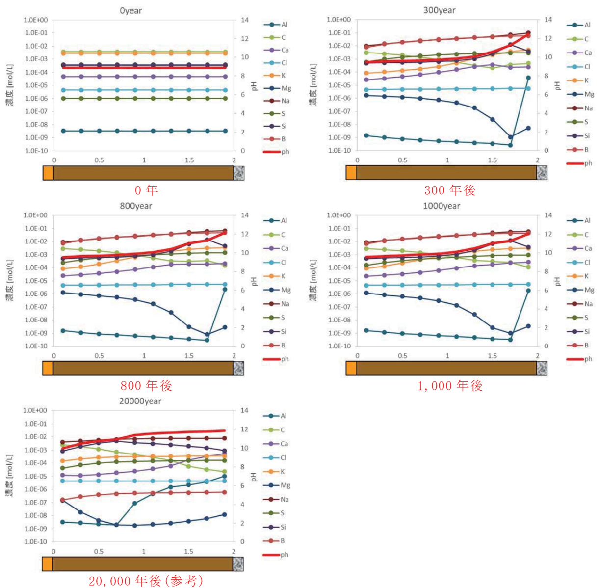
第7図 1号廃棄物埋設施設の難透水性覆土(Na型)内の液相組成の分布図 (ケース①：難透水性覆土の拡散を現実的なモデルとした場合)
