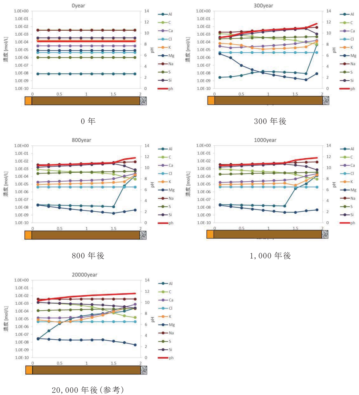
第 16 図 3 号廃棄物埋設施の うち 難透水性覆土における の 液相組成の分布図 (ケース②：難透水性覆土の拡散を単純なモデルとした場合)
