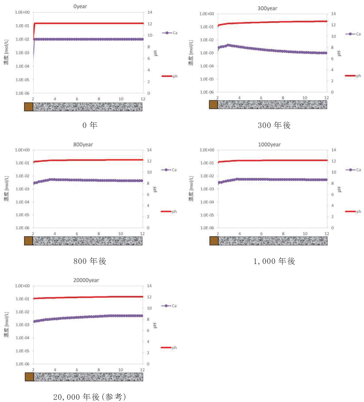
第 20 図 1 号廃棄物埋設施設のうち埋設設備内の液相組成(pH、Ca 濃度)の分布図 (ケース②：難透水性覆土の拡散を単純なモデルとした場合)
