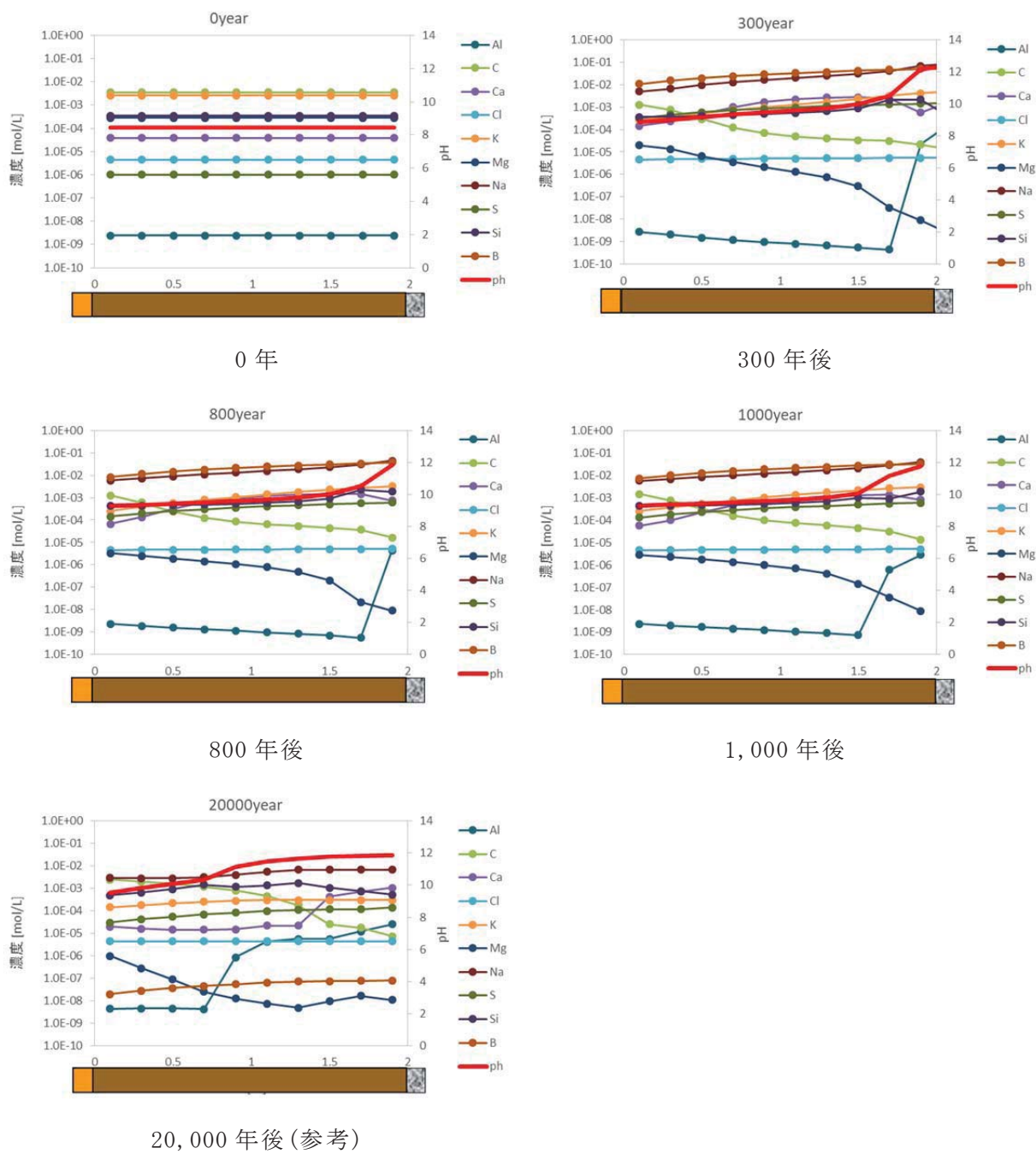
第 11 図 1 号廃棄物埋設施のうち難透水性覆土内の液相組成の分布図 (ケース①：難透水性覆土の拡散を現実的なモデルとした場合)
