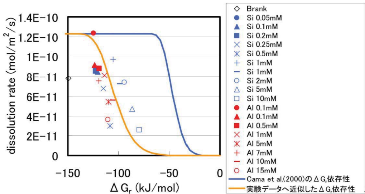
第2図 モンモリロナイトの溶解速度と化学親和力 \Delta G_r との関係(文献 (9) )
