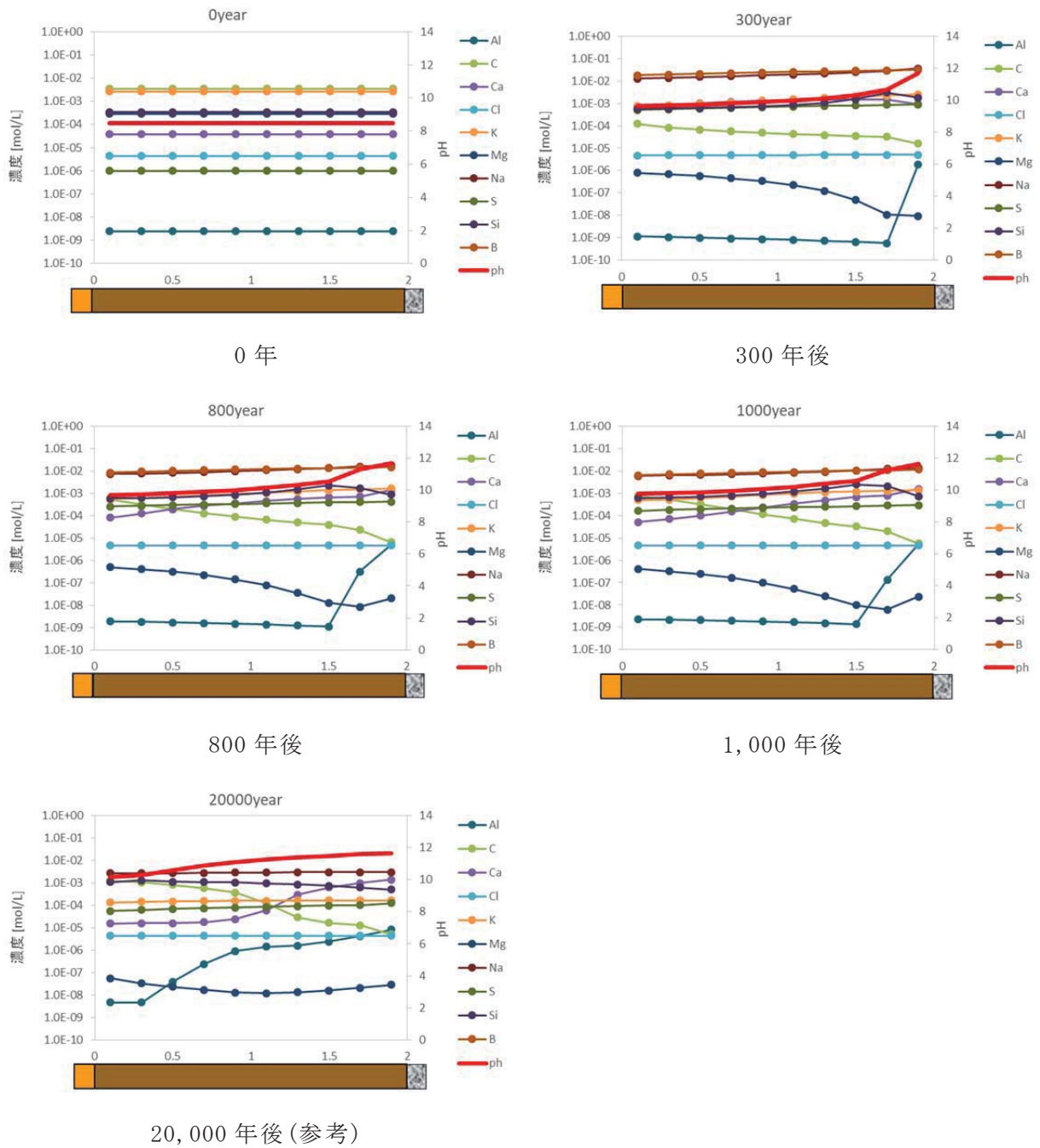
第 19 図 1 号廃棄物埋設施設の うち 難透水性覆土における の 液相組成の分布図 (ケース②：難透水性覆土の拡散を単純なモデルとした場合)
