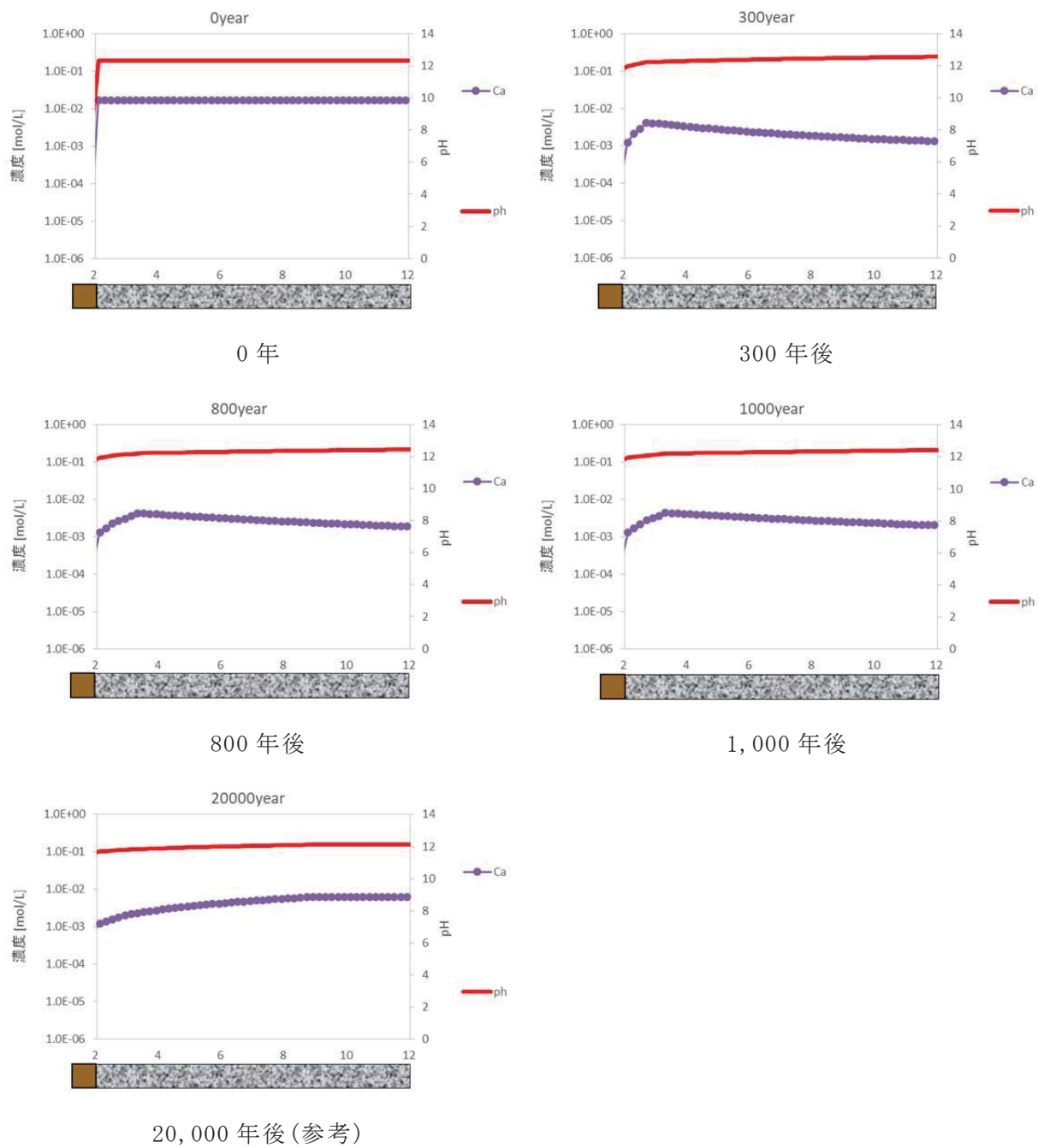
第 17 図 3 号廃棄物埋設施設のうち埋設設備内の液相組成(pH、Ca 濃度)の分布図 (ケース②：難透水性覆土の拡散を単純なモデルとした場合)
