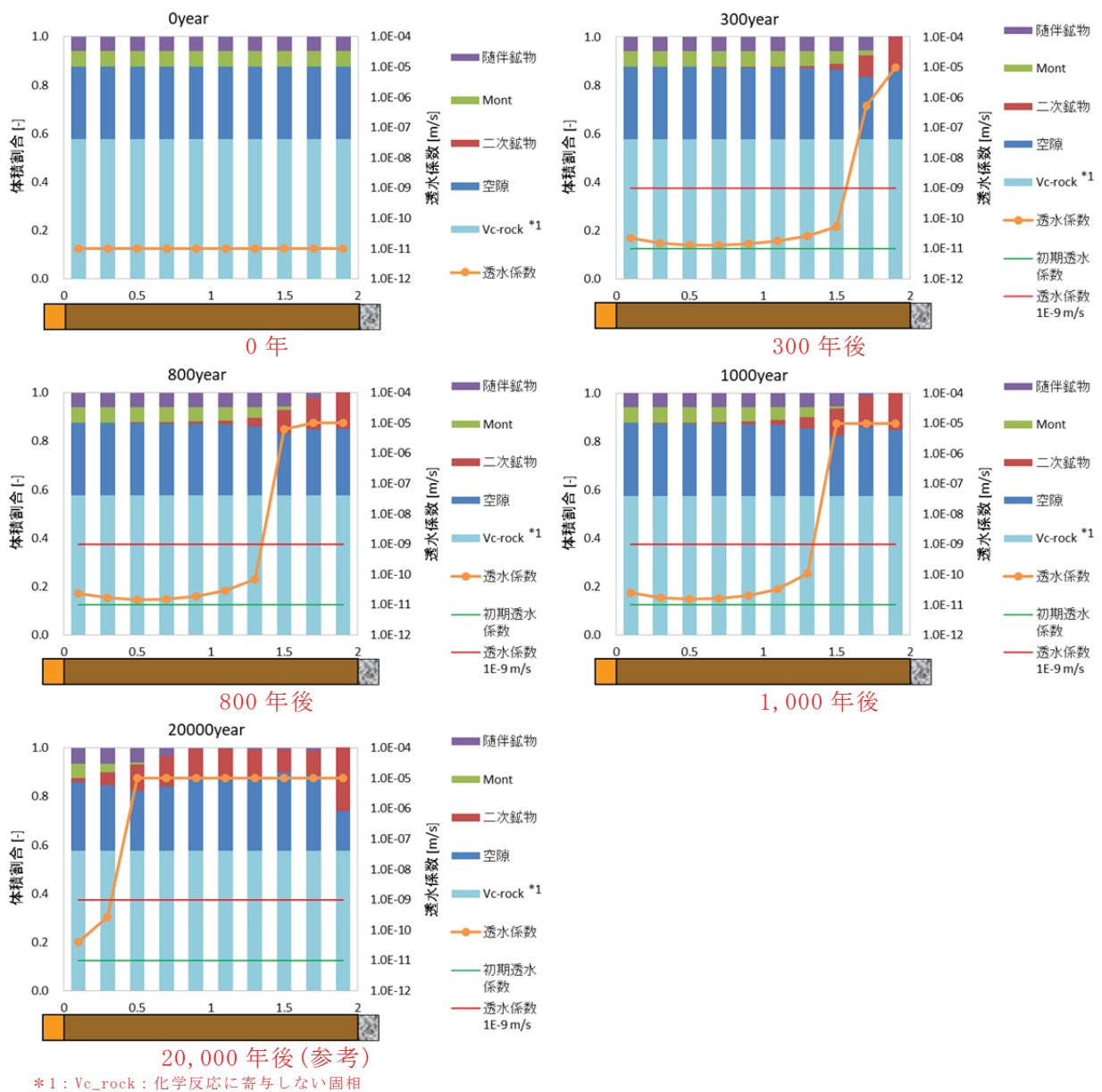
第6図 1号廃棄物埋設施の難透水性覆土(Na型)における鉱物組成と透水係数の分布図 (ケース①: 難透水性覆土の拡散を現実的なモデルとした場合)
