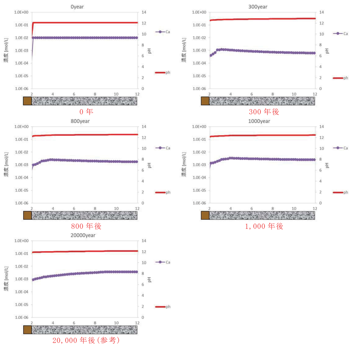
第 8 図 1 号廃棄物埋設施設の埋設設備内の液相組成 (pH、Ca 濃度) の分布図 (ケース①：難透水性覆土の拡散を現実的なモデルとした場合)
