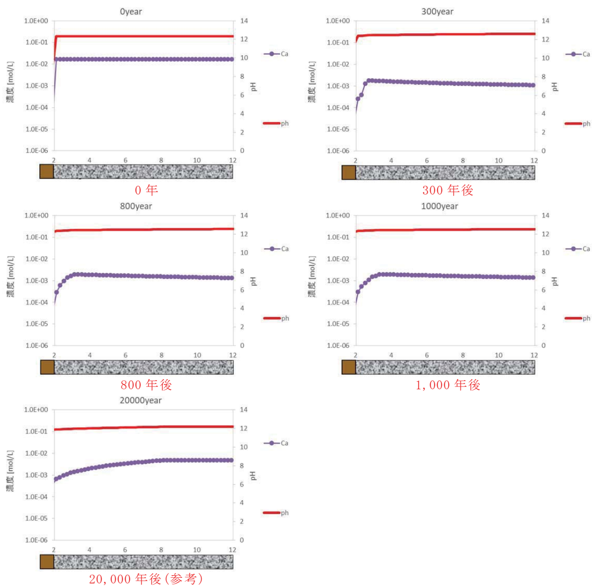
第 5 図 3 号廃棄物埋設施設の埋設設備内の液相組成 (pH、Ca 濃度) の分布図 (ケース①：難透水性覆土の拡散を現実的なモデルとした場合)
